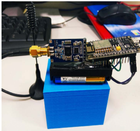
Лабораторный стенд для тестирования WMN
