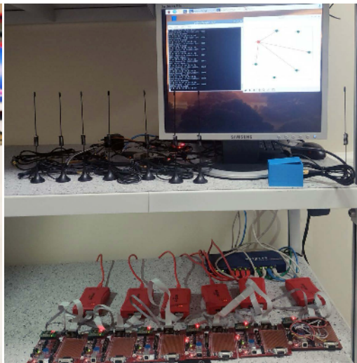
Лабораторный стенд для тестирования WMN
