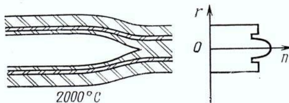
Рис. 5.3. Схлопывание опорной трубки с напыленными слоями двуокиси кремния
