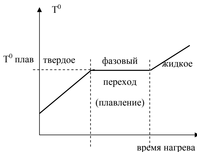
Рис. 1.8, в. Кристаллическая среда
