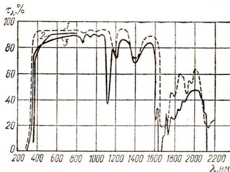
Рис. 4.2. Спектры пропускания оптических полимеров
