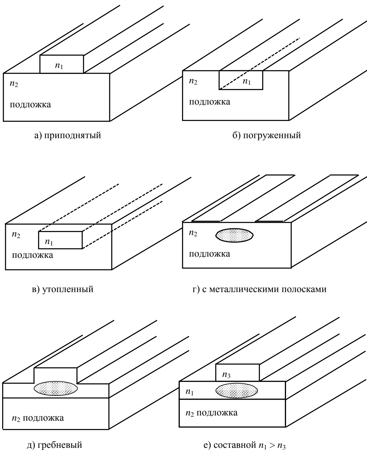
Рис. 5.21. Канальные волноводы различных конструкций.
