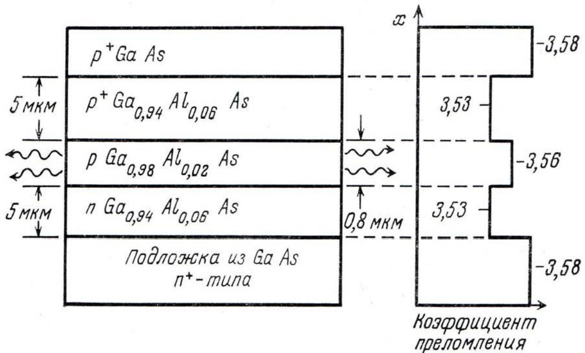
Рис. 5.19. Лазерный диод с двойной гетероструктурой
