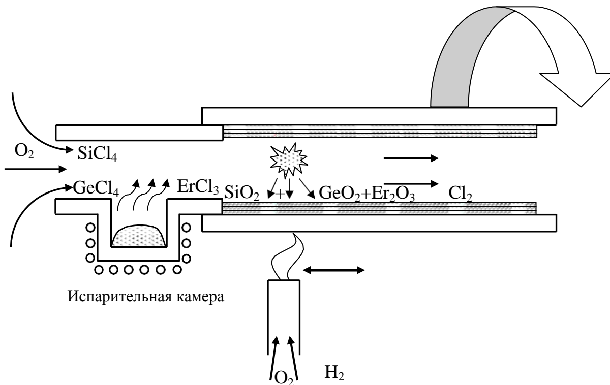
Рис. 5.23. Технология изготовления РЗЭ – легированных ОВ методом MCVD
