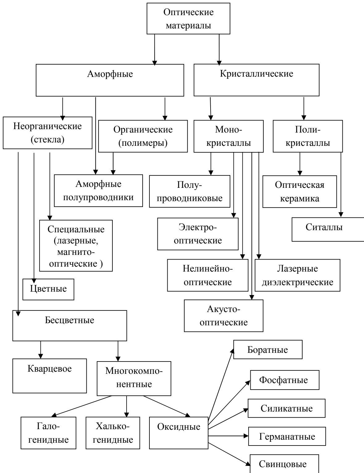
Рис. 1.1. Оптические материалы
