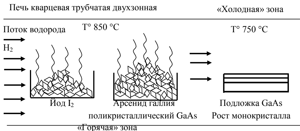
Рис. 3.13. Эпитаксия из газовой фазы
