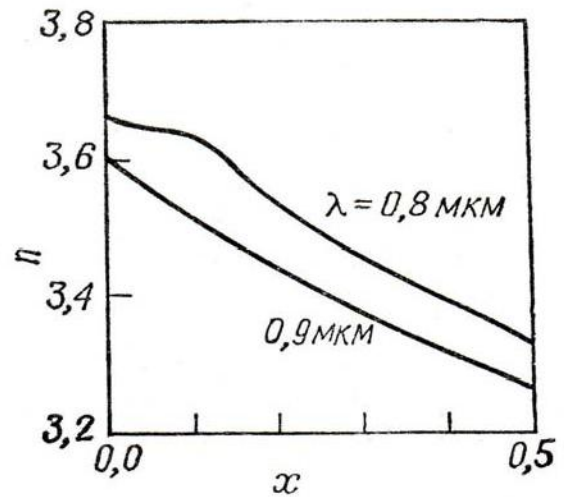
Рис. 5.18. Зависимость показателя преломления материала \text{Ga}_{1-x}\text{Al}_x\text{As} от мольной доли алюминия
