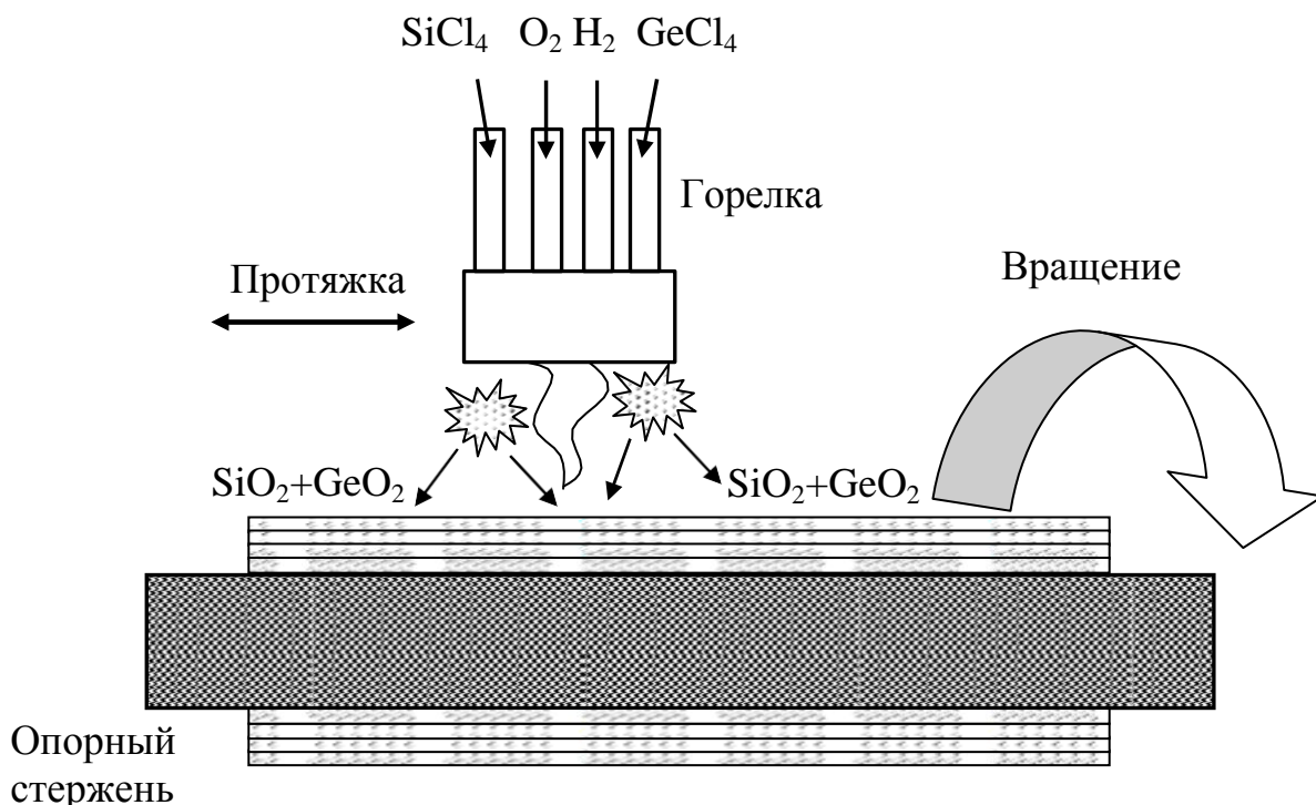
Рис. 5.5. Схема технологического процесса OVD
