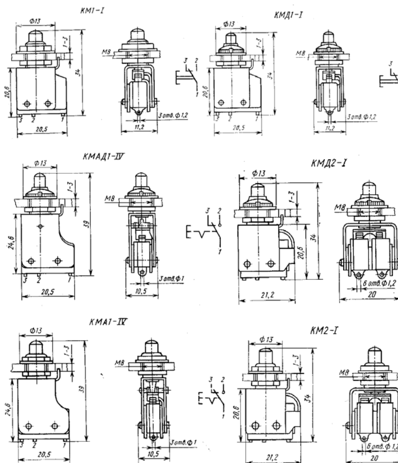
Кнопки командные
