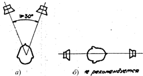
Рис. 5 Размещение слуховых индикаторов
