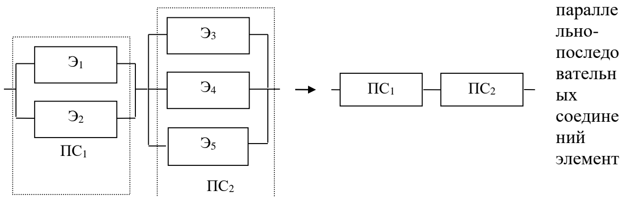
Рис. 12.1. Пример параллельно-последовательного преобразования
