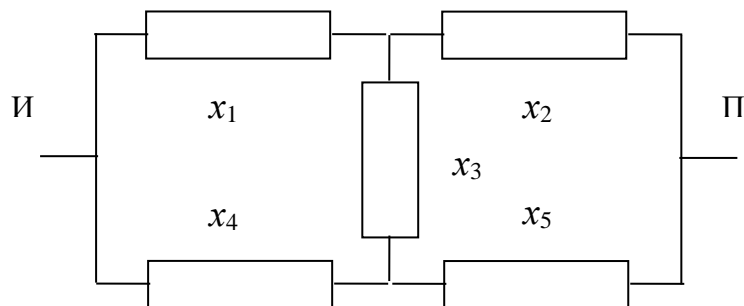
Рис. 6.1. Надежностная схема системы
