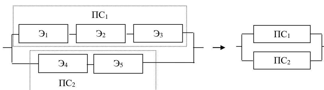
Рис. 6.2. Пример последовательно-параллельного преобразования
