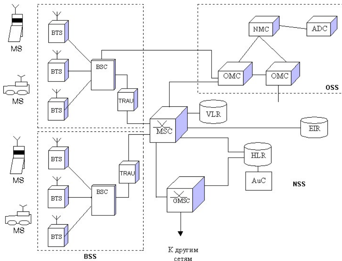
Рис 3.14. Архитектура сети GSM
