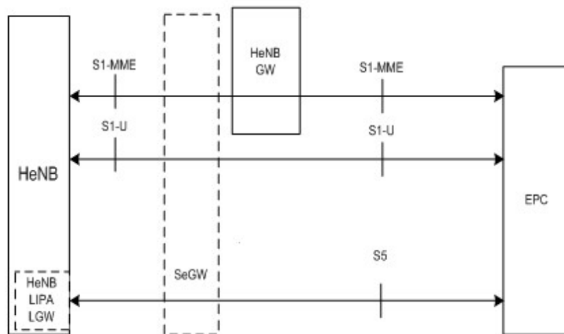
Рис.3.41. Использование LIPA в фемтосети
