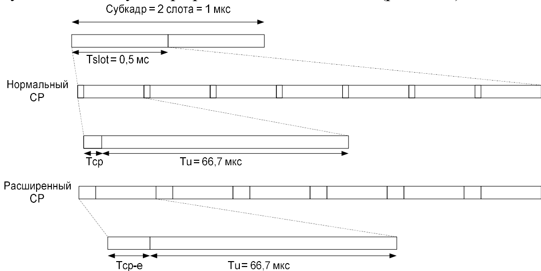
Рис. 3.31. Структура слота на физическом уровне
