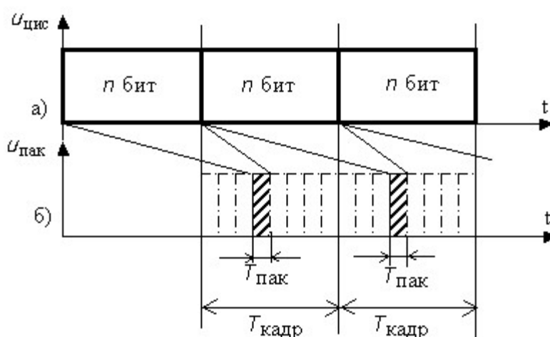
Рис 3.11. Принцип временного уплотнения сигналов
