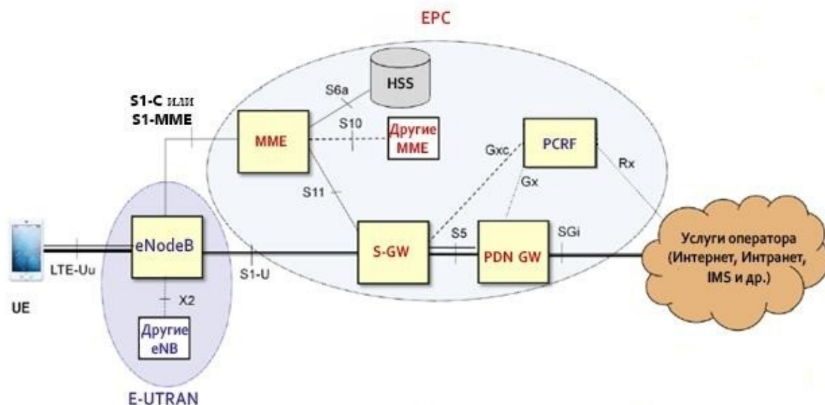
Рис. 3.27. Структура сети LTE
