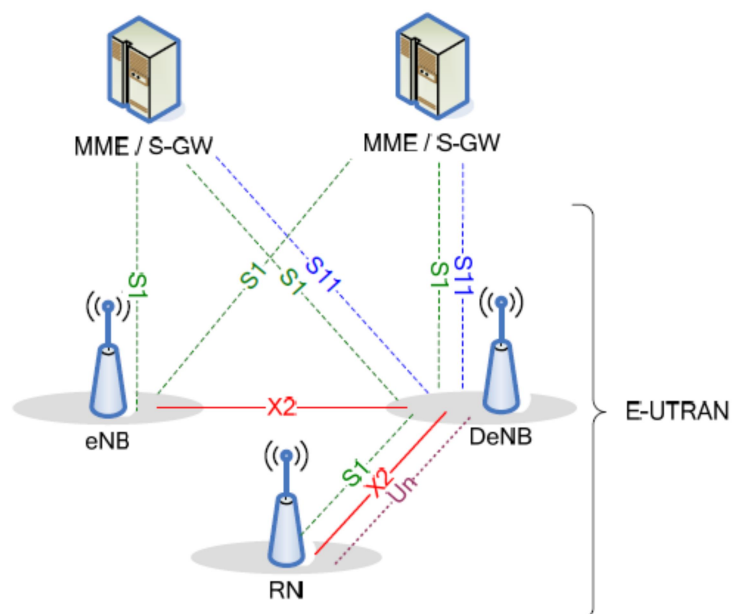
Рис.3.44. Интерфейсы в сетях с релейными станциями
