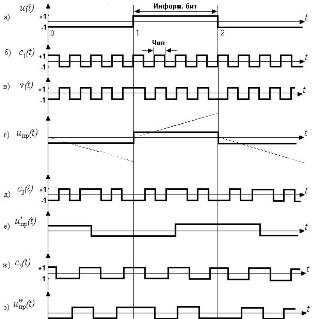
Рис. 3.17. Принцип CDMA
