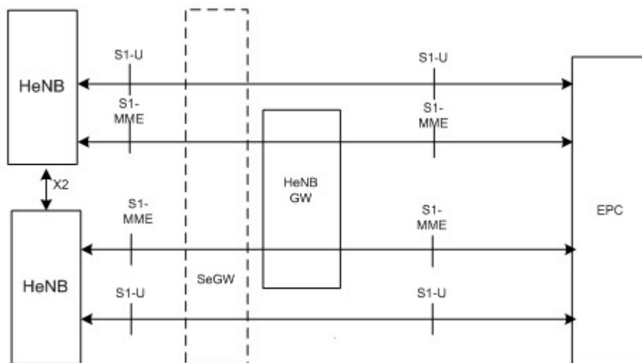
Рис.3.40. Подсоединение HeNB к ядру сети через фемтошлюз
