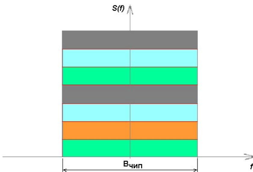
Рис. 3.20. Спектр сигнала на входе приемника BTS
