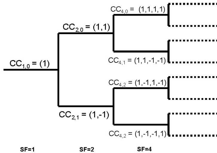
Рис. 3.26. Принцип формирования ортогональных кодов
