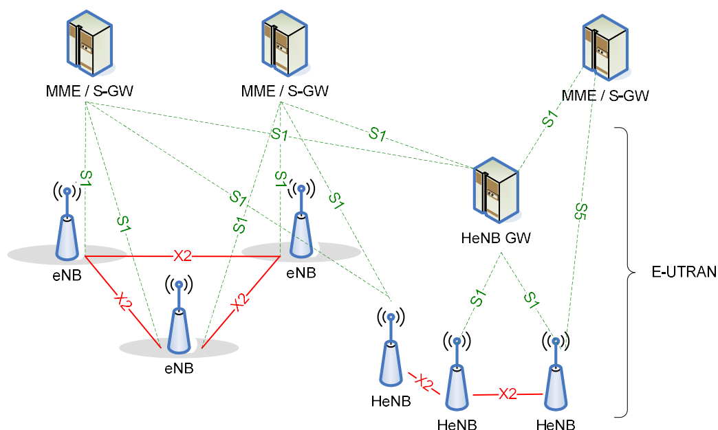
Рис.3.39. Архитектура E-UTRAN с фемтосотами
