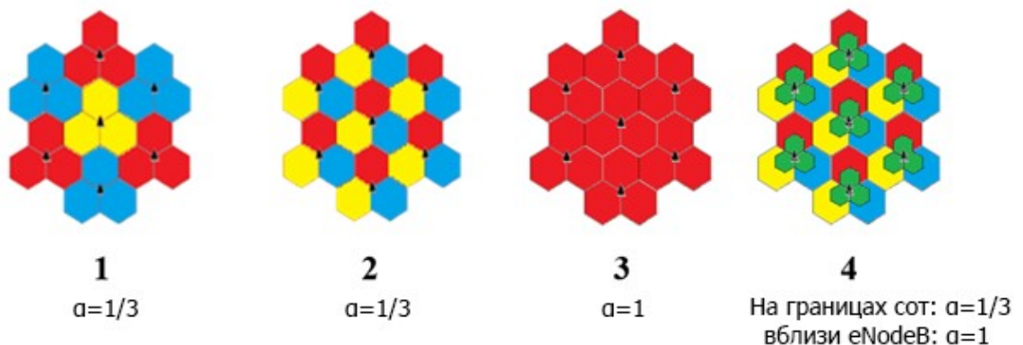
Рис.3.35. Варианты распределения частотного ресурса
