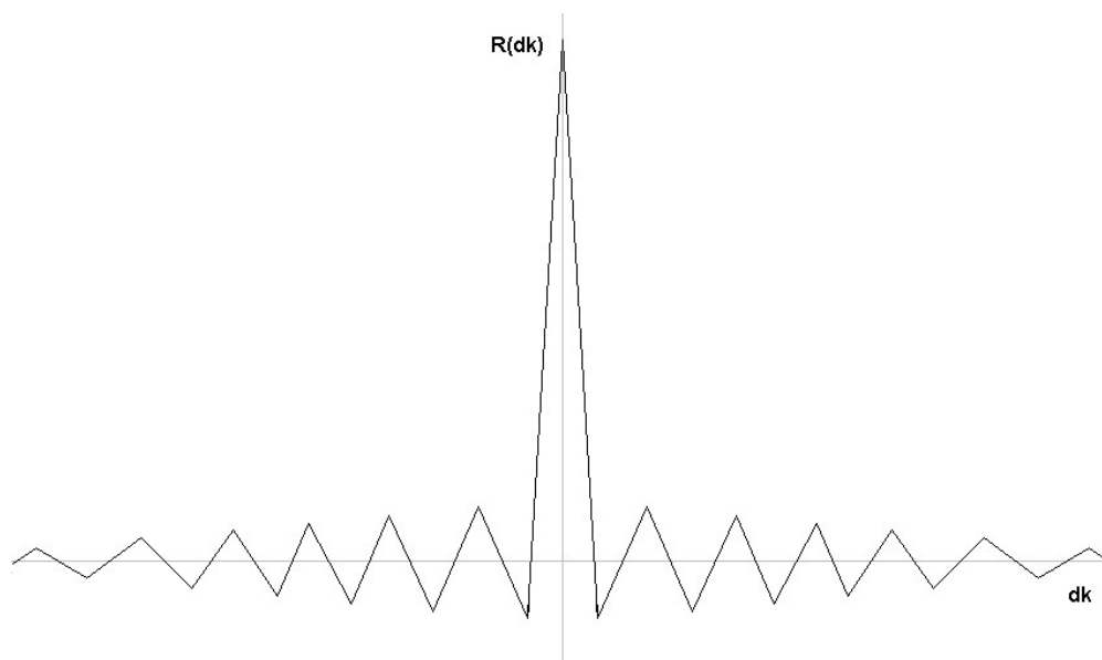
Рис. 3.18. Функция корреляции m -последовательности
