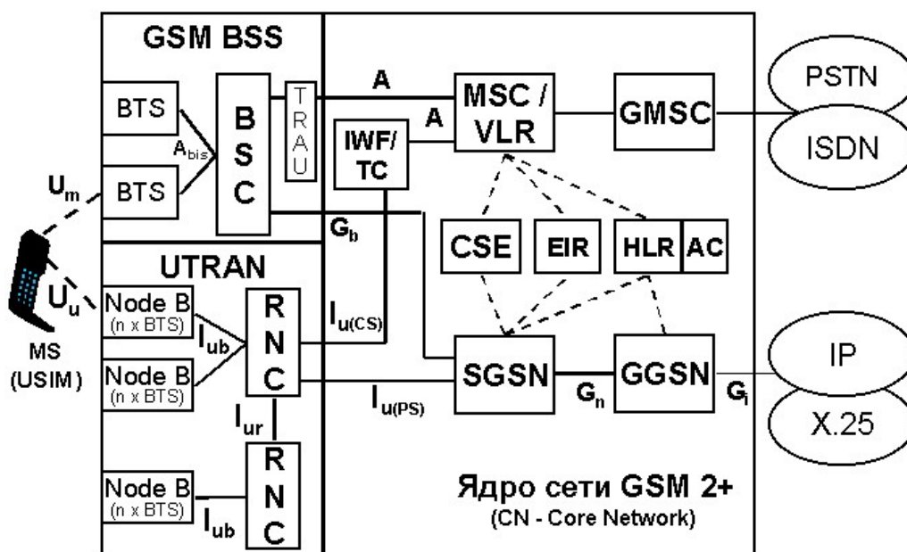
Рис. 3.25. Архитектура интегральной сети UMTS и GSM
