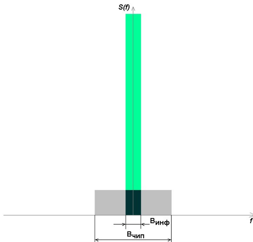
Рис. 3.23. Спектры сигнала и помех на выходе приемника
