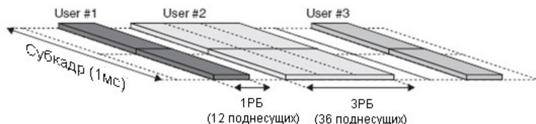
Рис. 3.34. Распределение канального ресурса вверх
