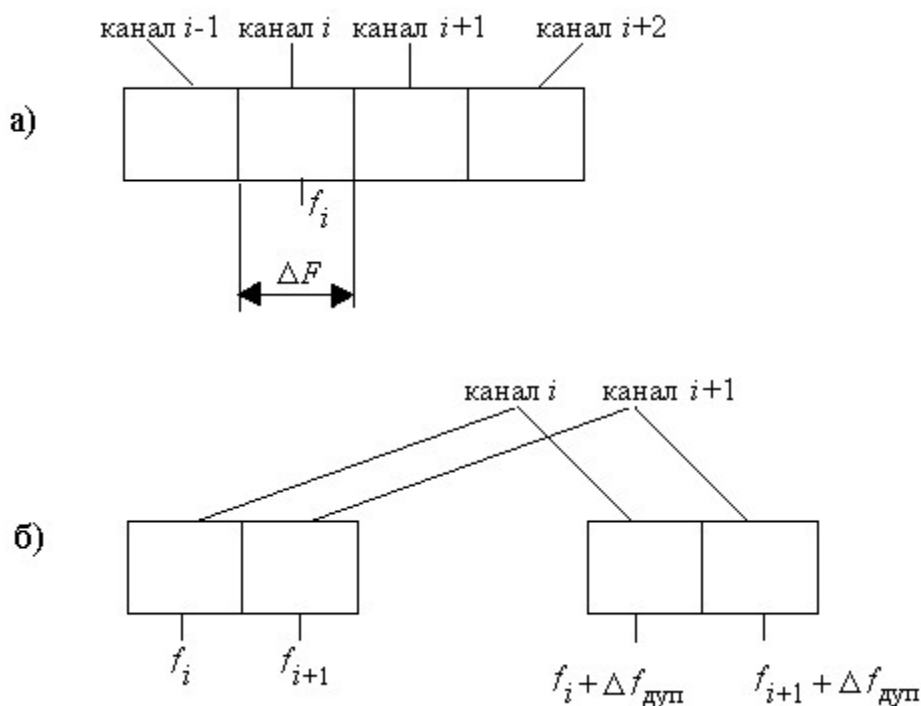
Рис. 3.2. Полосы частот для симплексного (а) и дуплексного (б) каналов
