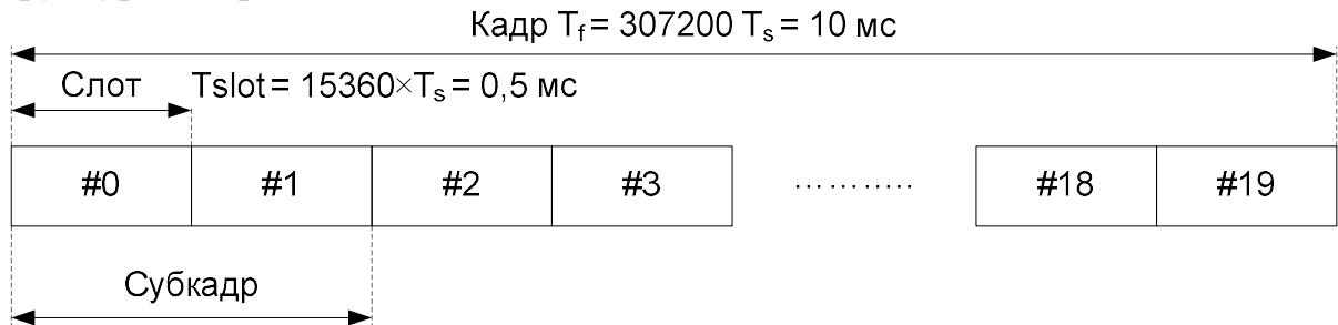
Рис.3.28. Структура кадра LTE
