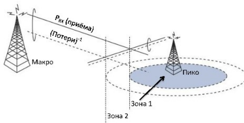
Рис.3.38. Неоднородная структура с макро и пикосотами
