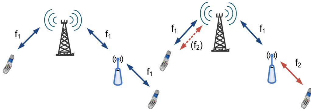
Рис.3.43. LTE-A. In-band (слева) и out-of-band (справа)
