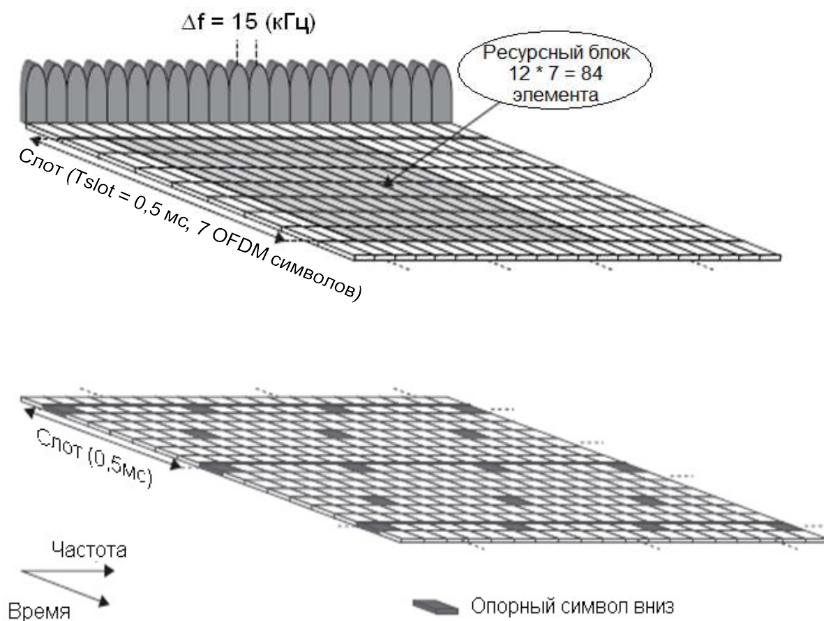
Рис. 3.32. Структура ресурсного блока при передаче вниз
