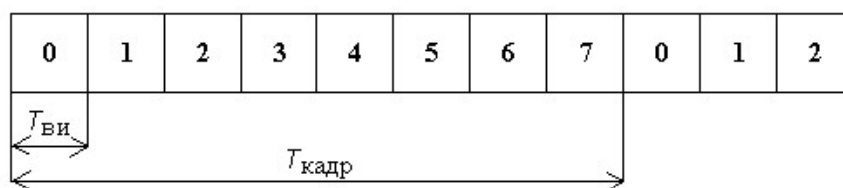
Рис 3.12. Кадр, состоящий из 8 временных интервалов
