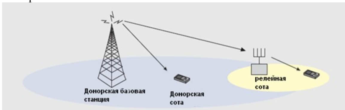
Рис. 3.42 Структура сети с релейной станцией
