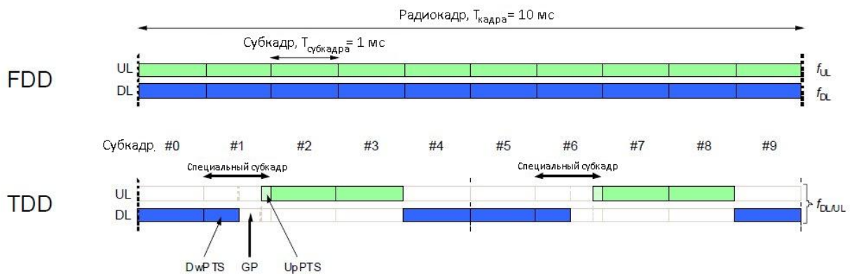
Рис.3.29. Конфигурация кадра при частотном и временном дуплексе
