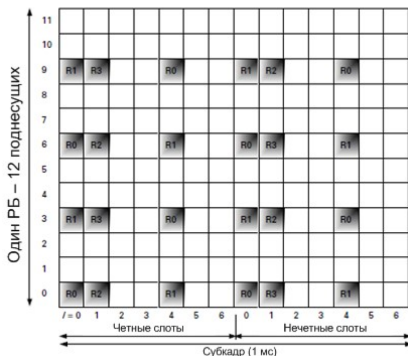
Рис.3.33. Позиционирование символов CRS в ресурсном блоке при передаче Вниз
