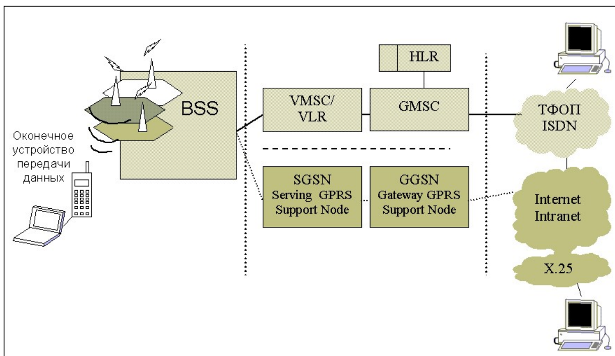
Рис. 3.16. Укрупненная структура сети GSM с поддержкой GPRS
