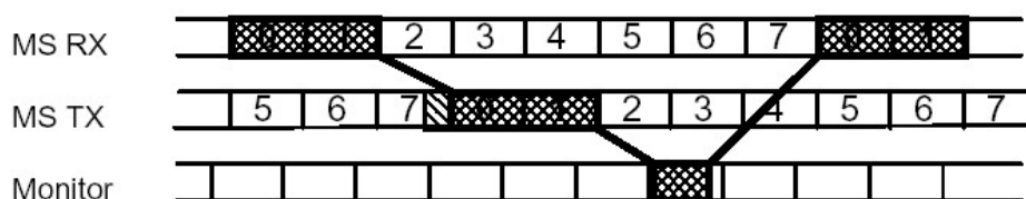
Рис. 3.15. Задачи приема и передачи сигналов MS при HSCSD
