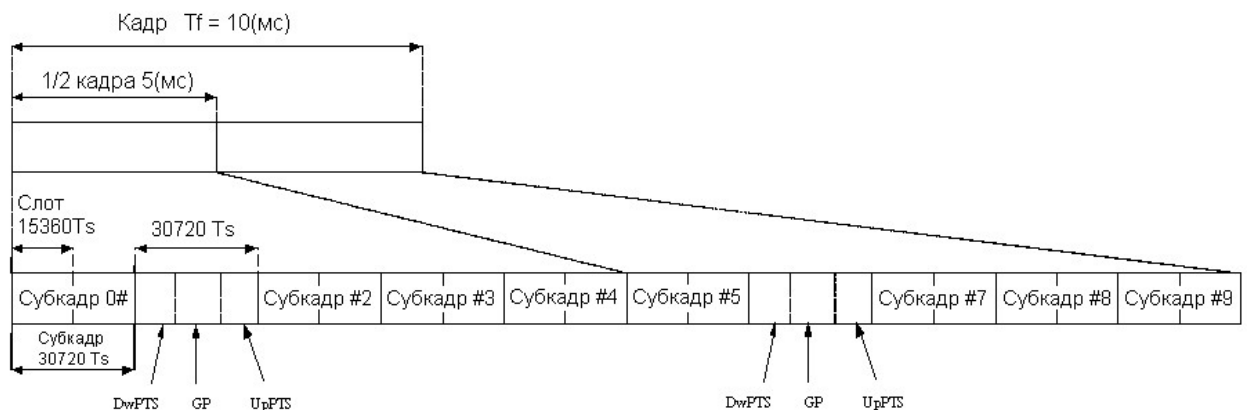
Рис. 3.30. Конфигурации кадра при временном дуплексе
