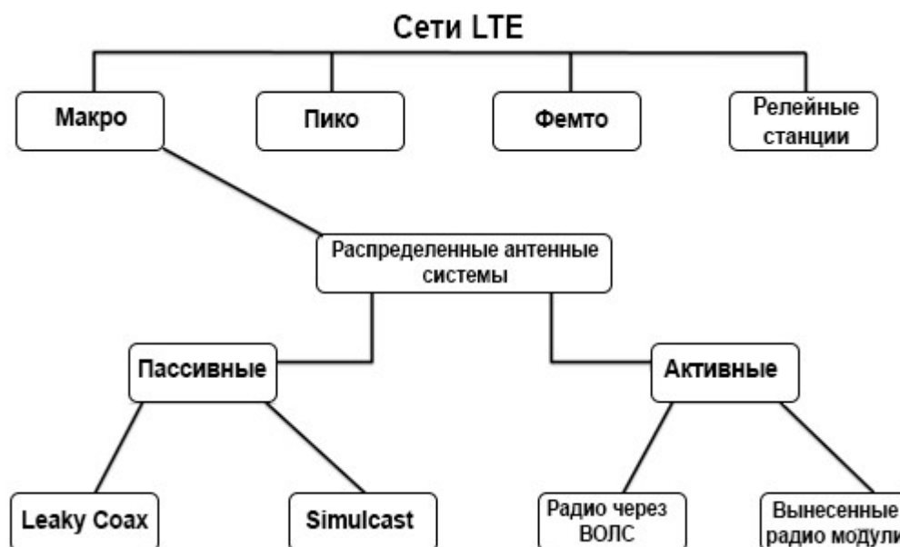
Рис. 3.37. Варианты неоднородных структур сетей LTE
