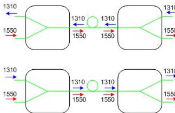
Рис.14. Работа WDM-сплиттеров при спектральном уплотнении каналов в одном направлении и во встречных направлениях.
