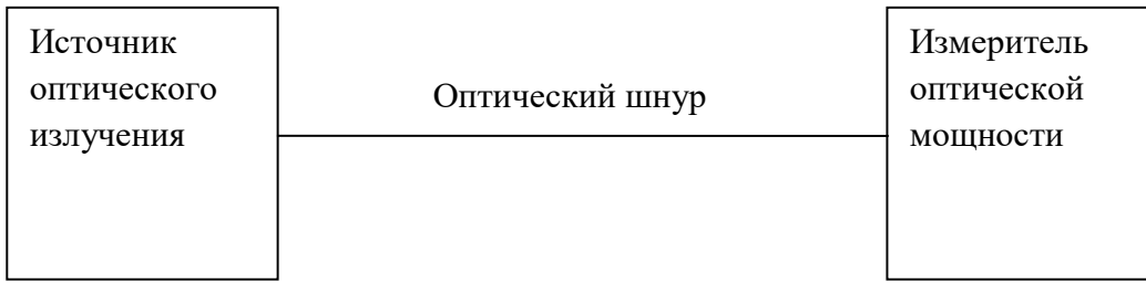
Рис.8. Подготовка измерительных приборов к проведению измерений. Измерение уровня мощности, вводимой во входной порт оптического разветвителя.
