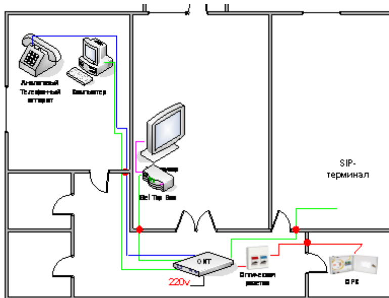
Рис.П.3.12. Схема предоставления услуг в помещении абонента.
