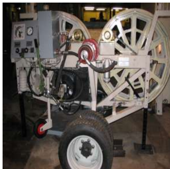
Рис.9.13. Натяжная и тормозная машина для самонесущего ВОК.
