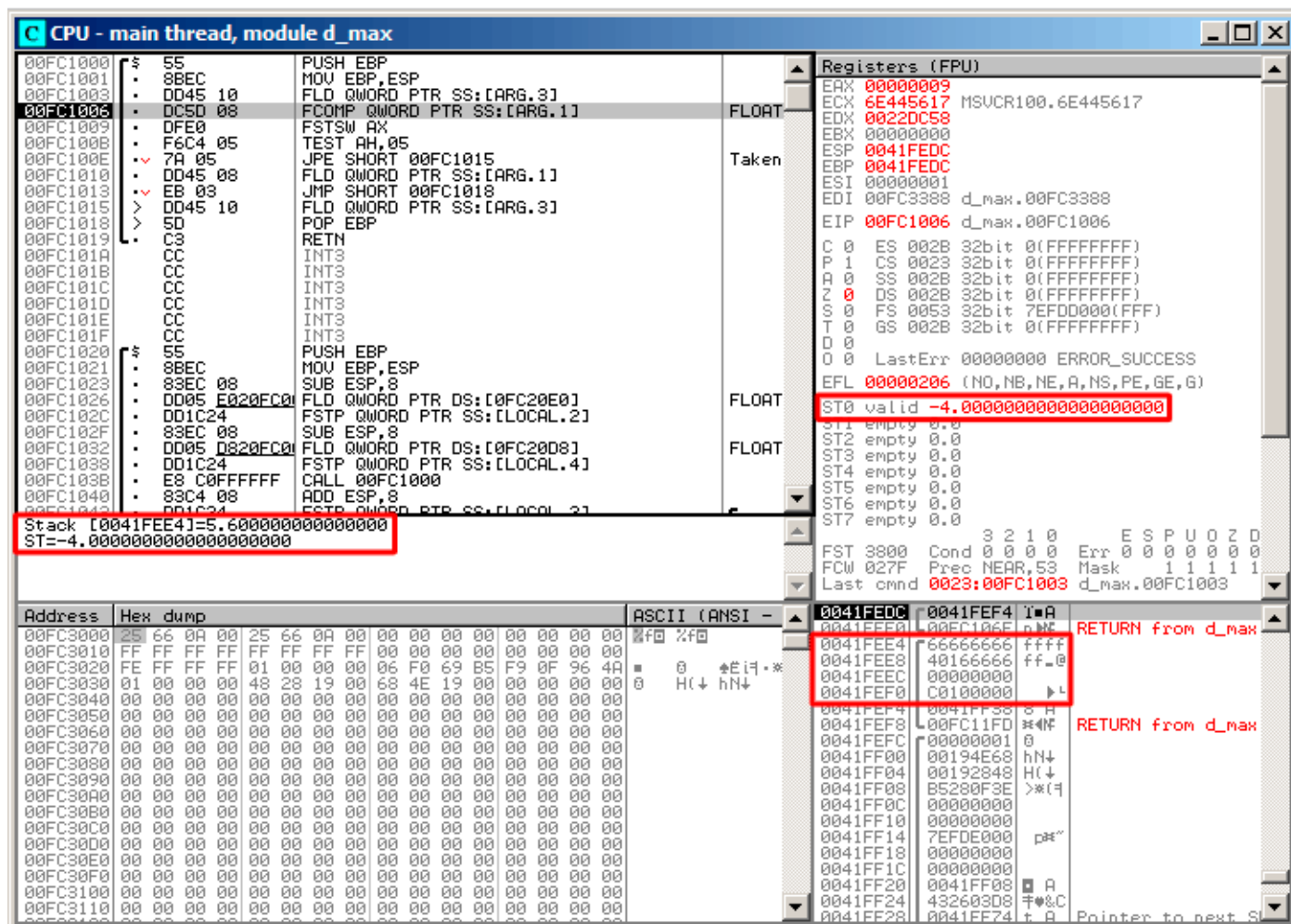
Рис. 1.64: OllyDbg: первая FLD исполнилась
