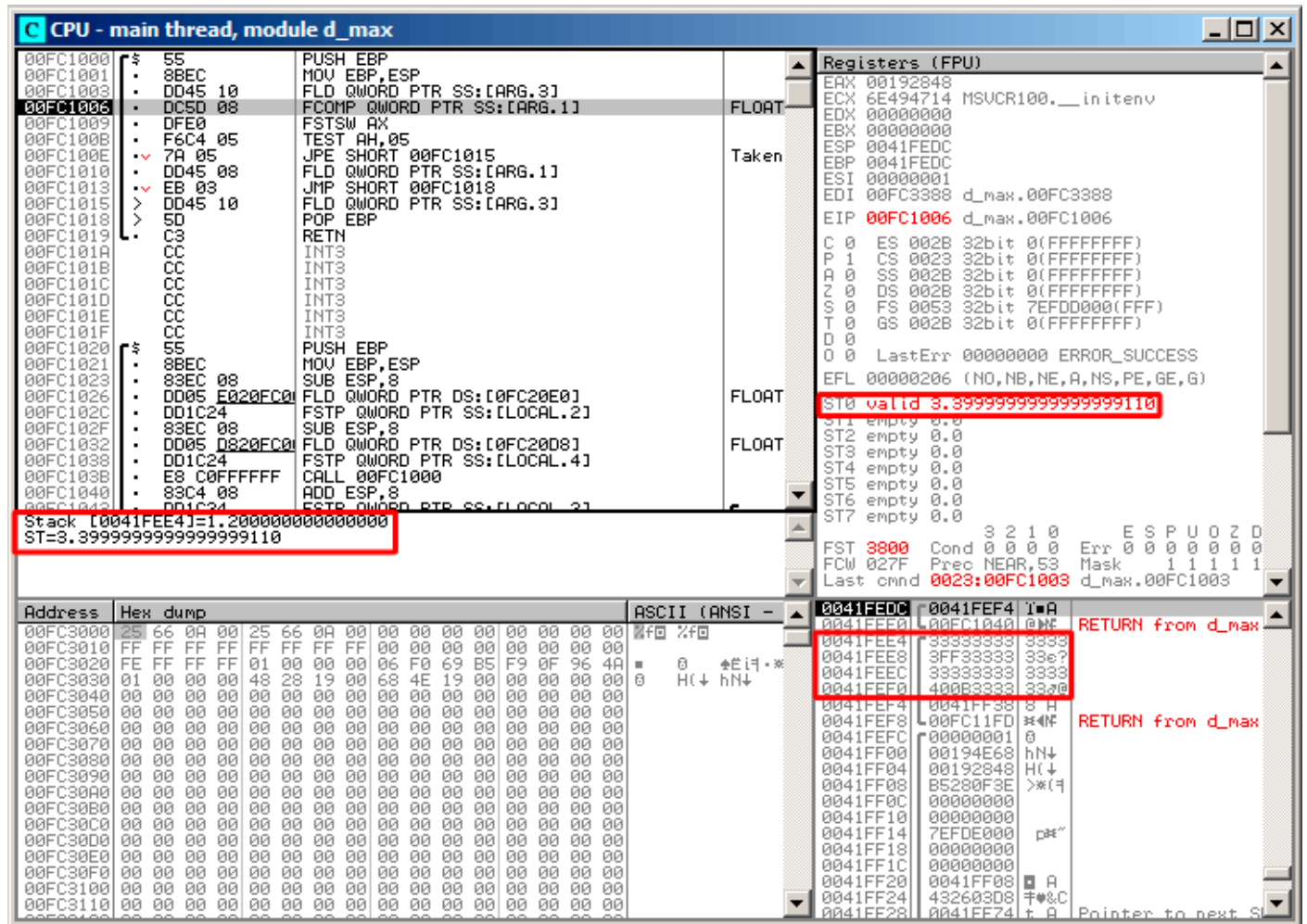
Рис. 1.59: OllyDbg: первая FLD исполнена
