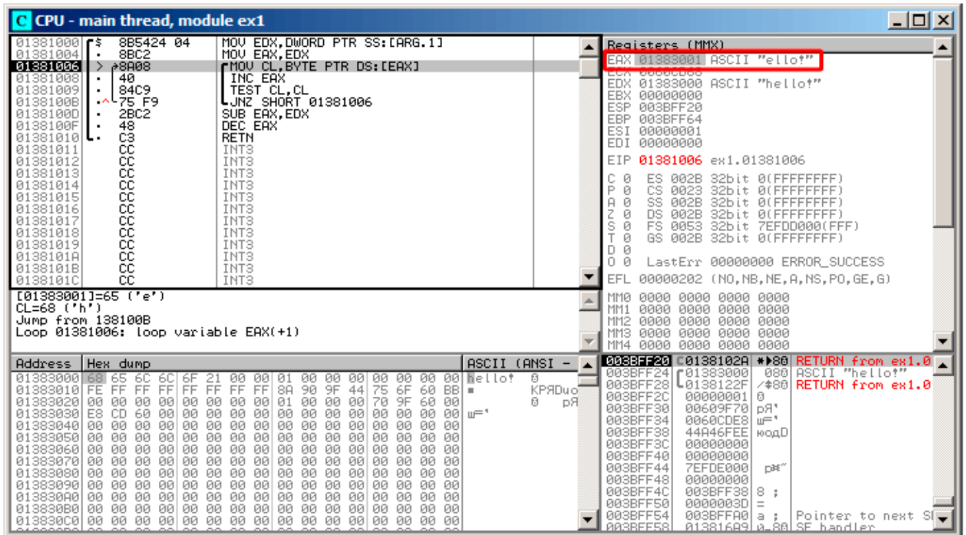
Рис. 1.51: OllyDbg: начало второй итерации
