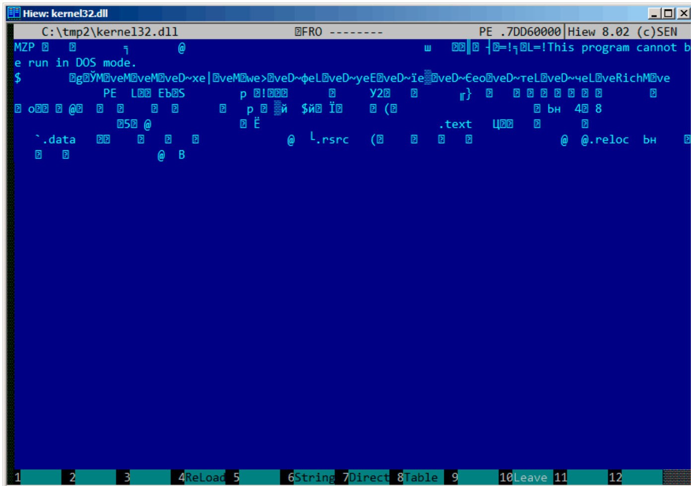
Рис. 9.3: Оригинальный файл
