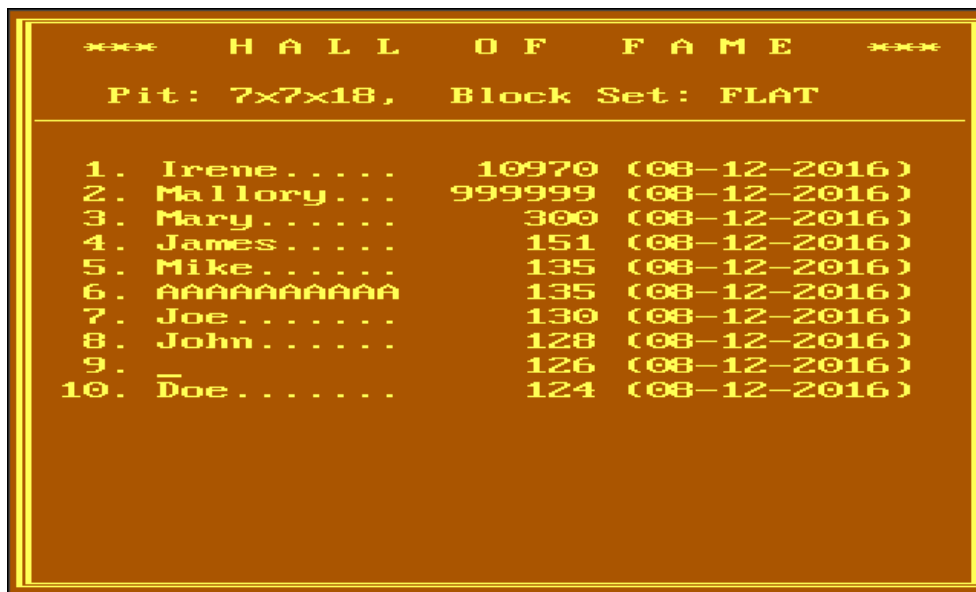
Рис. 3.7: Таблица рекордов
