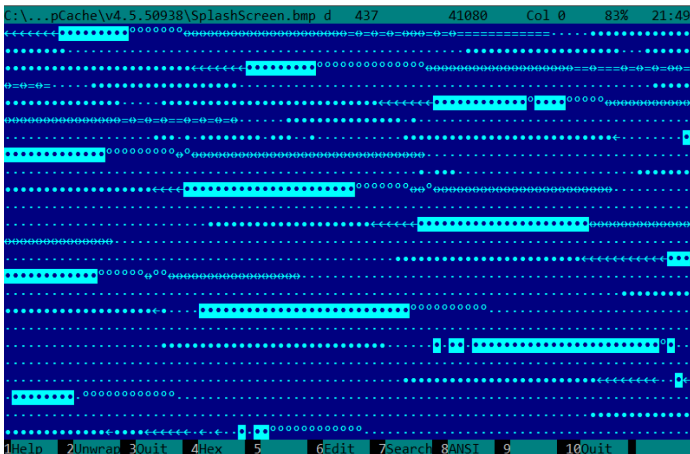
Рис. 5.15: Фрагмент BMP-файла
