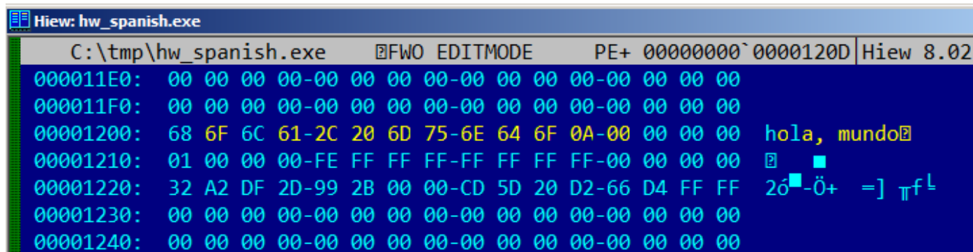
Рис. 1.2: Hiew
