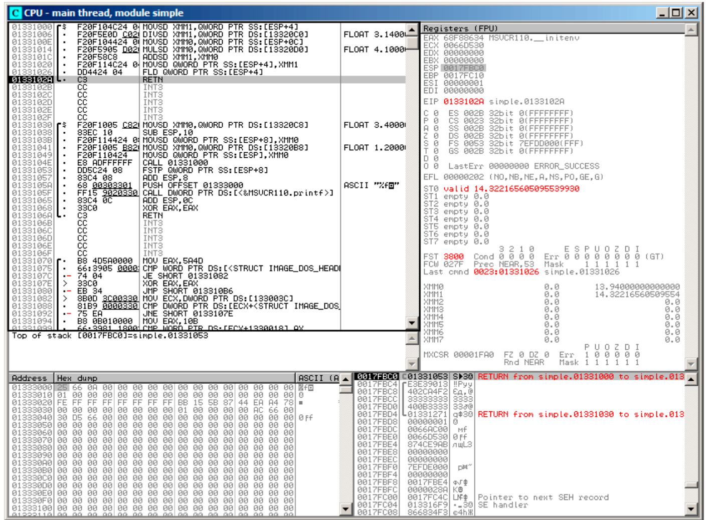
Рис. 1.109: OllyDbg: FLD оставляет результат функции в ST(0)
