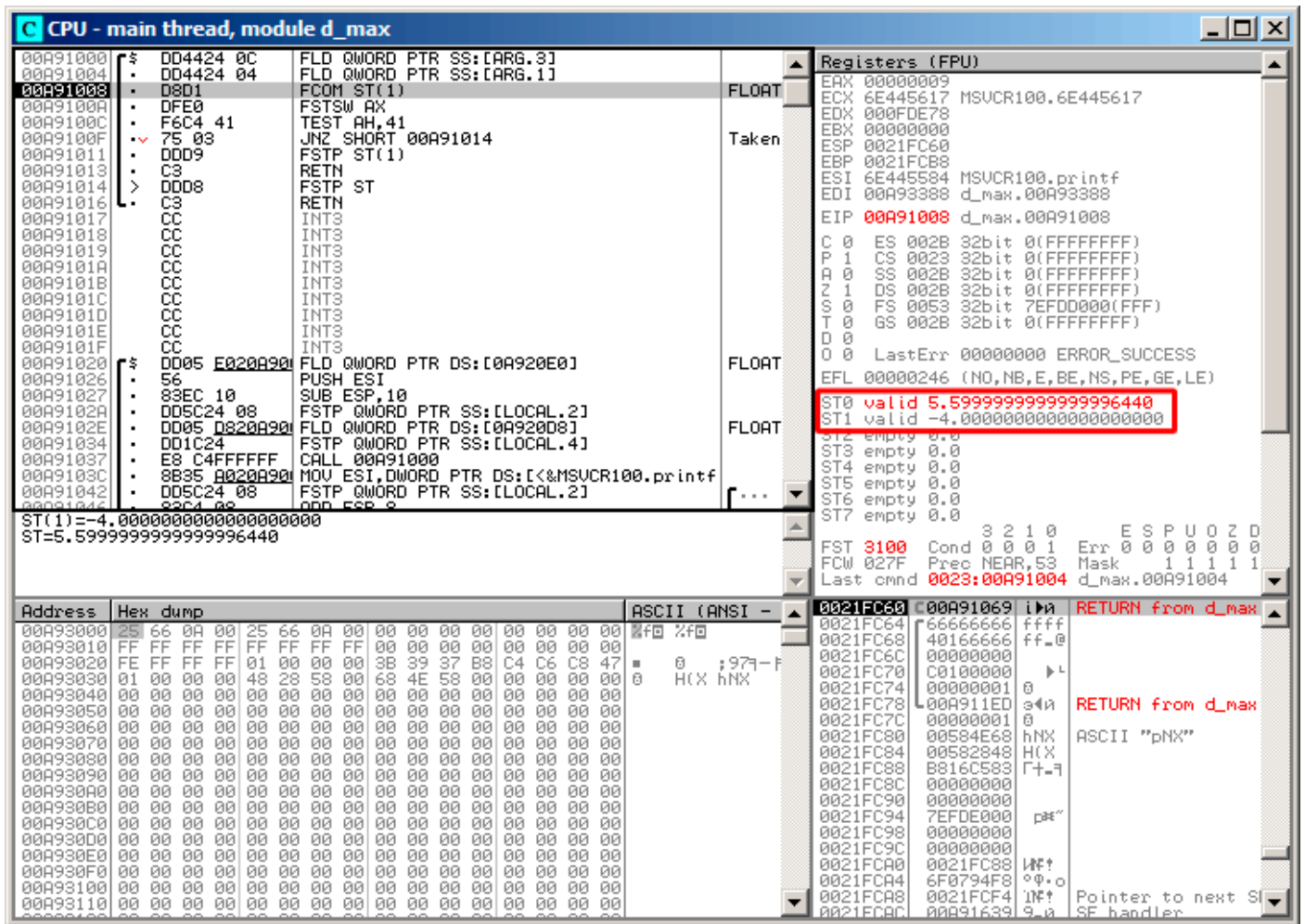
Рис. 1.74: OllyDbg: обе FLD исполнились
