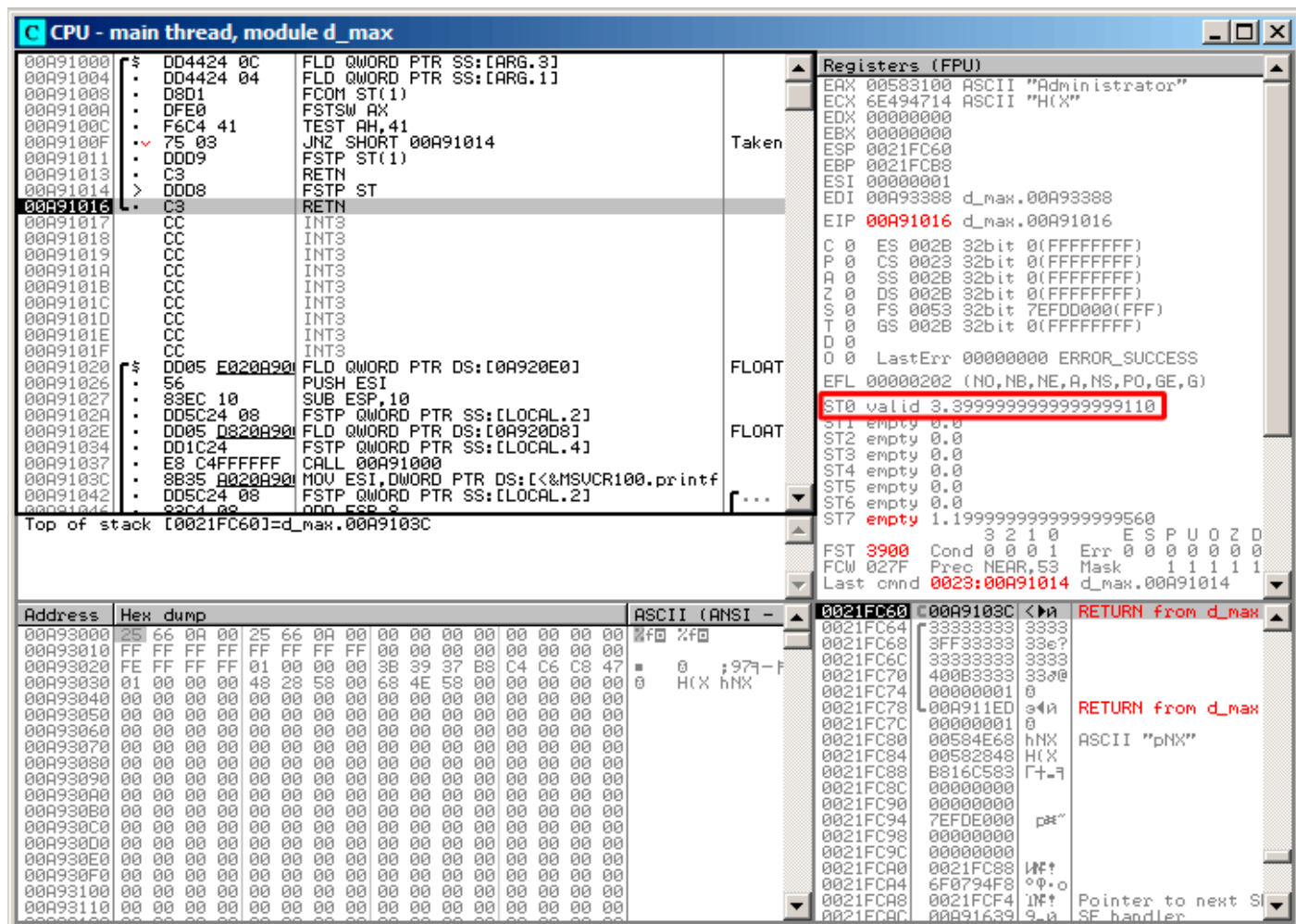
Рис. 1.73: OlyDbg: FSTP исполняется
