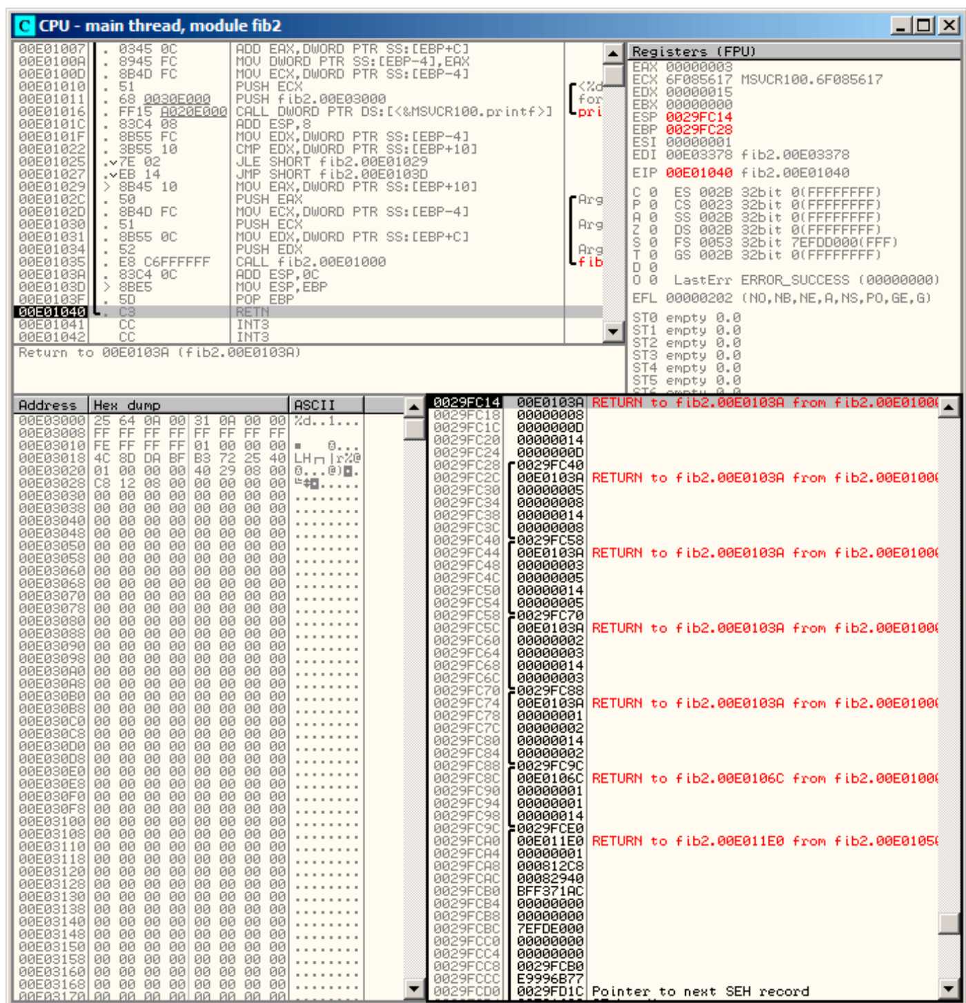
Рис. 3.2: OllyDbg: последний вызов f()
