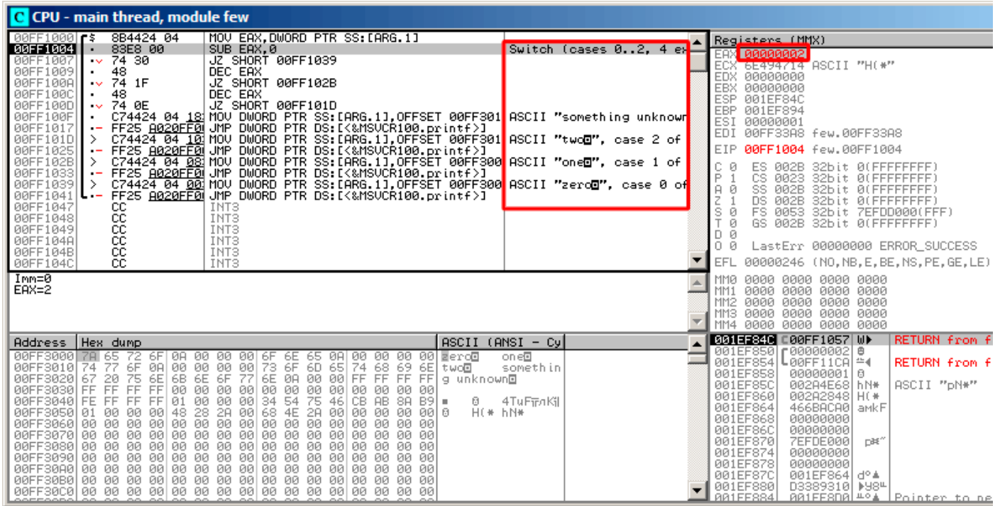
Рис. 1.34: OllyDbg: EAX содержит первый (и единственный) аргумент функции
