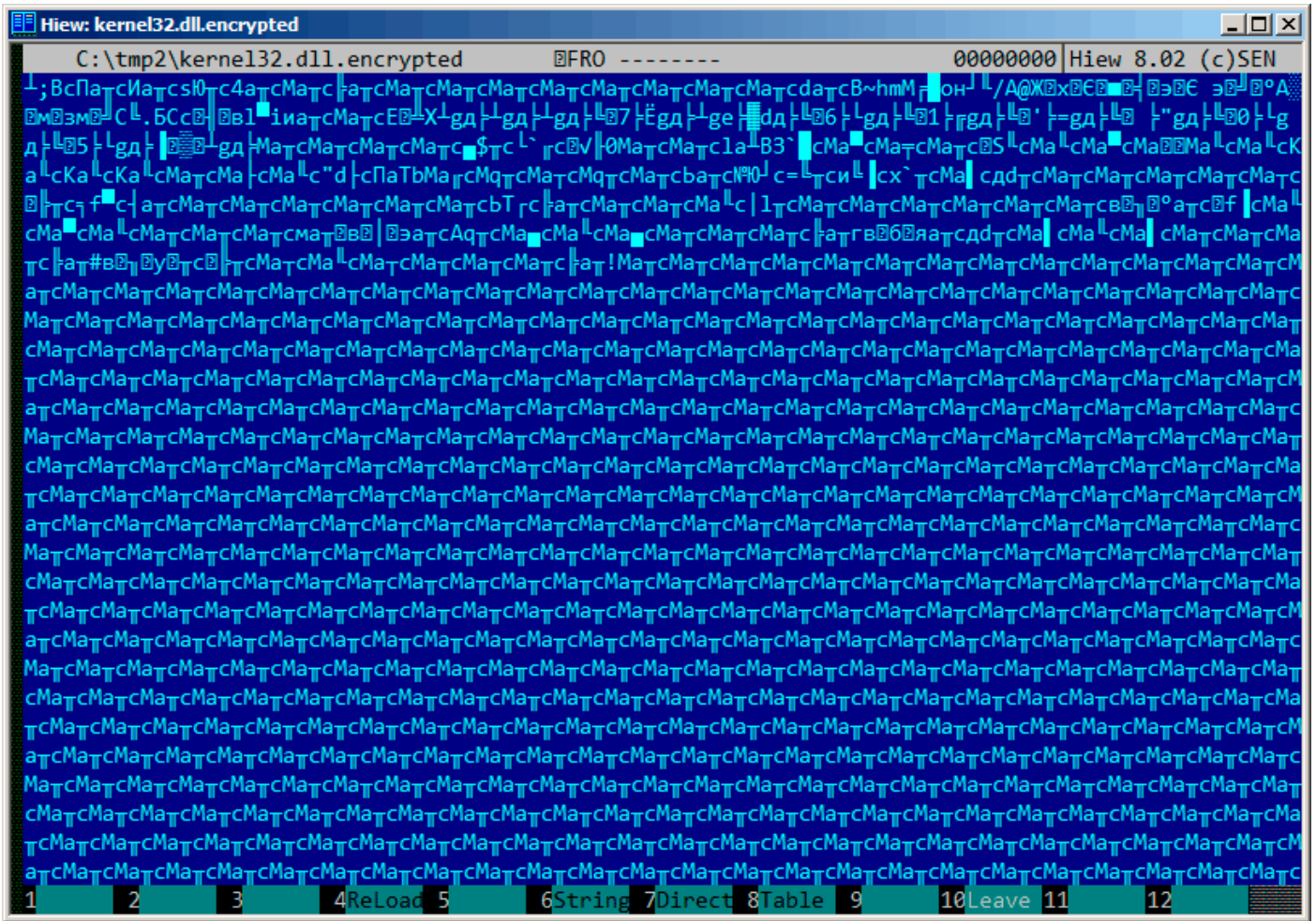
Рис. 9.4: «Зашифрованный» файл
