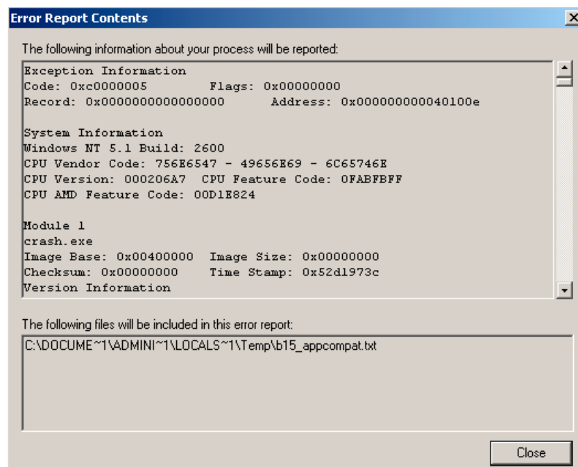
Рис. 6.3: Windows XP
