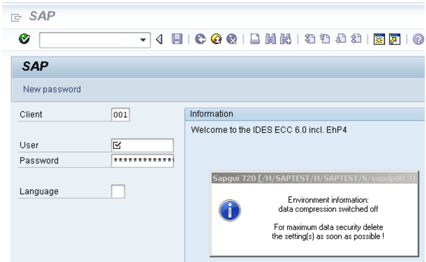
Рис. 8.15: Скриншот
