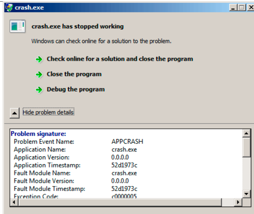
Рис. 6.4: Windows 7
