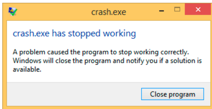
Рис. 6.5: Windows 8.1
