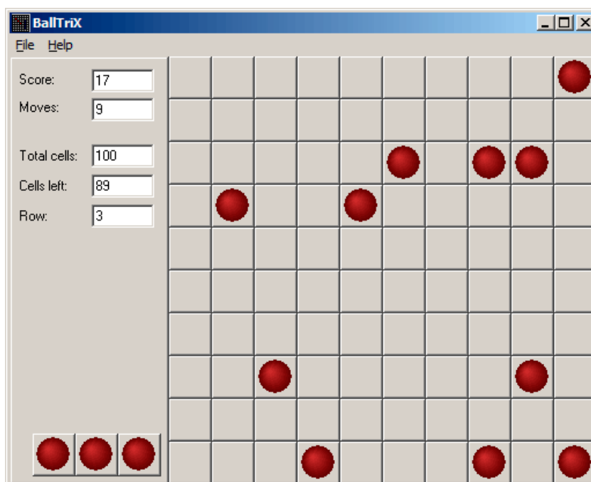
Рис. 8.6: Шутка сработала
