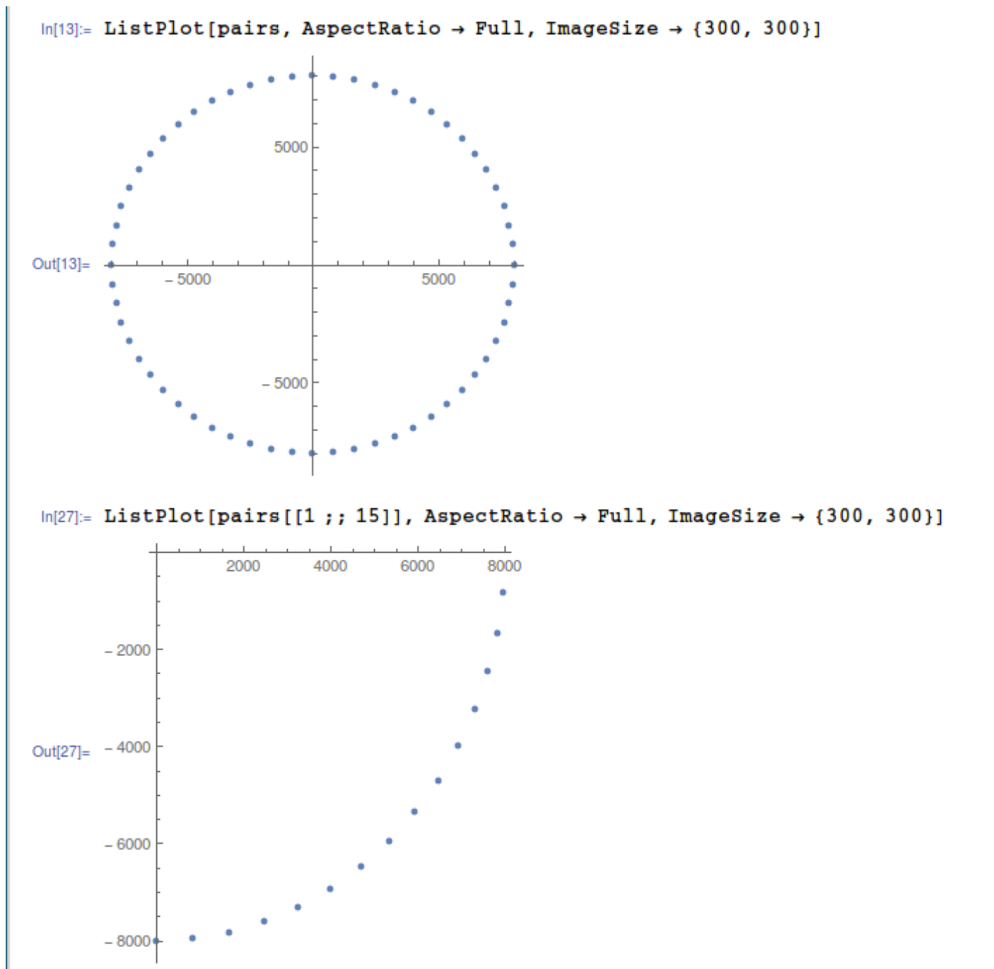
Рис. 8.12: Mathematica
