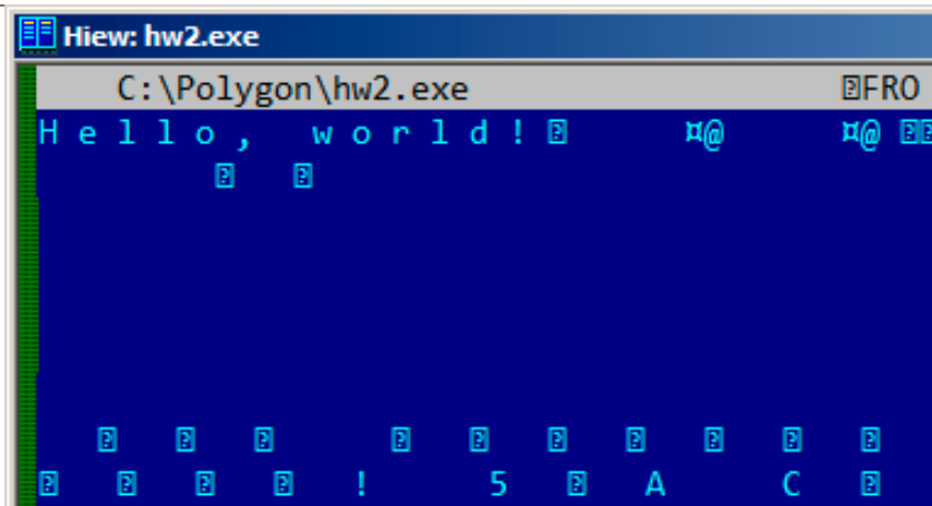
Рис. 5.3: Hiew
