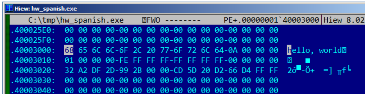
Рис. 1.1: Hiew
