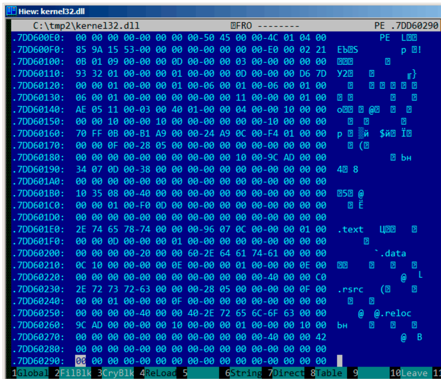
Рис. 9.5: PE-заголовок
