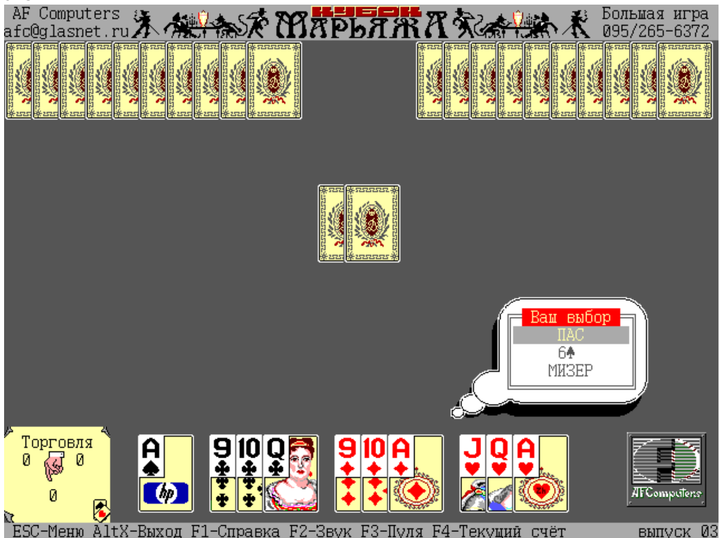
Рис. 8.19: "Торги"
