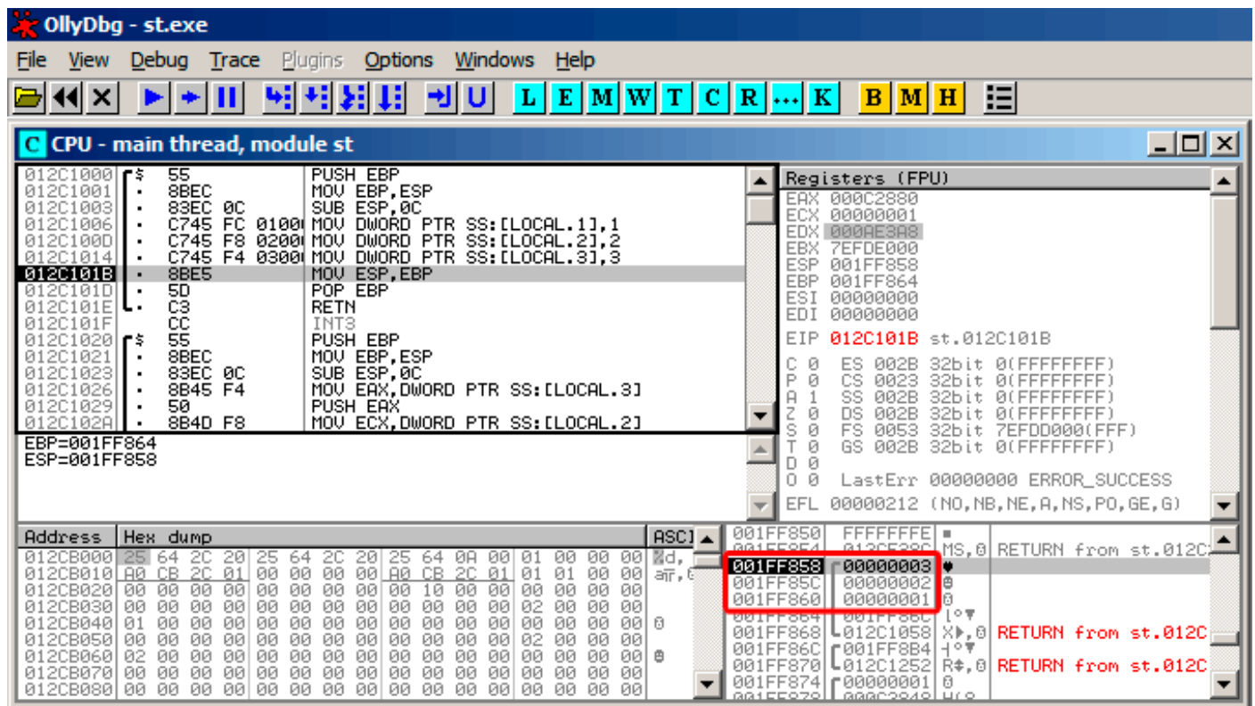
Рис. 1.5: OllyDbg: f1()
