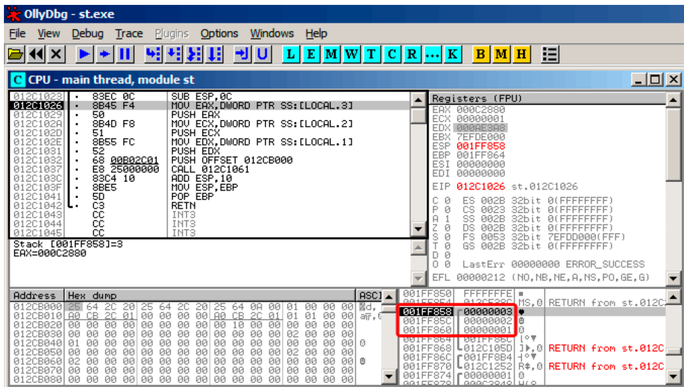
Рис. 1.6: OllyDbg: f2()
