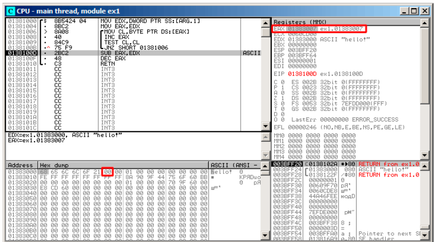
Рис. 1.52: OllyDbg: сейчас будет вычисление разницы указателей
