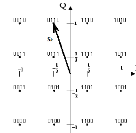
Рис.2.2. Созвездие сигнала 16-КАМ
