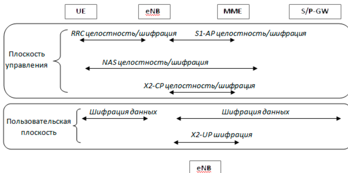
Рис.4.16. Реализуемые процедуры безопасности в сети E-UTRAN
