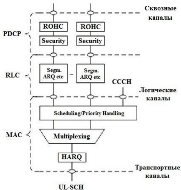
Рис. 4.XX. Структура уровня L2 при передаче вверх
