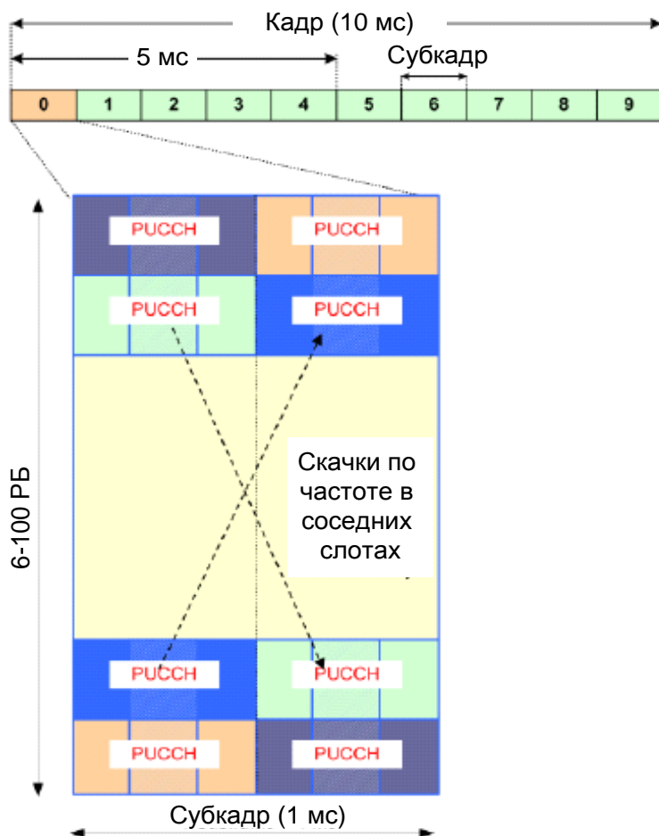
Рис.3.27. Размещение каналов PUCCH в субкадре
