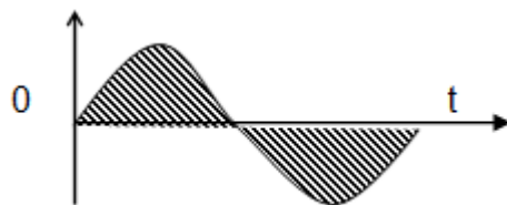
Рис.2.5. К определению площади синусоиды
