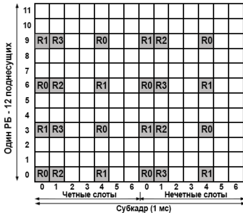
Рис.2.13. Позиционирование символов опорных сигналов в ресурсном блоке при передаче вниз
