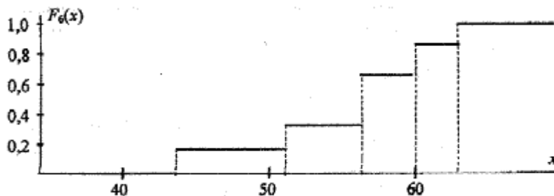
Рис. 2.1. Эмпирическая функция распределения
