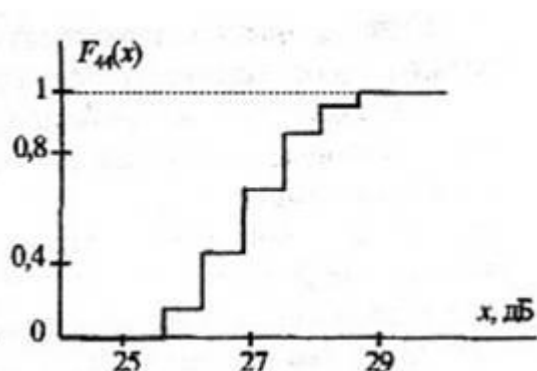
Рис. 2.3. Эмпирическая функция распределения
