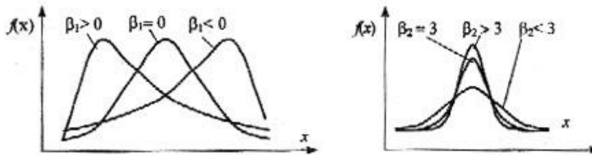
Рис. 2.4. Асимметрия распределения Рис. 2.5. Эксцесс распределения
