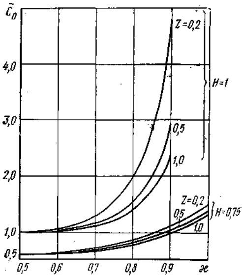
Рис. 6.2. Зависимости среднего числа повторных вызовов \bar{c}_0 от удельной поступающей нагрузки на одну линию пучка x при v=20
