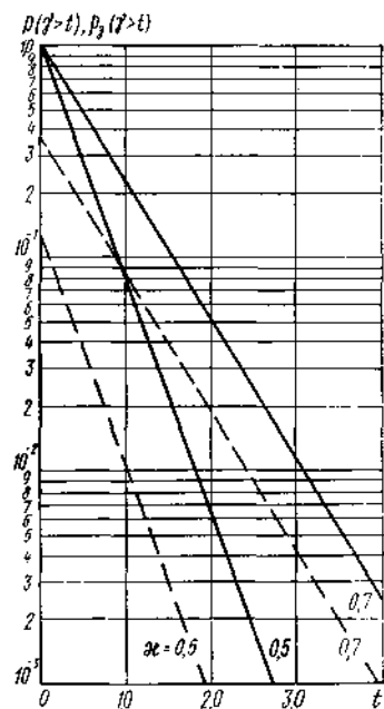
Рис. 5.1. Зависимости p(\gamma > t) = f(t) и p_0(\gamma > t) = f(t) при \nu = 5 и показательном распределении длительности занятия
