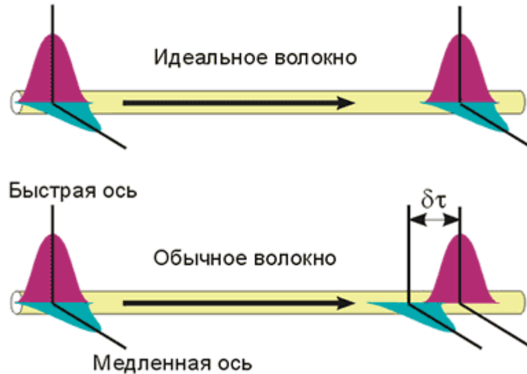
Рис. 6.19. Механизм возникновения поляризационно-модовой дисперсии
