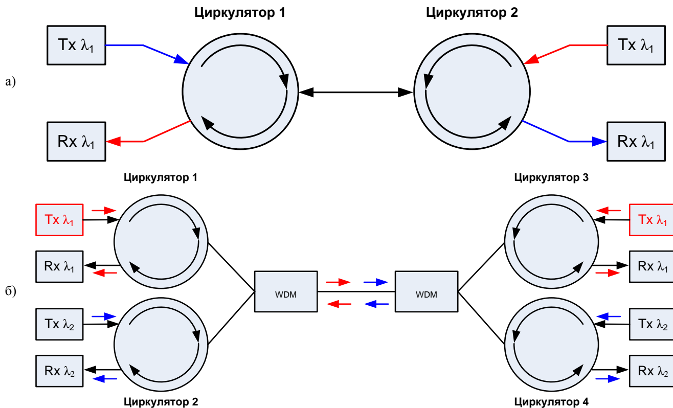
Рис. 7.31. Использование циркуляторов для организации дуплексной связи по одному ОВ на одной длине волны: а – организация одного канала, б – организация двух каналов.
