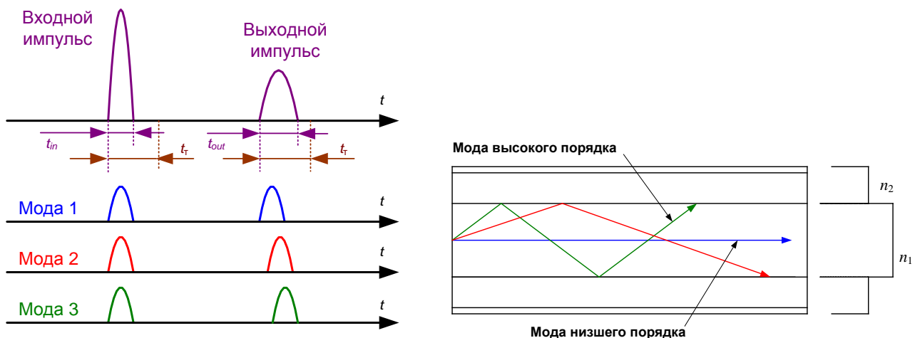
Рис.5.6. Межмодовая дисперсия в ММ ОВ со ступенчатым ППП.
