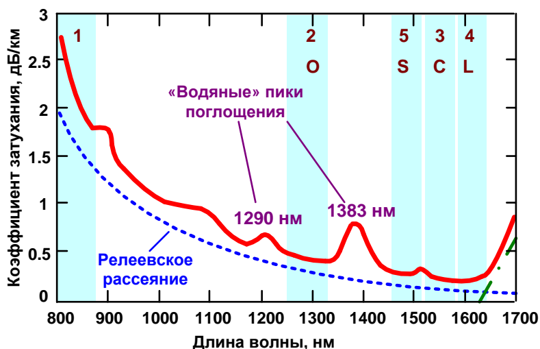
Рис. 4.1. Зависимость коэффициента затухания от длины волны и положение окон прозрачности в кварцевых ОВ
