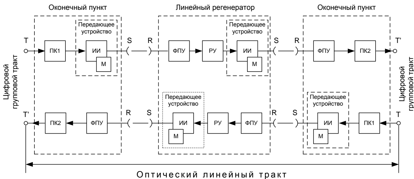
Рис.1.4. Общая схема передачи цифровых сигналов по волоконному тракту (ВТ). Оптический линейный тракт ЦСП с плезеохронной или синхронной иерархией.
