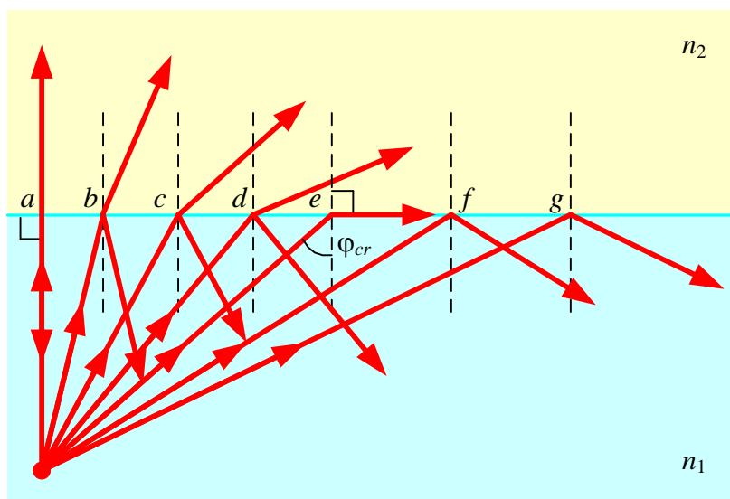
Рис. 2.2. Полное внутреннее отражение.
