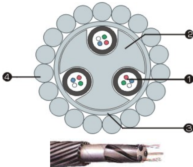
б) ОКГТ с профилированным алюминиевым сердечником, содержащим оптические модули в спирально расположенных пазах
