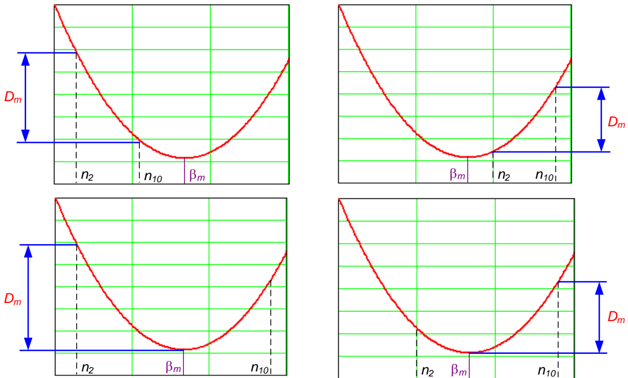
Рис. 5.12. Расчет коэффициента межмодовой дисперсии.
