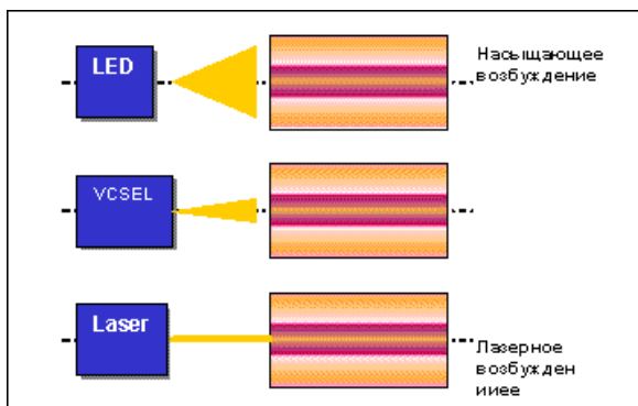
Рис. 5.16. Ввод излучения в волокно от различных источников
