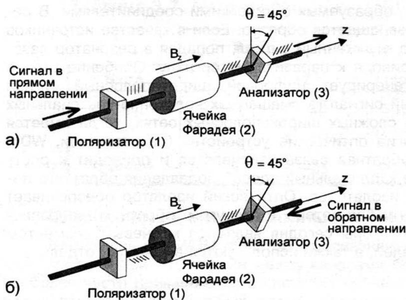
Рис. 7.23. Схема оптического изолятора.
