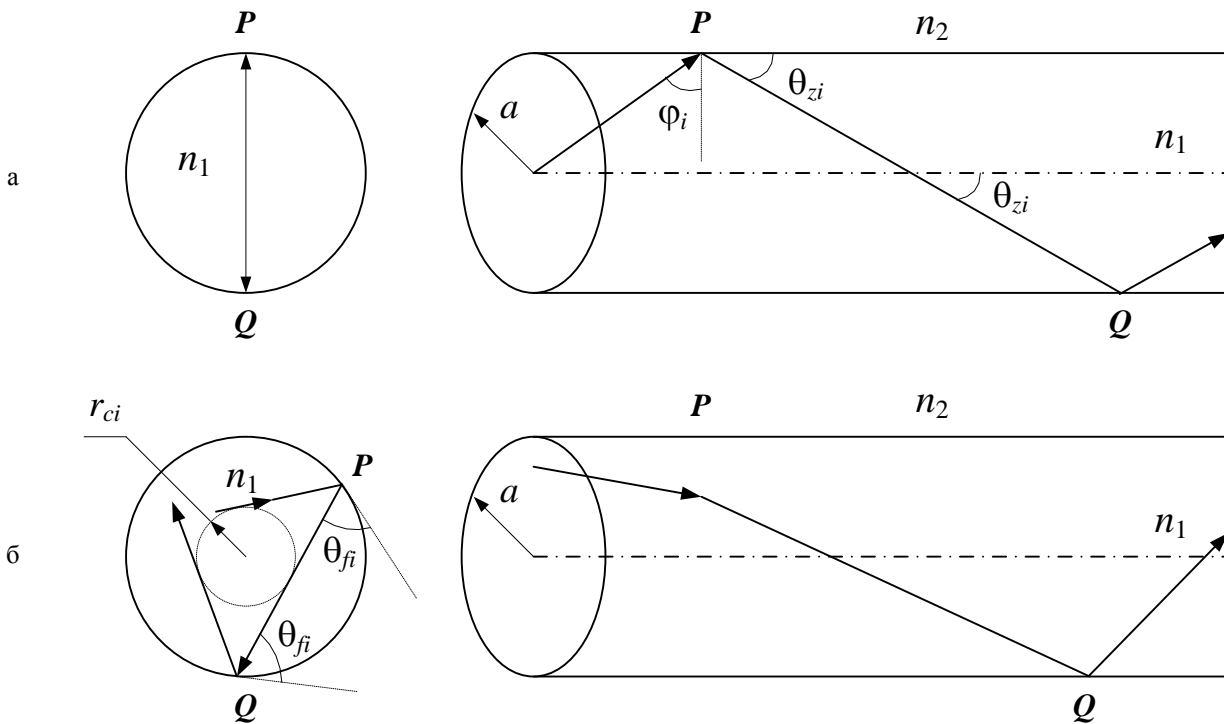
Рис.5.3. Траектории лучей в ММ ОВ со ступенчатым профилем показателя преломления.
