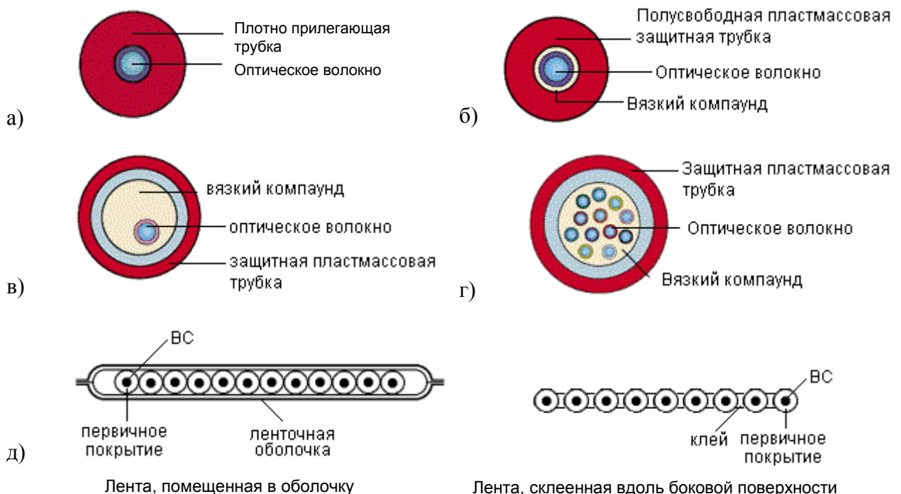
Рис. 3.8. Типы вторичного покрытия оптических волокон: а) сплошное; б) полусвободное трубчатое; в) свободное трубчатое; г) многоволоконное свободное трубчатое; д) ленточное.
