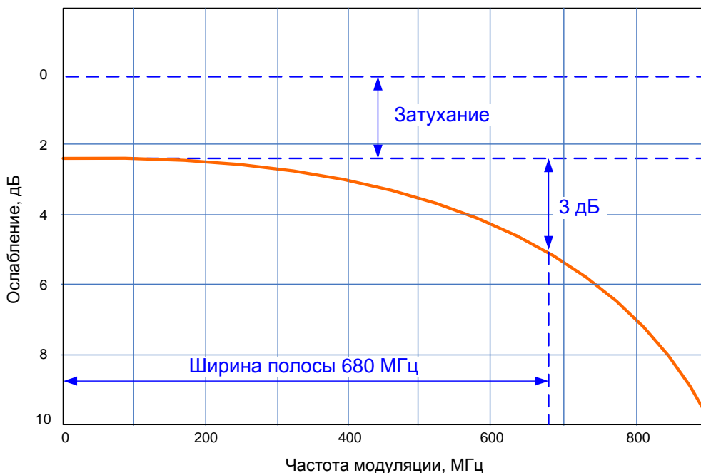
Рис. 5.8. Понятие широкополосности ОВ.
