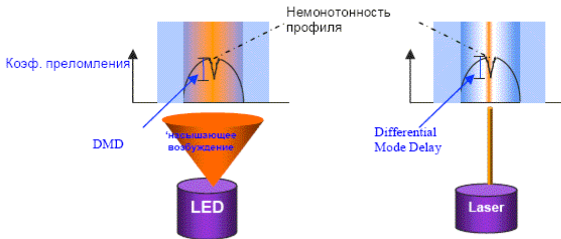
Рис. 5.17. Использование светоизлучающего диода и лазера с ММ ОВ.
