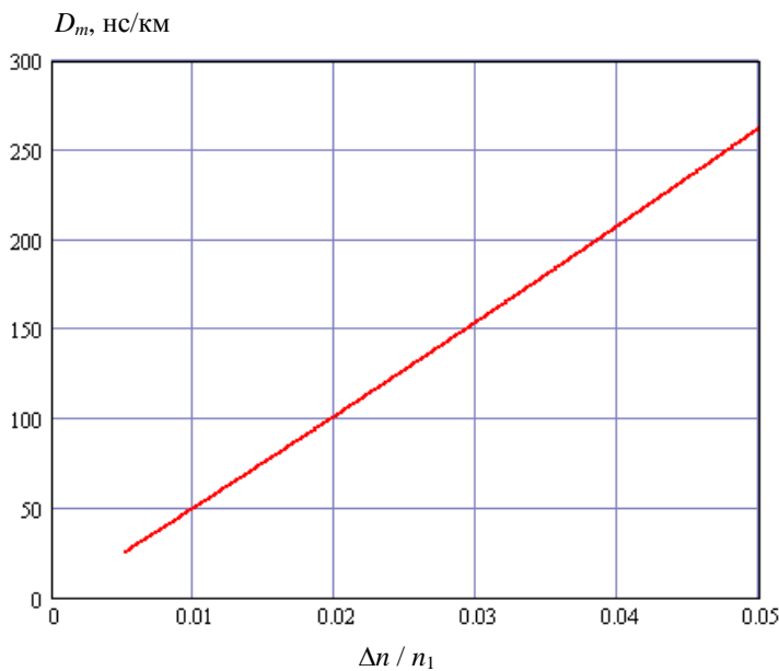
Рис. 5.7. Зависимость коэффициента межмодовой дисперсии от относительной разности показателей преломления сердцевины и оболочки \Delta n / n_1 = (n_1 - n_2) / n_1 .
