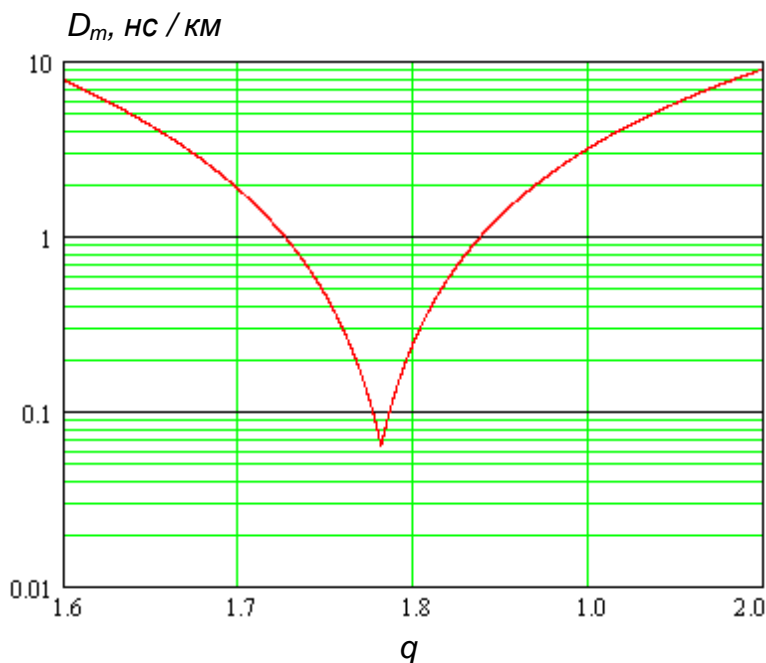
Рис. 5.14. Зависимость межмодовой дисперсии от показателя степенного профиля
