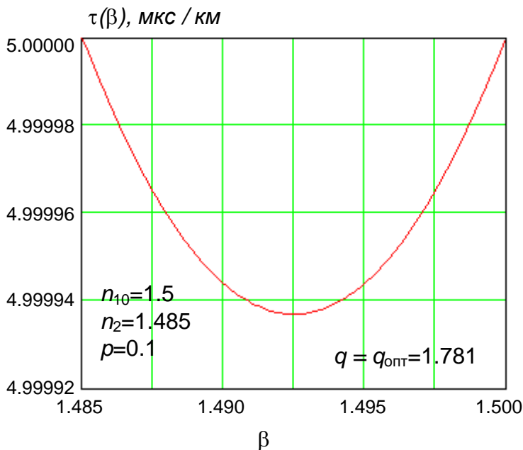
Рис. 5.13. Зависимость удельного времени задержки от величины инварианта для оптимального показателя степенного профиля
