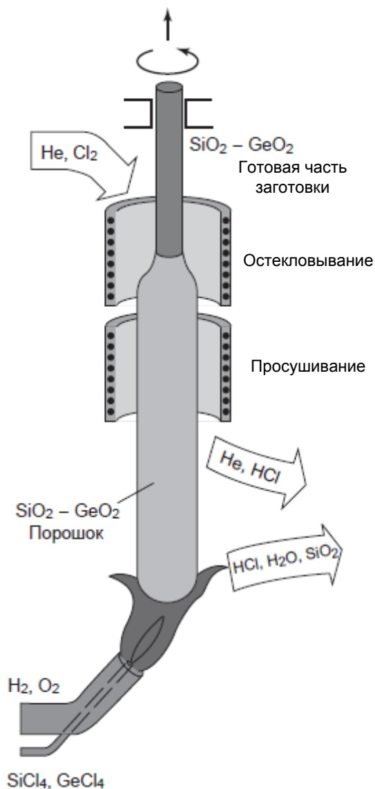
Рис. 3.5. Производство заготовки методом осевого парофазного осаждения
