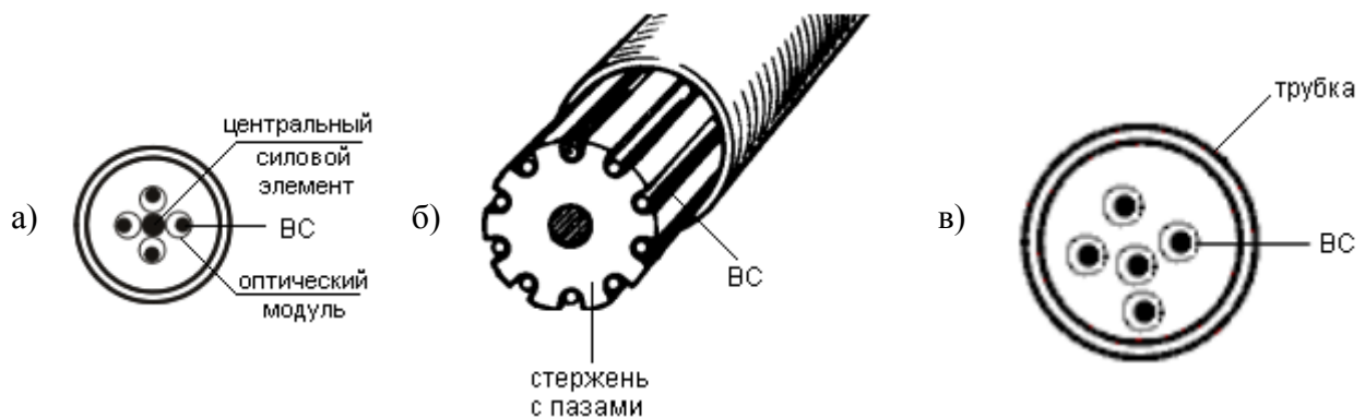
Рис.3.9. Основные конструкции сердечников ОК: а) повивный; б) профилированный; в) центральный.
