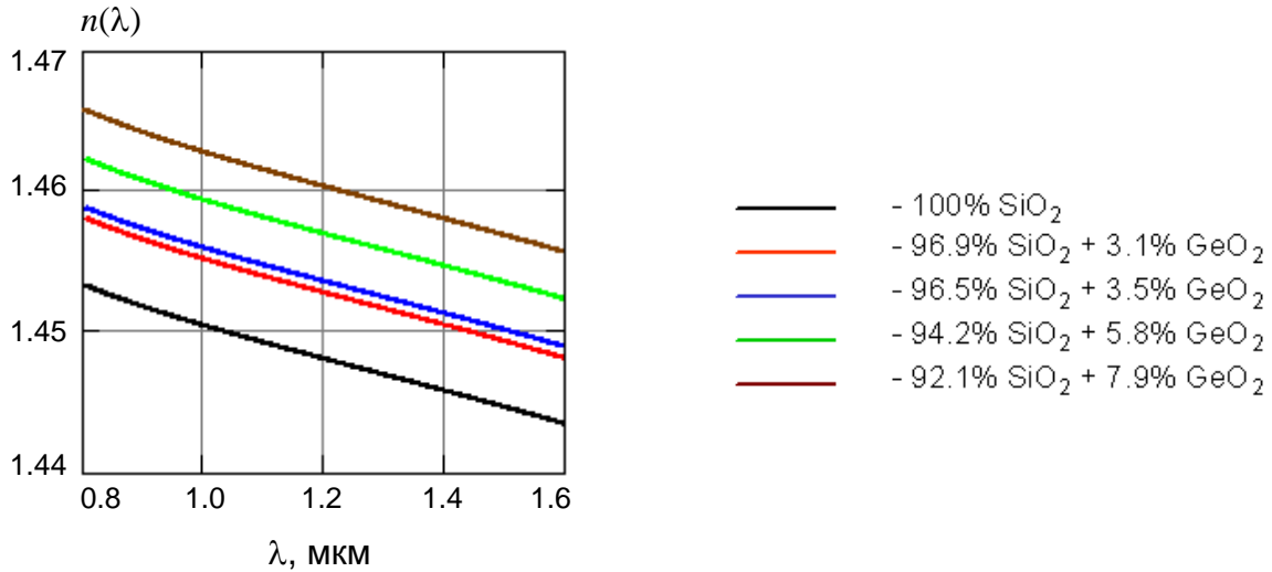
Рис. 5.5. Зависимости показателя преломления от длины волны.
