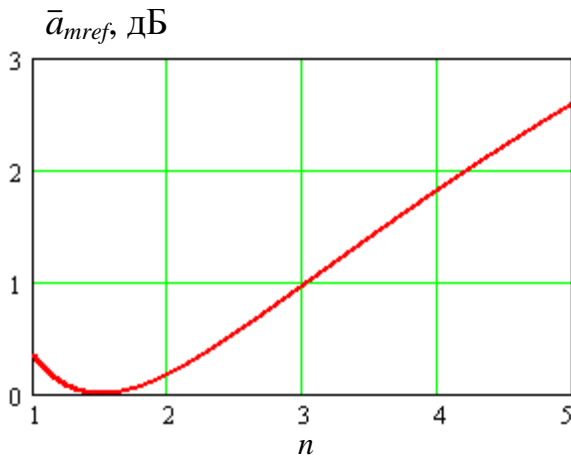
Рис. 7.9. Зависимость средних вносимых потерь от показателя преломления среды в зазоре.
