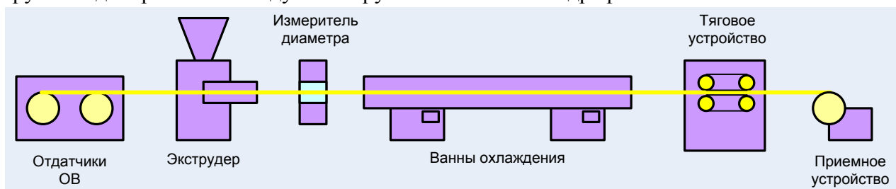
Рис. 3.15. Упрощенная схема экструзионной линии.
