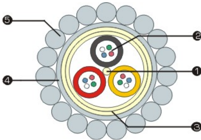
а) ОКГТ с сердечником повивной скрутки, содержащим оптические модули, в алюминиевой трубе
