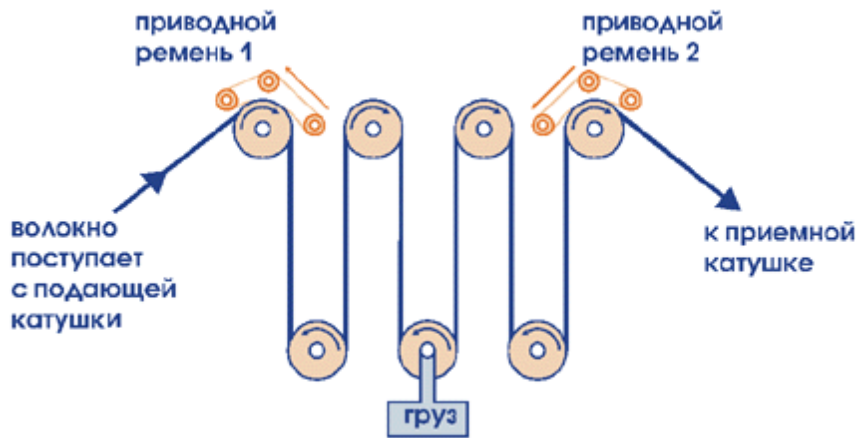
Рис. 3.7. Установка для перематки ОВ с натяжением
