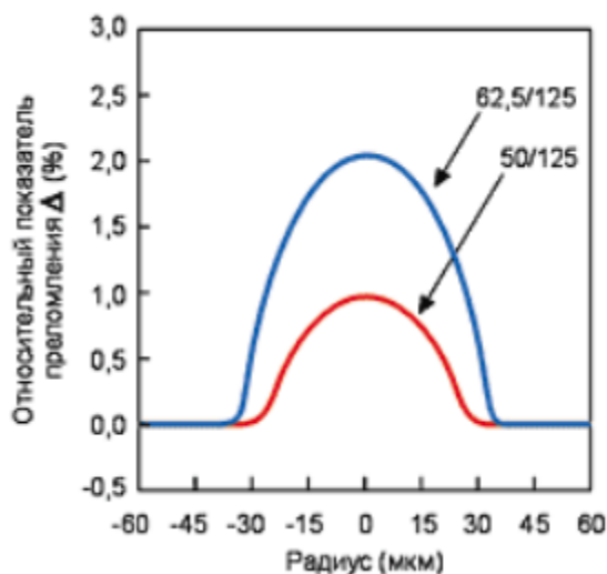
Рис. 5.15. Профили показателей преломления волокон 50/125 и 62,5/125.
