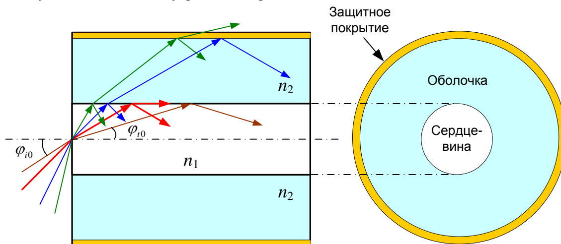
Рис. 5.1. Моды в ступенчатом ВС
