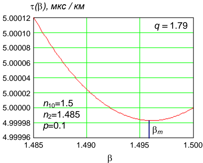
Рис. 5.11. Зависимость удельного времени задержки от величины первого инварианта.
