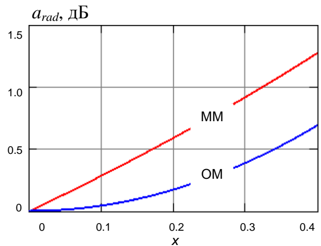
Рис. 7.5. Потери от радиального смещения соединяемых ОВ
