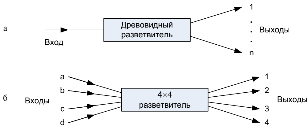
Рис. 7.26. Типы разветвителей: а) древовидный, б) звездообразный.
