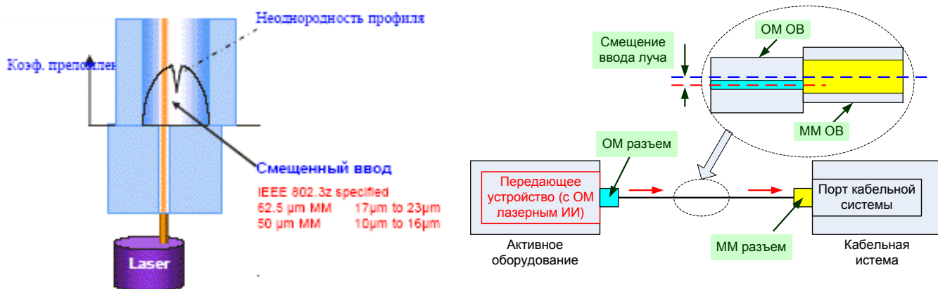
Рис. 5.18. Принцип и схема смещенного ввода светового луча в ММ ОВ
