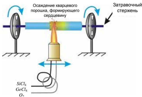
Рис. 3.4. Производство заготовки методом внешнего парофазного осаждения.
