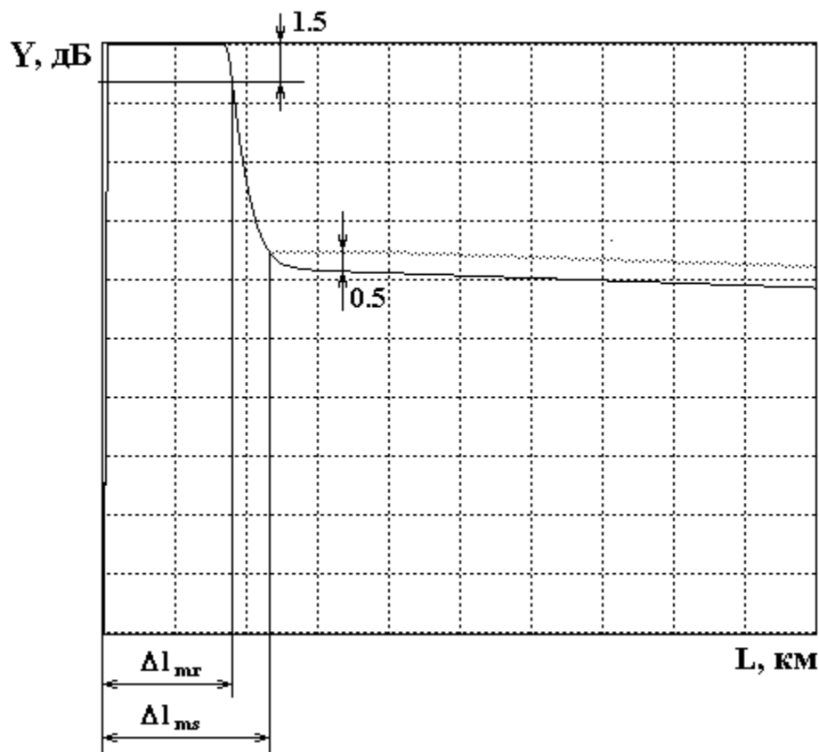
Рис. 10.16 Мертвая зона
