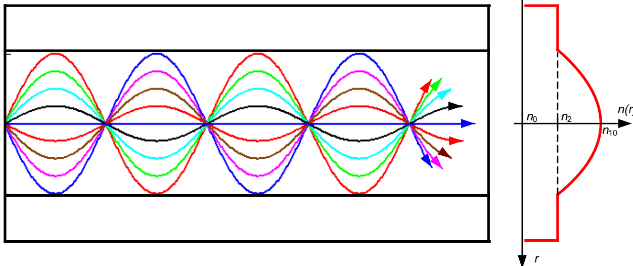
Рис. 5.10. Траектории меридиональных лучей в ВС с усеченным степенным профилем показателя преломления.
