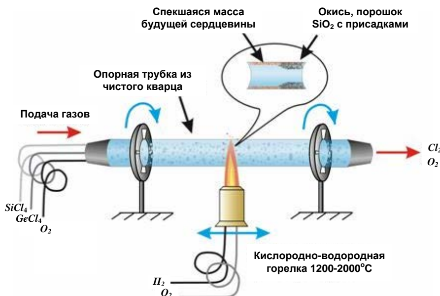
Рис. 3.2. Производство заготовки методом внутреннего парофазного осаждения
