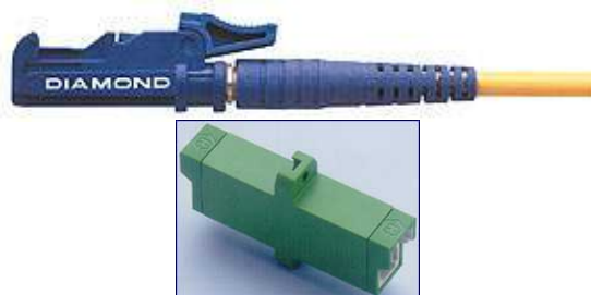
Рис. 7.18. Малогабаритный соединитель E-2000
