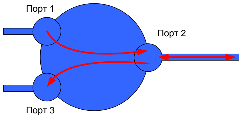
Рис. 7.30. Оптический циркулятор.
