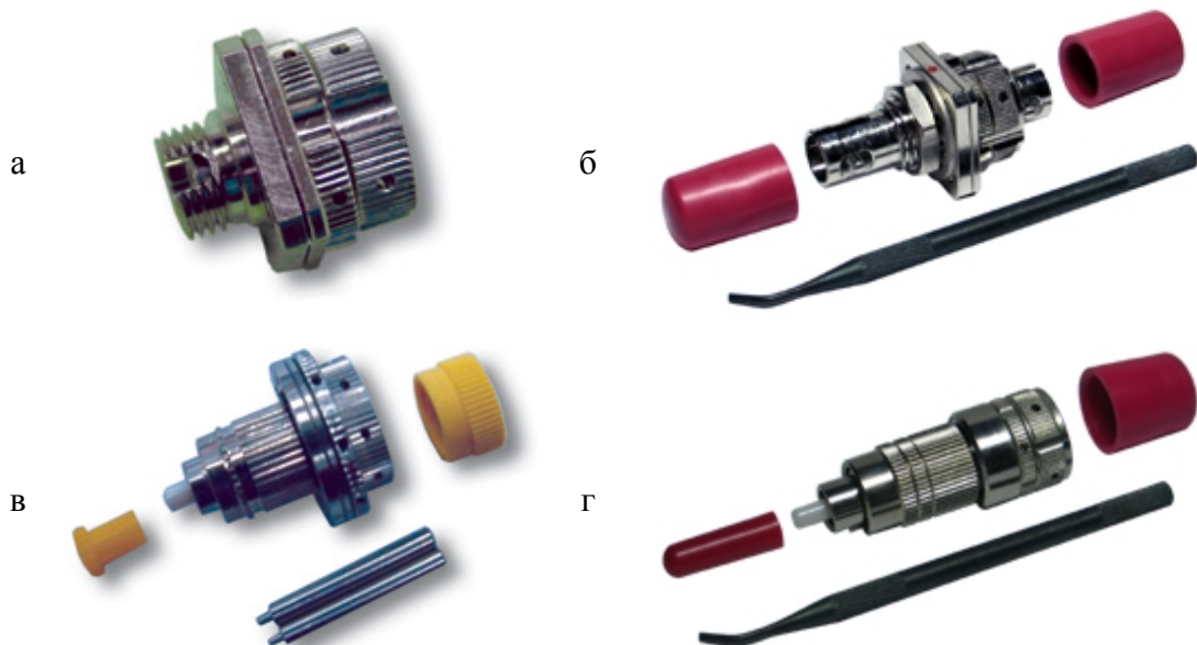
Рис. 7.25. Перестраиваемые аттенюаторы розетка-розетка (а, б) и вилка-розетка (в, г).
