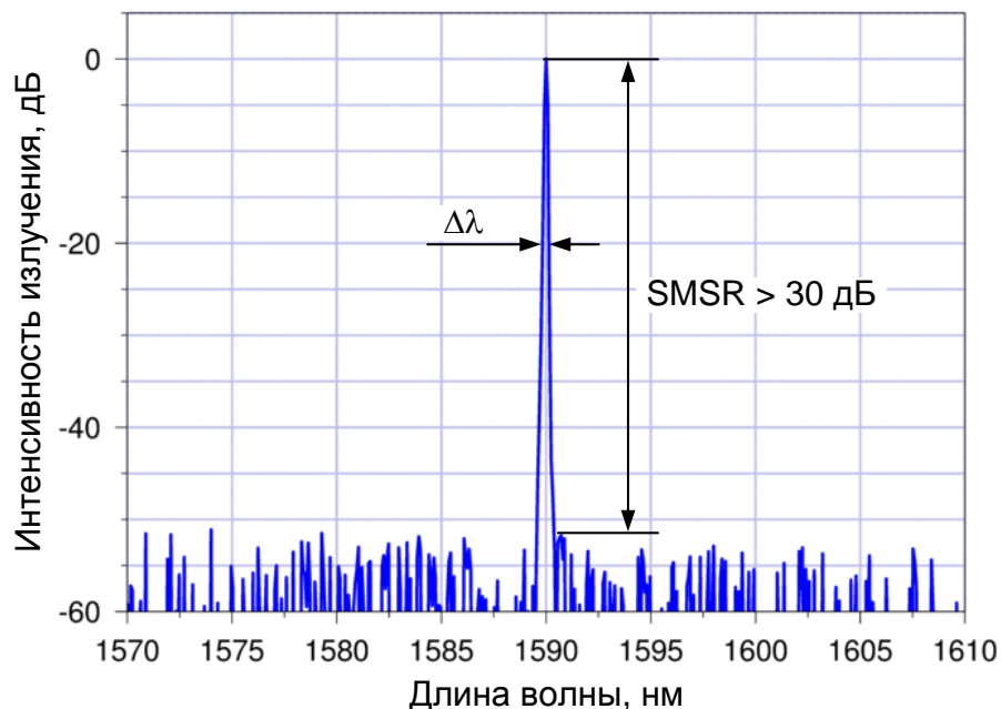
Рис. 8.18. Спектр излучения ЛД DFB
