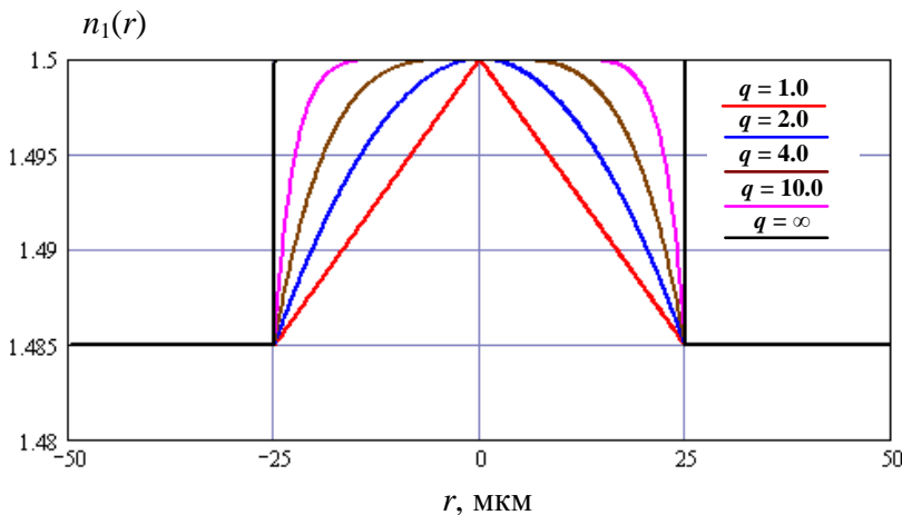
Рис. 5.9. Усеченные степенные профили показателя преломления.
