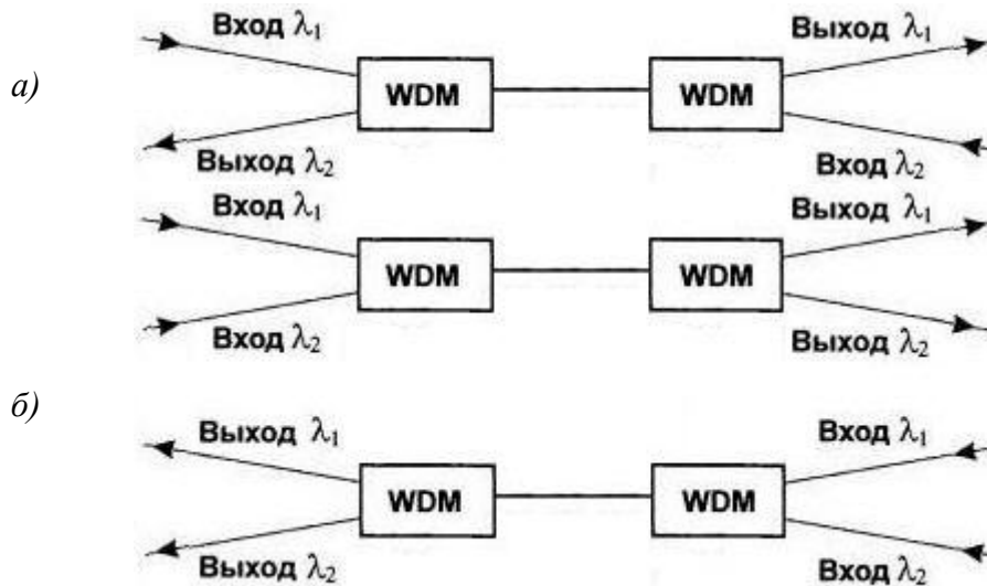
Рис. 7.29. Использование мультиплексоров/демультиплексоров WDM для ВОСП, работающих по одному (а) и по двум ОБ (б).
