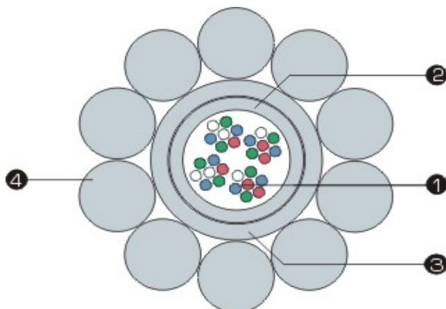
в) Центральный сердечник из нержавеющей стали с плотной укладкой волокон, заключенный в алюминиевую трубку
