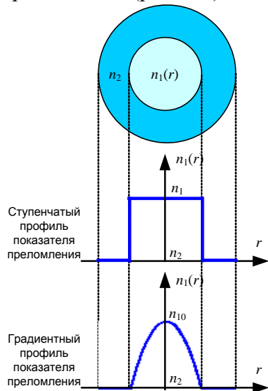
Рис. 5.2. Ступенчатый и градиентный профили показателя преломления
