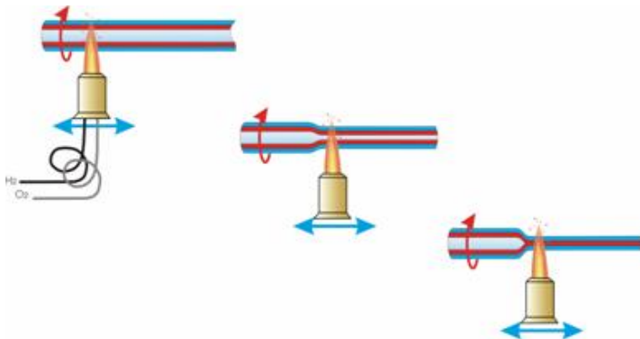
Рис. 3.3. Усаживание заготовки
