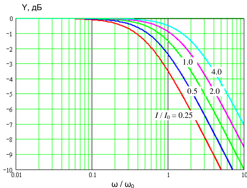
Рис. 8.10. Семейство амплитудно-частотных характеристик СИД при малых входных сигналах
