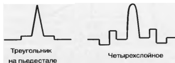
Рис. 6.9. Профили показателей преломления ОВ со смещенной дисперсией
