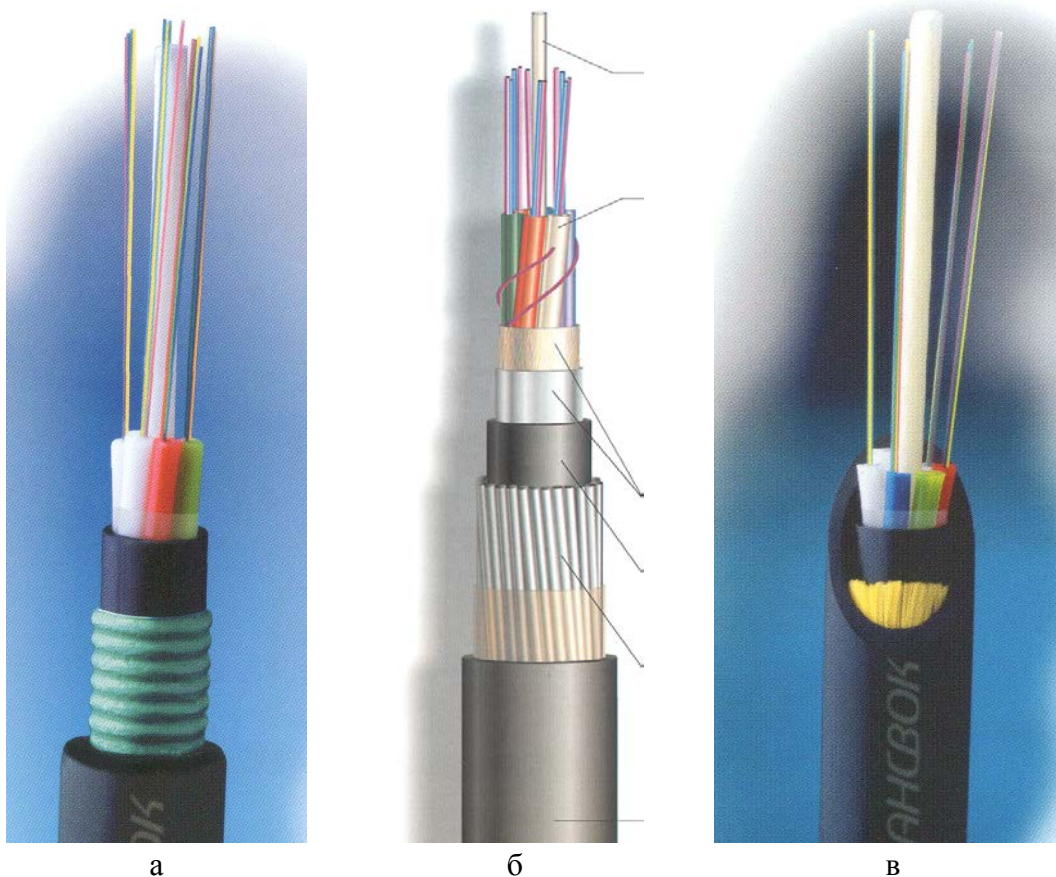
Рис. 3.11. Конструкции броневого покровов: а – ленточная, б – круглопроволочная, в – из арамидных нитей
