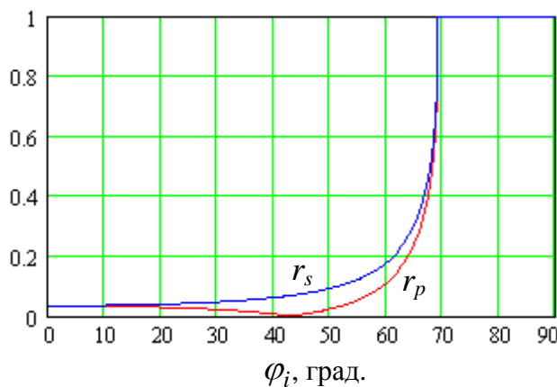
Рис. 2.5. Зависимости коэффициентов отражения от угла падения при падении светового луча из менее плотной оптической среды ( n_1=1.4 ) в более плотную ( n_2=1.5 ) (слева) и из более плотной оптической среды ( n_1=1.5 ) в менее плотную ( n_2=1.4 ) (справа).
