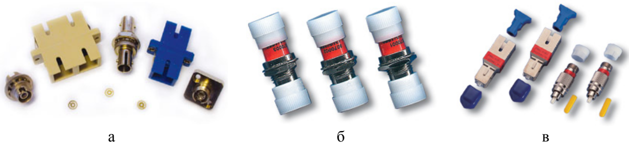
Рис. 7.24. Фиксированные аттенюаторы розетка-розетка (а, б) и вилка-розетка (в).
