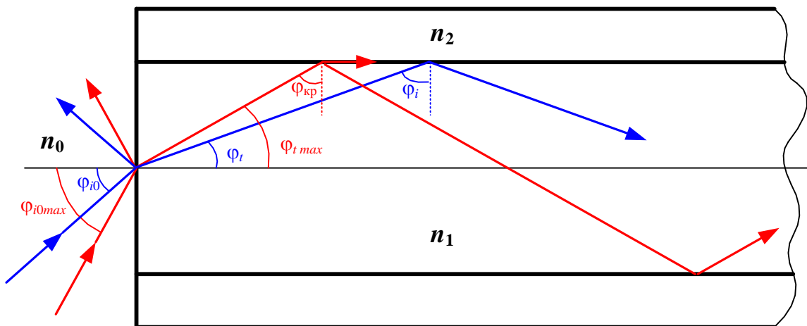
Рис.5.4. Ввод и распространение меридиональных лучей по ступенчатому ОВ
