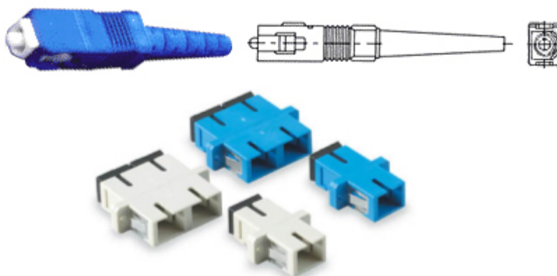
Рис. 7.16. Соединитель SC
