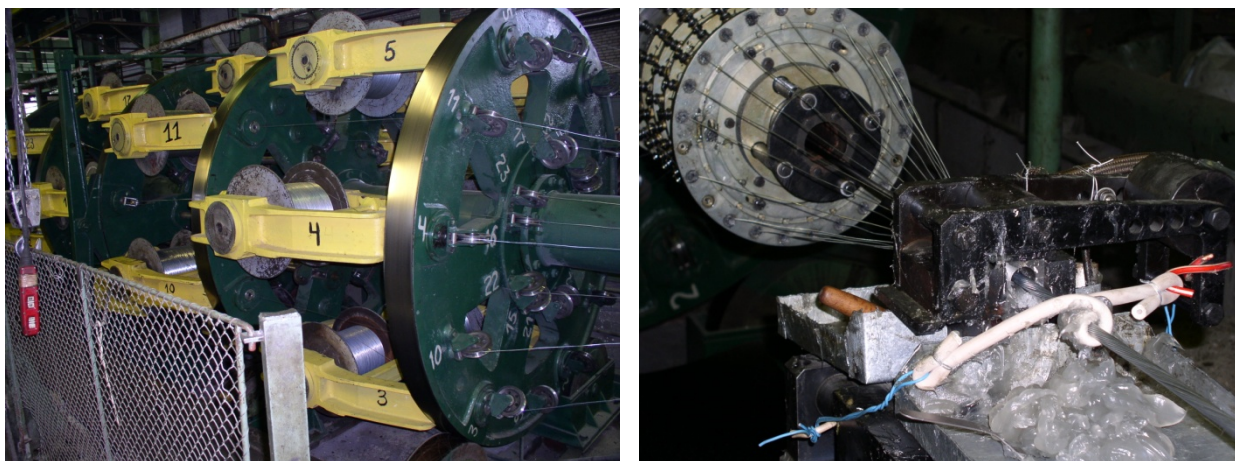
Рис. 3.17. Бронировочная машина.
