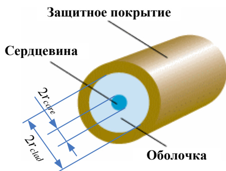
Рис. 3.1. Структура ОВ
