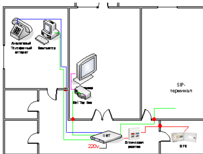
Рис.П.3.12. Схема предоставления услуг в помещении абонента. Тип и количество интерфейсов определяется на этапе проектирования.
