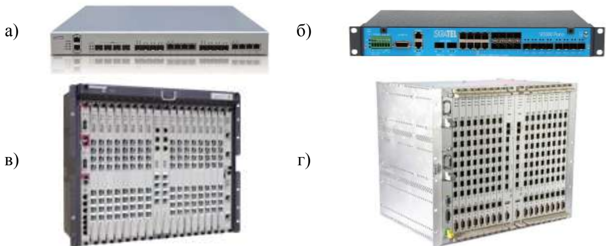
Рис. П.3.8. Внешний вид оборудования OLT: а) BW-5004-OLT ( Broadware Networks ), б) SI3000 Pono (Искрател), в) SmartAX 5680T (Huawei Technologies), г) MA-4000PX (Элтекс)
