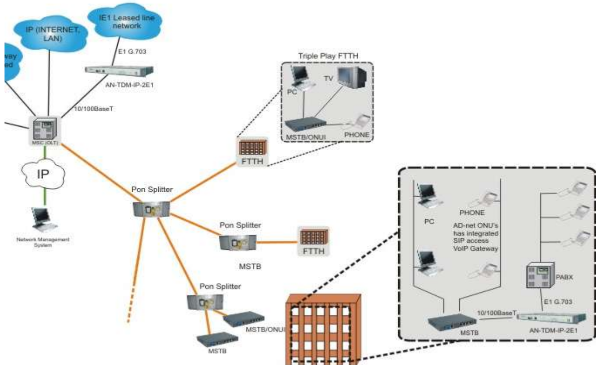
Рис.3.2. Структура построения сети FTTH.
