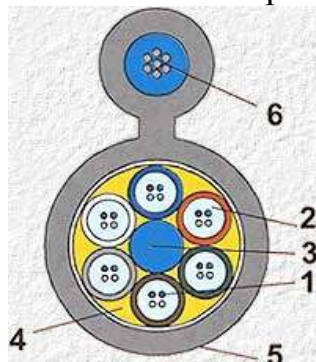
Рис. 9.9. Конструкция ВОК типа 8-ки.
