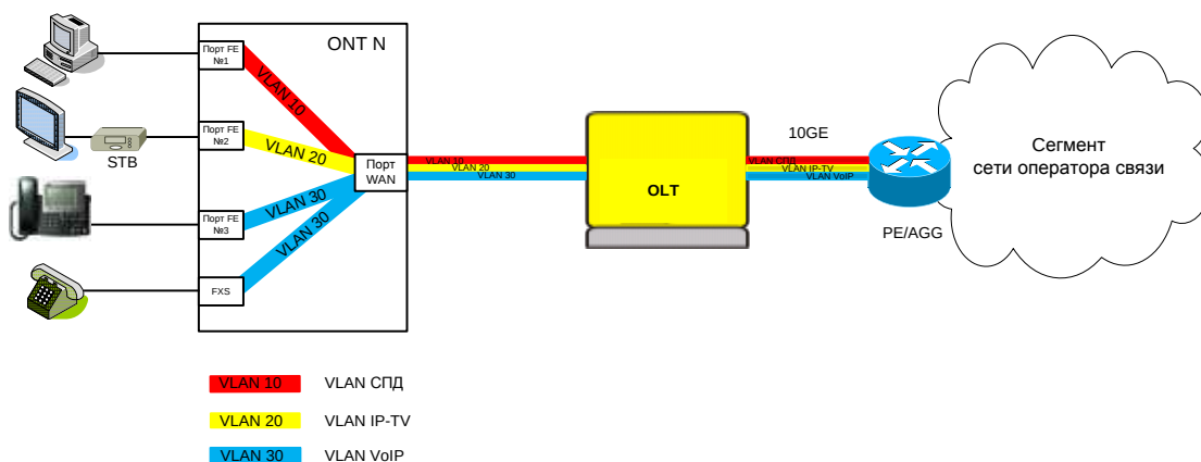
Рис.П.3.13. Назначение VLAN.
