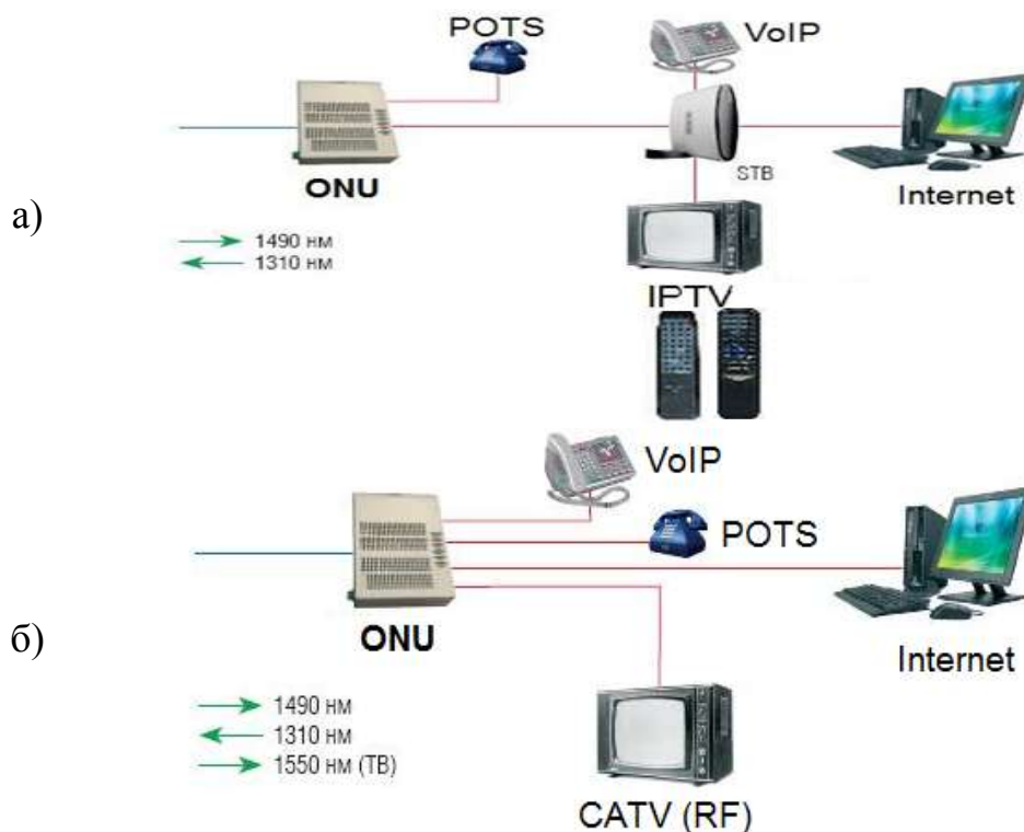
Рис.П.3.11. Предоставление услуг: а) по IP (телевизионный сигнал IPTV преобразуется в аналоговый с помощью TV-приставки STB); б) с использованием оптической поднесущей 1550 нм (TV-приёмник подключён непосредственно к ONU через разъём RF).
