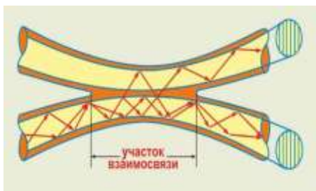
Рис.П.2.7. Сплиттеры сплавного типа.
