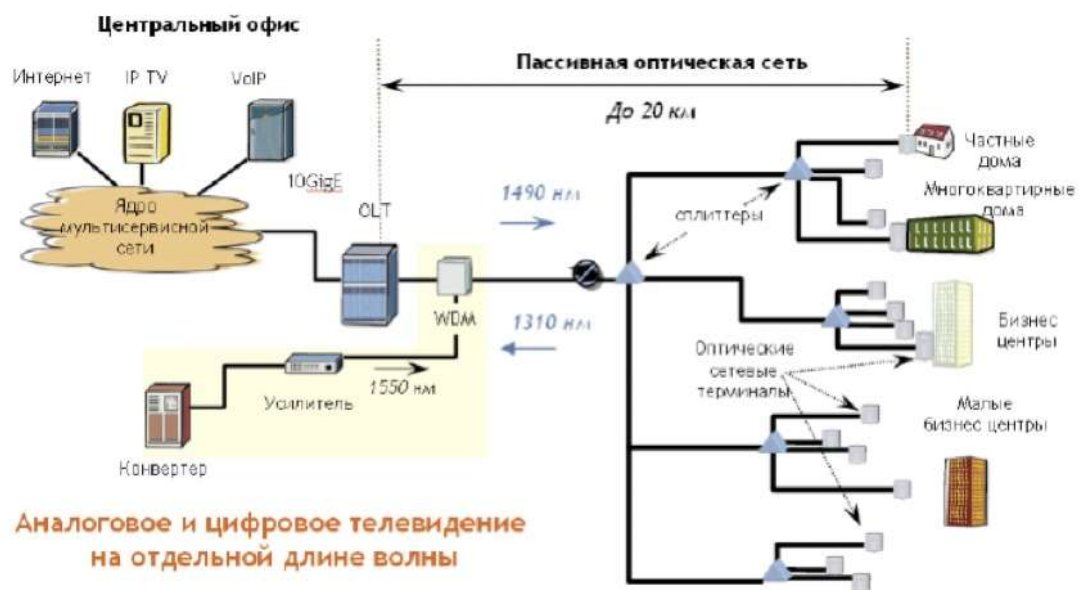
Рис.П.3.1. Типовая схема решений для оборудования PON Alcatel-Lucent
