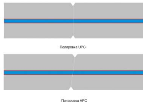
Рис.П.2.13. Полировка торца.
