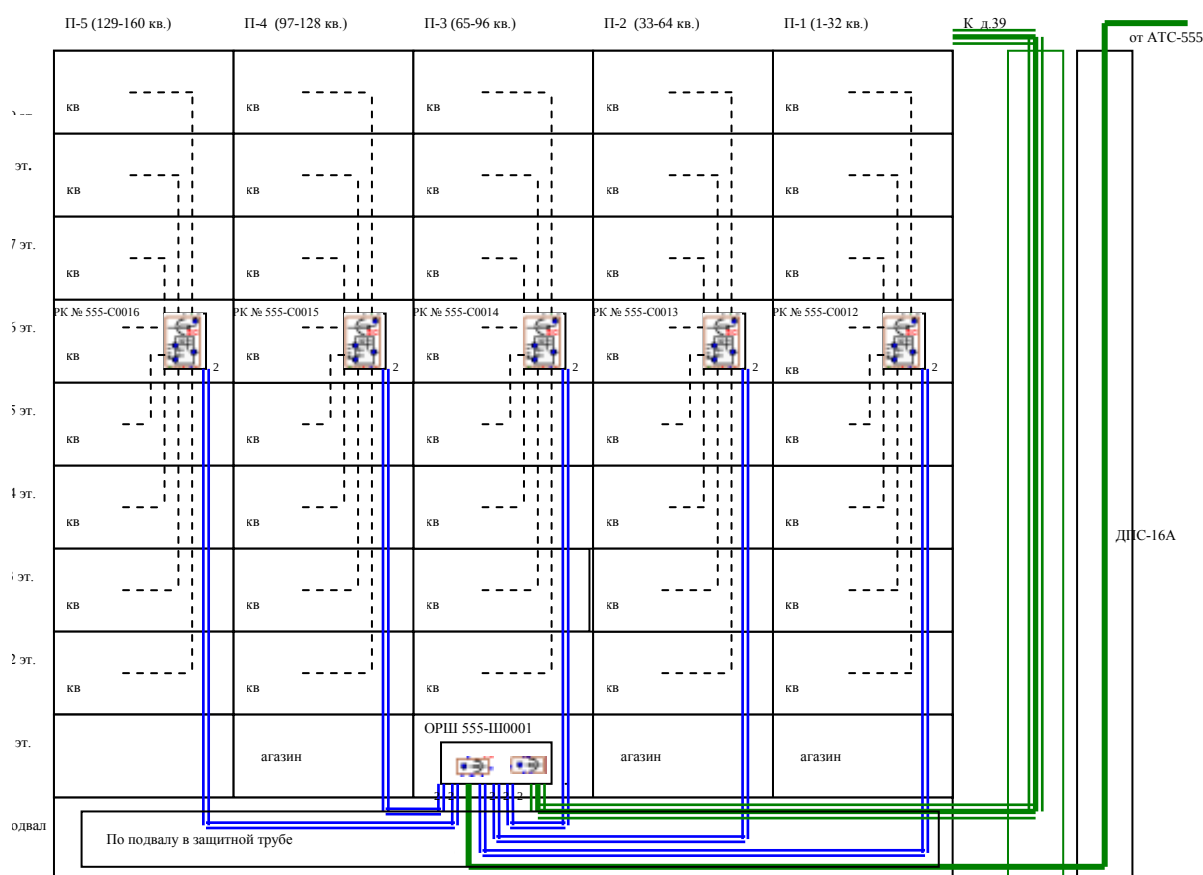
Рис.7.1. Структура домового распределительной сети.
