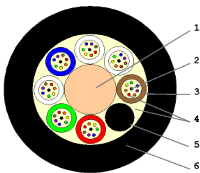
Рис.9.4. ВОК для пневмопрокладки
