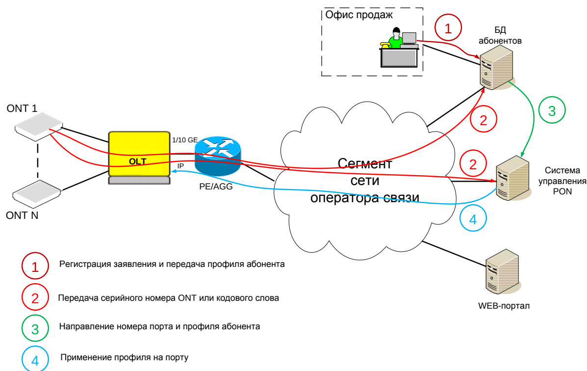
Рис.П.3.14. Подключение абонента
