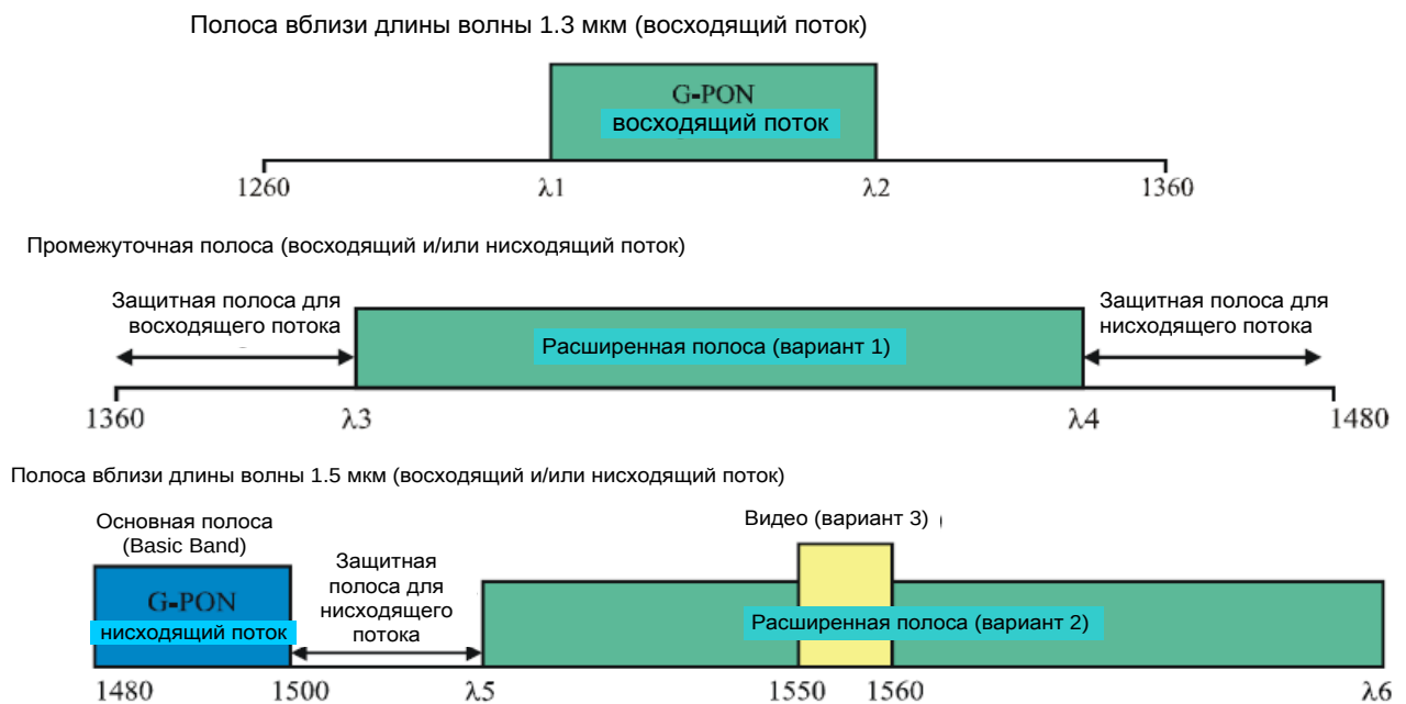
Рис. П.3.7. Распределение длин волн в сетях GPON.
