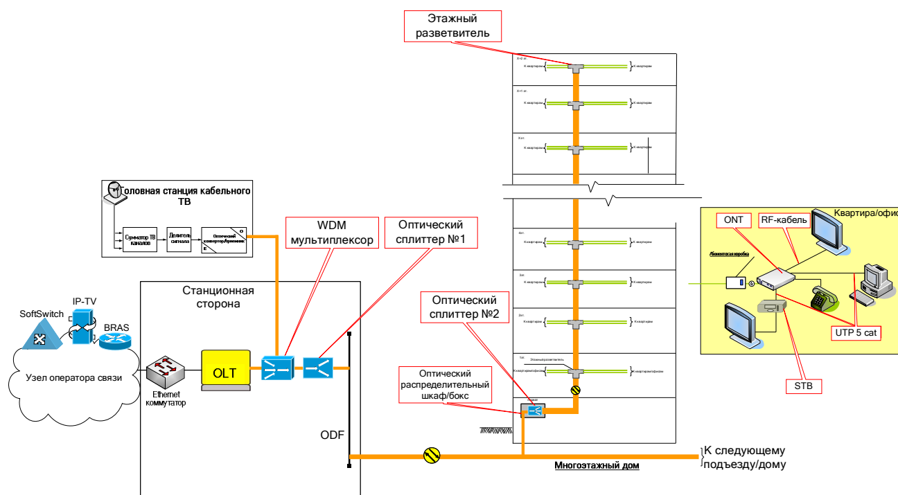
Рис. 5.4. Типовая функциональная схема организации связи по технологии PON при городской (многоэтажной) застройке.
