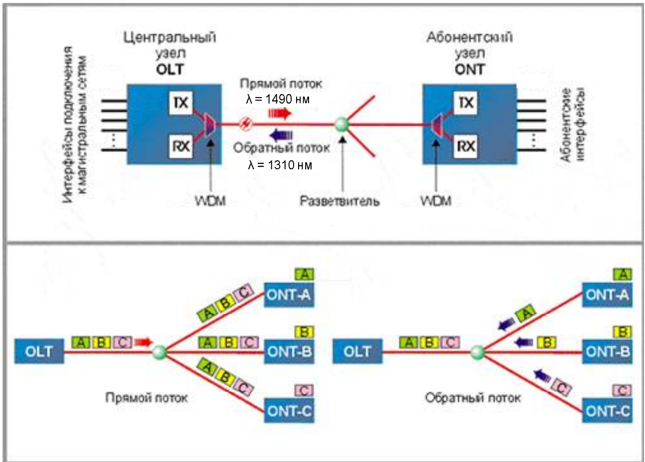
Рис.4.1. Принцип работы сети PON.
