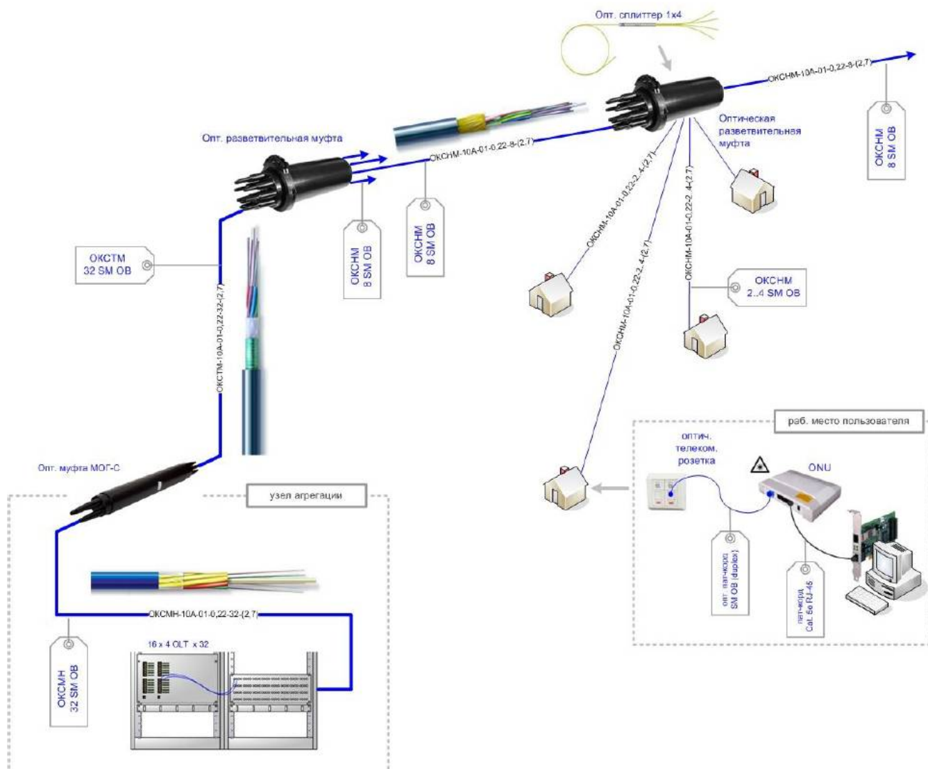
Рис. 5.6. Структурная схема кабельных магистралей PON P2MP топологии «дерево» в условиях малоэтажной застройки.
