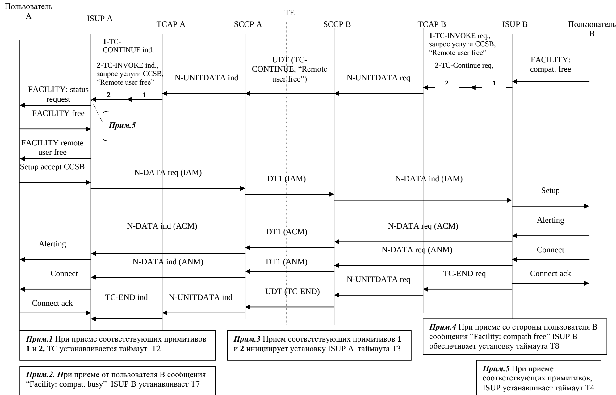
Рис.3 Упрощенная стрелочная диаграмма успешного выполнения сетью услуги CCBS
