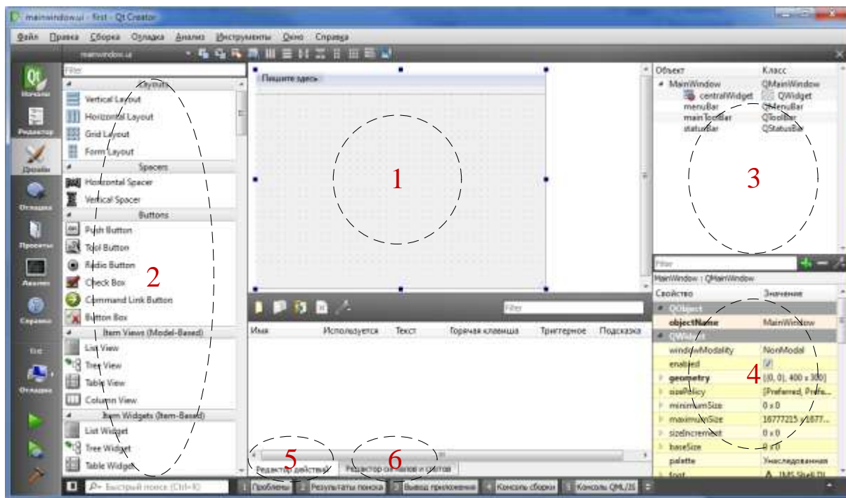
Рисунок 6. Разработка интерфейса пользователя
