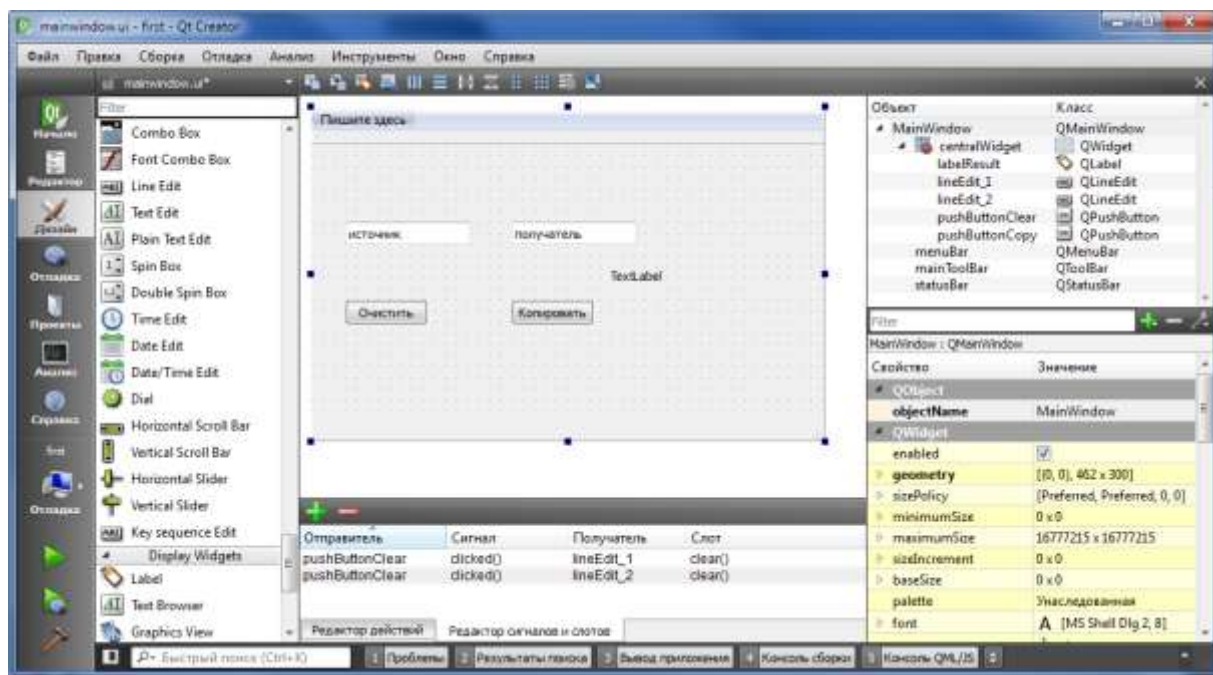
Рисунок 9. Добавление сигналов и слотов
