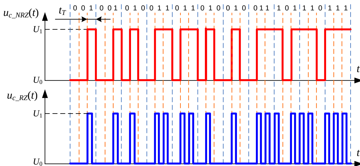
Рис. 3.3. Получение модулирующего сигнала
