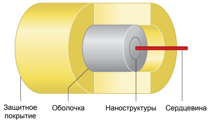
Рис. 6.14. Конструкция ОВ G.657
