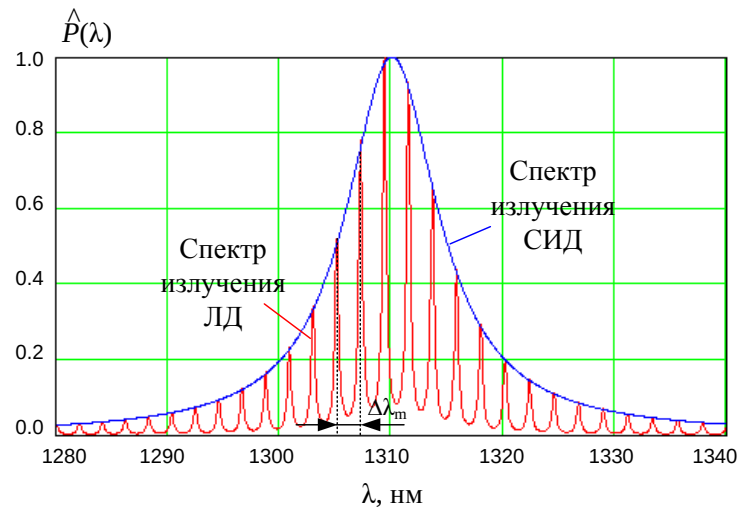
Рис. 2.14. Спектр излучения ФР лазера
