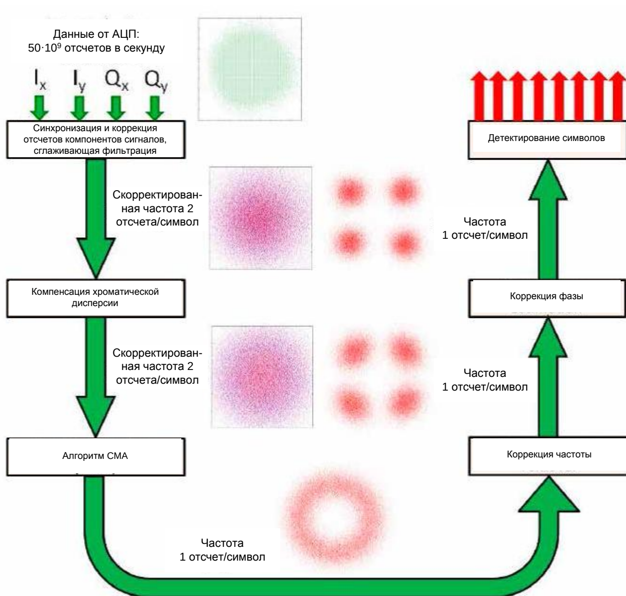
Рис. 5.12. Операции, выполняемые блоком ЦОС.
