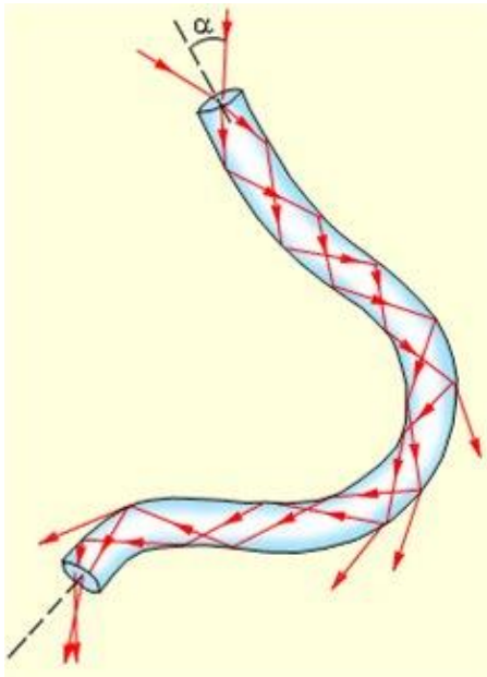
Рис. 6.13. Потери излучения на изгибах
