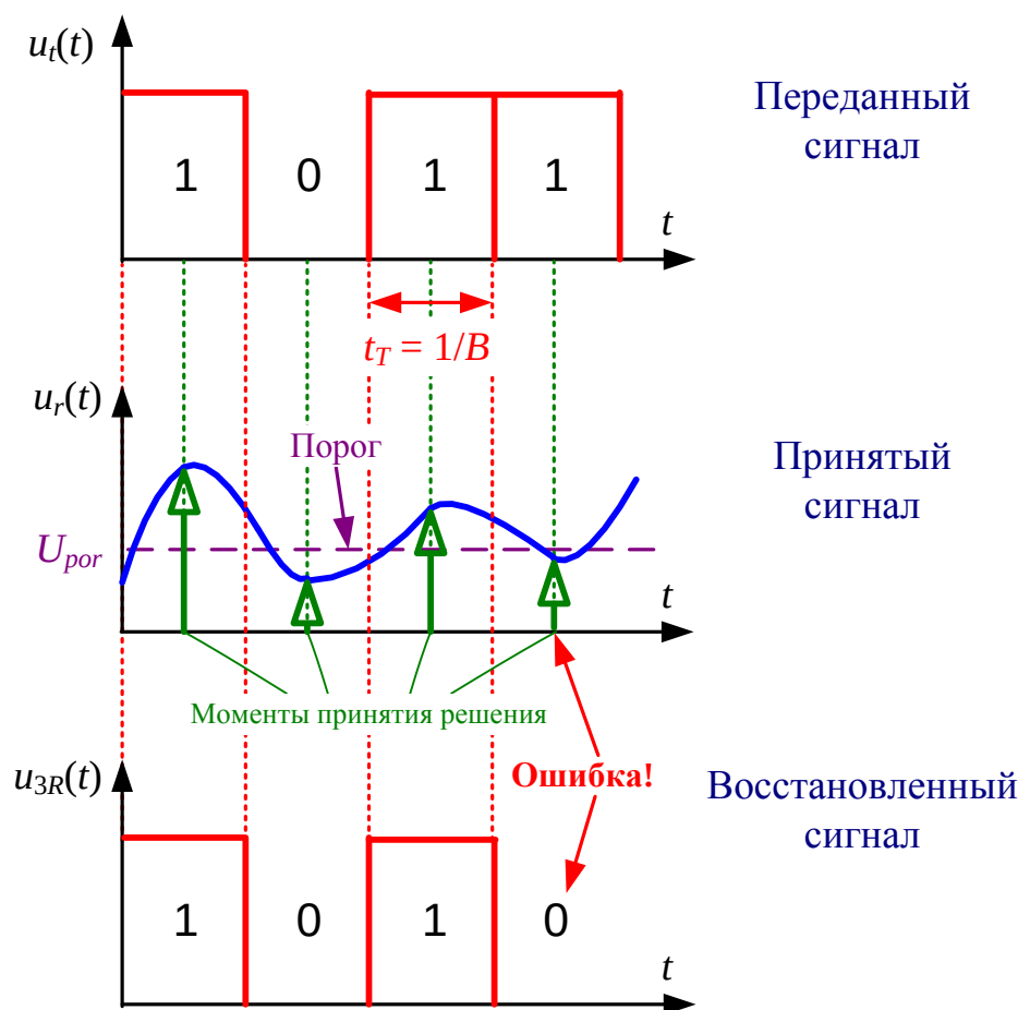
Рис. 5.6. Регенерация сигнала в формате NRZ: u_t(t) – исходный (модулирующий) сигнал, u_r(t) – принятый сигнал на входе регенератора, u_{3R}(t) – сигнал на выходе регенератора.
