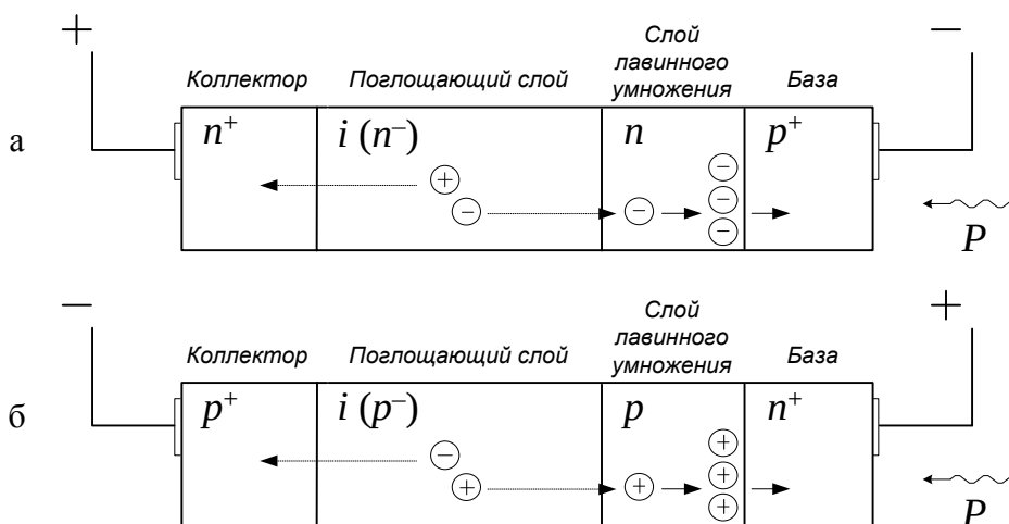
Рис. 4.4. Лавинные ФД
