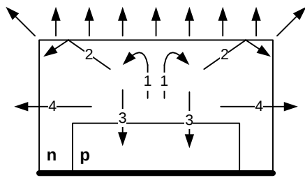
Рис. 2.1. Вывод излучения
