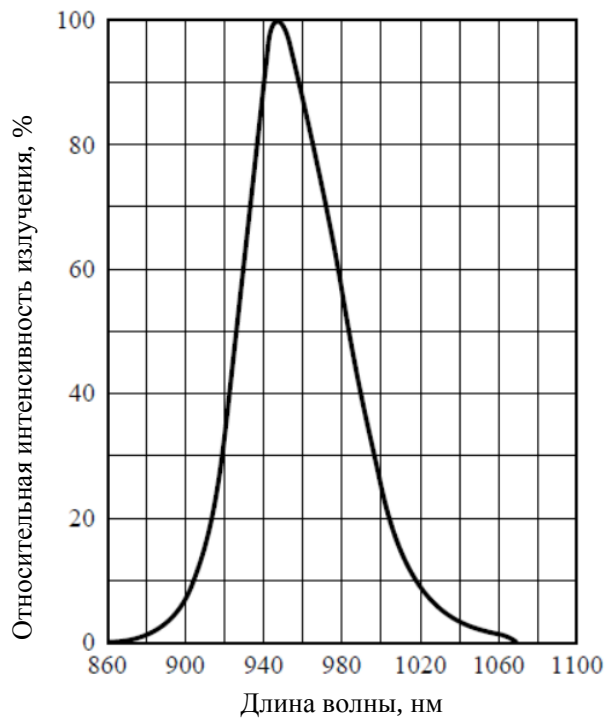
Рис. 2.6. Спектр излучения реального СИД.
