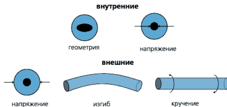
Рис.6.9. Причины возникновения поляризационно-модовой дисперсии
