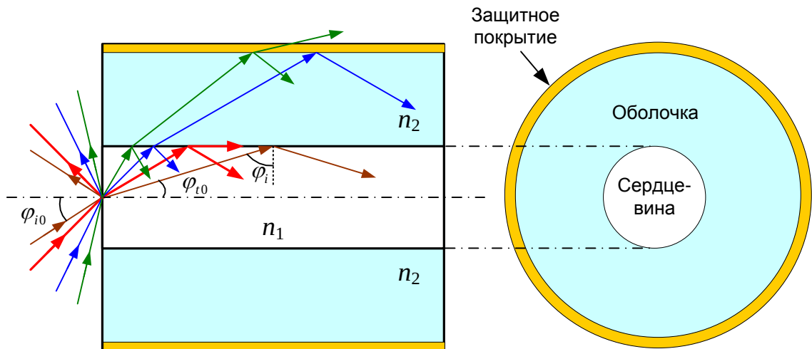
Рис. 6.2. Моды в ступенчатом ОВ
