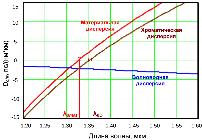
Рис. 6.7. Хроматическая дисперсия в стандартном ОВ.
