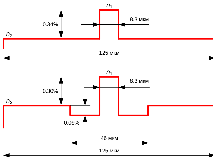
Рис. 6.11. Профили показателей преломления стандартных одномодовых ОВ
