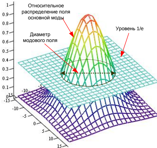
Рис. 6.6. Определение диаметра модового поля ступенчатого ОВ
