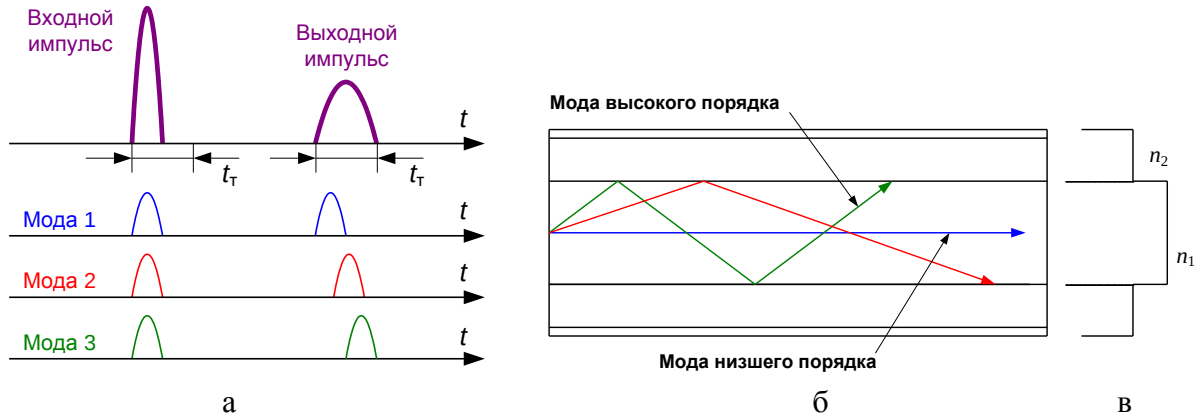
Рис.6.3. Возникновение межмодовой дисперсии в волокне со ступенчатым профилем показателя преломления, формы входного и выходного оптических импульсов (а). Траектории меридиональных лучей в ОВ со ступенчатым профилем показателя преломления (б). Ступенчатый профиль показателя преломления (в).
