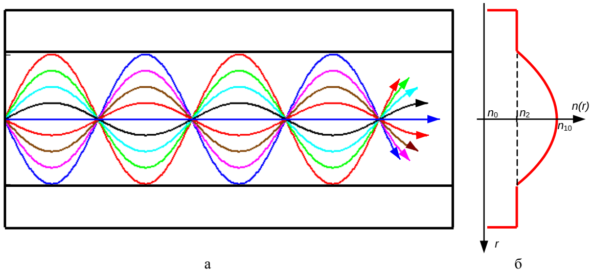
Рис. 6.5. Траектории меридиональных лучей (а) в ОВ с усеченным степенным профилем показателя преломления (б).
