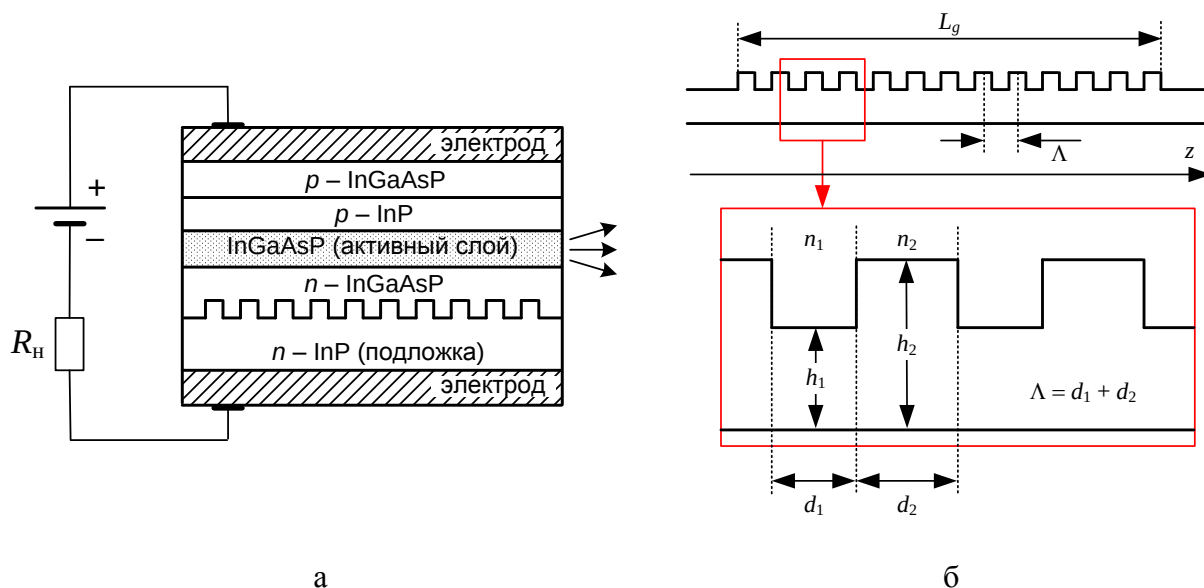
Рис. 2.17. Конструкция и схема включения ЛД DFB (а) и конструкция решетки Брэгга (б)
