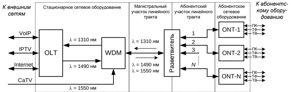
Рис. 1.8. Упрощенная схема одного сегмента PON.
