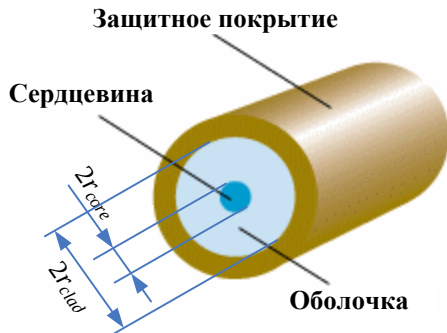
Рис. 6.1. Структура ОВ
