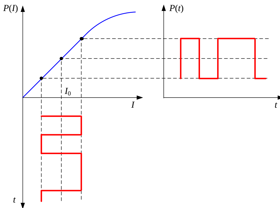
Рис. 3.5. Внутренняя модуляция излучения СИД
