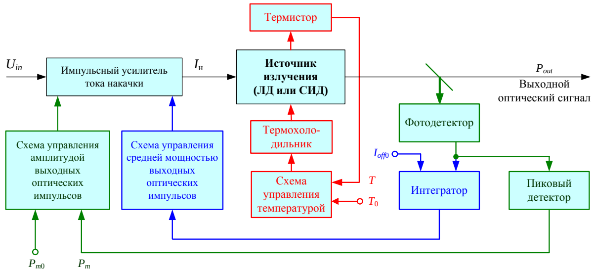
Рис. 3.6. Структурная схема ПОМ с внутренней модуляцией.
