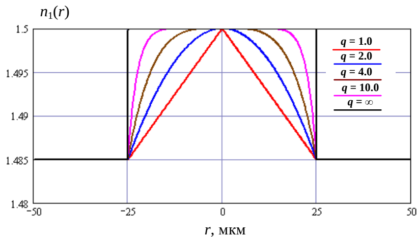
Рис. 6.4. Усеченные степенные профили показателя преломления.
