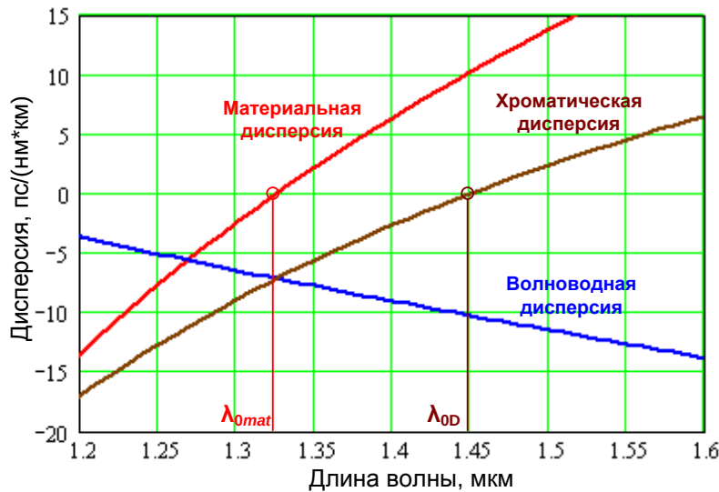
Рис.6.8. Смещение длины волны нулевой хроматической дисперсии путем изменения волноводной дисперсии.
