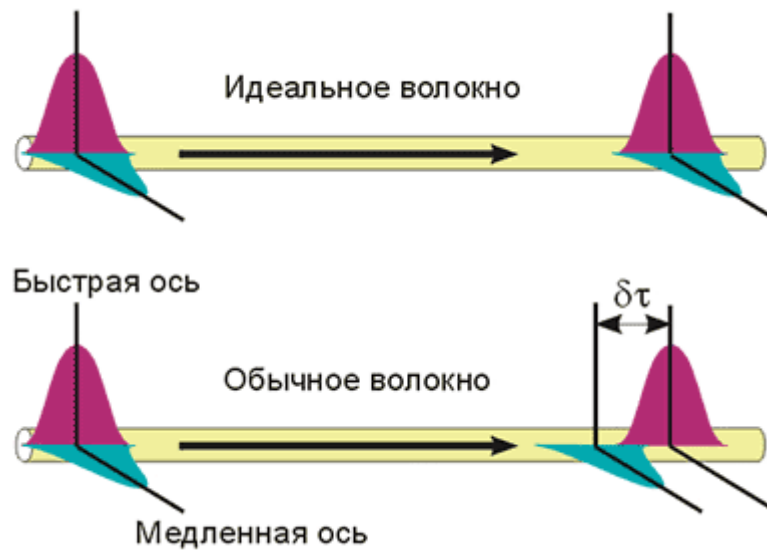
Рис. 6.10. Возникновение поляризационно-модовой дисперсии
