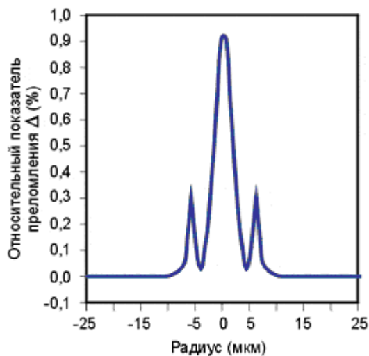
Рис. 6.12. Профили показателей преломления ОВ со смещенной дисперсией
