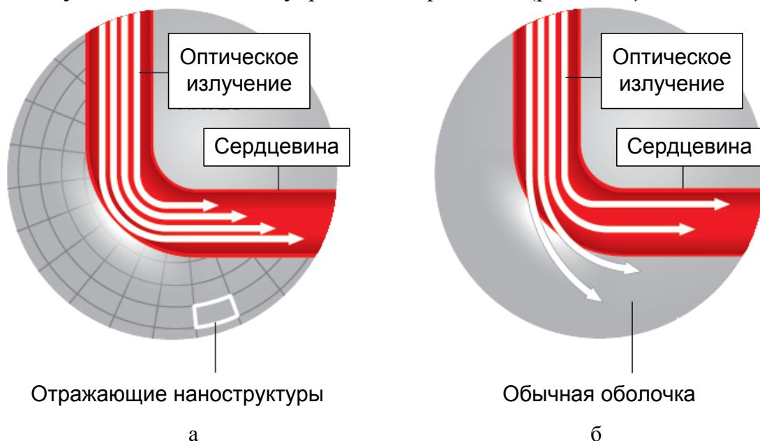
Рис. 6.15. Удержание света в сердцевине ОВ стандарта G.657
