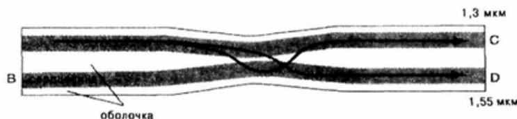
Рис. 5.7. Процесс разделения длин волн при помощи разветвителя на основе одномодового волокна
