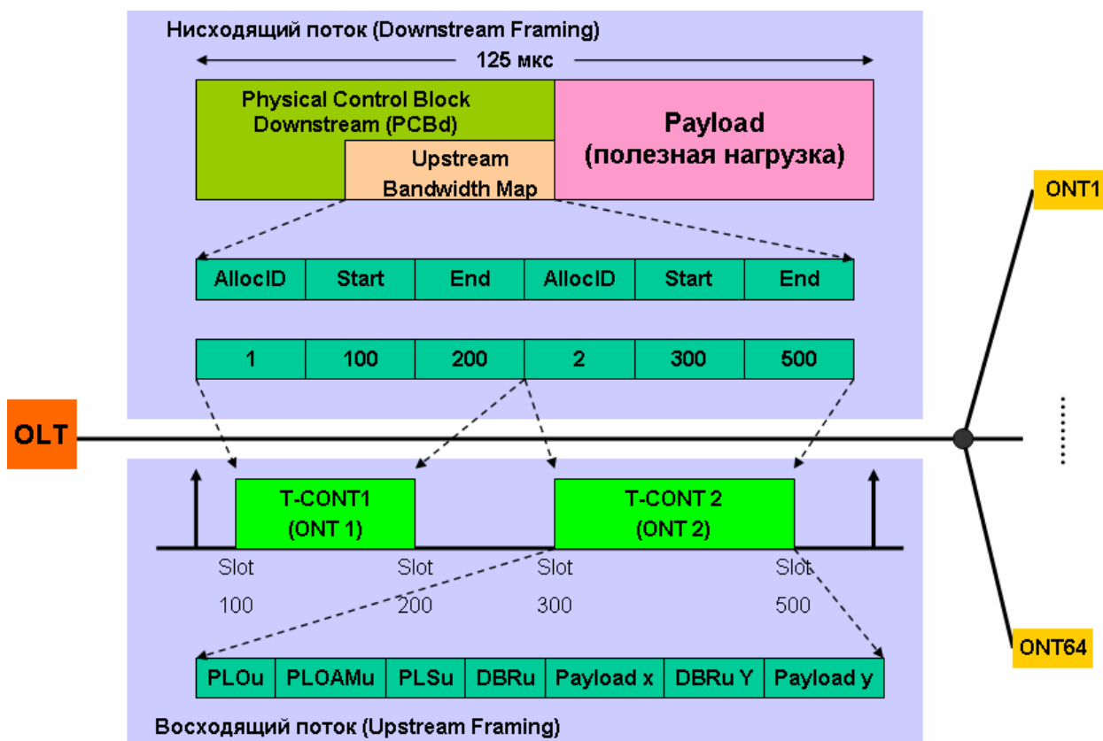
Рис. 6.7. Распределение полосы пропускания в восходящем потоке GPON (пример T-CONT1 и T-CONT2).
