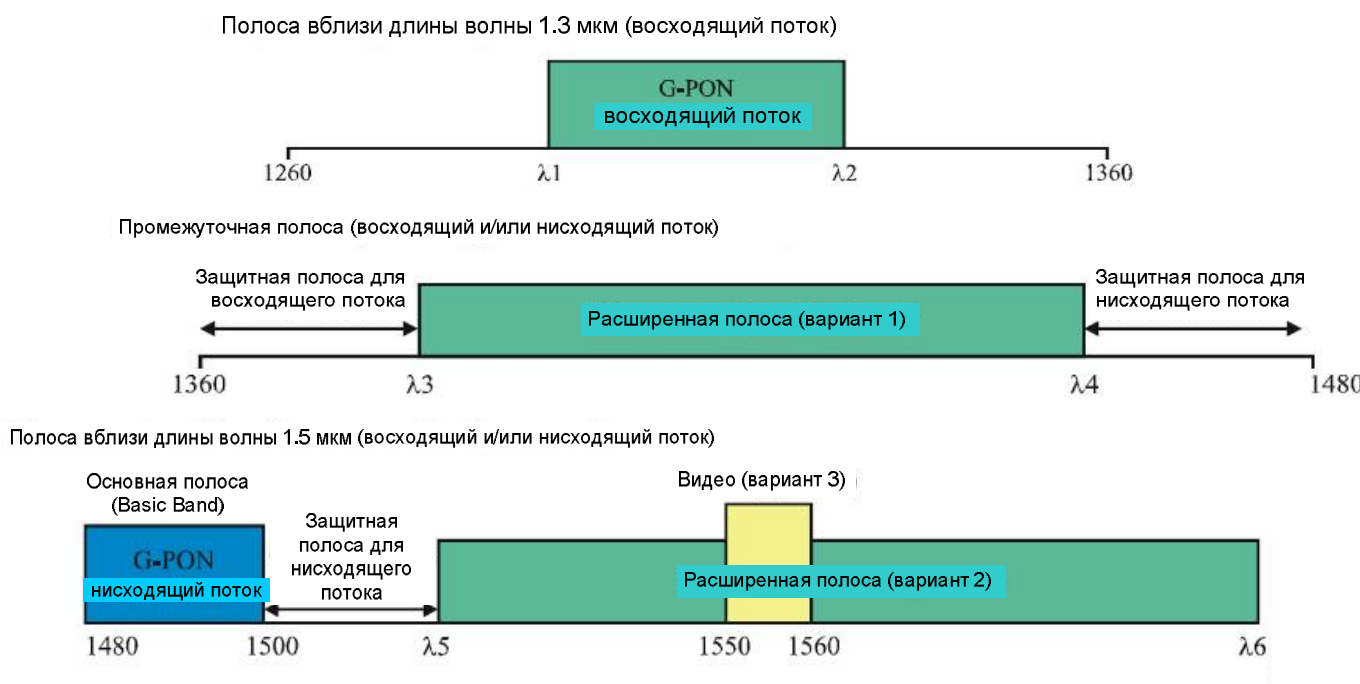
Рис. 2.13. Распределение длин волн в сетях GPON.
