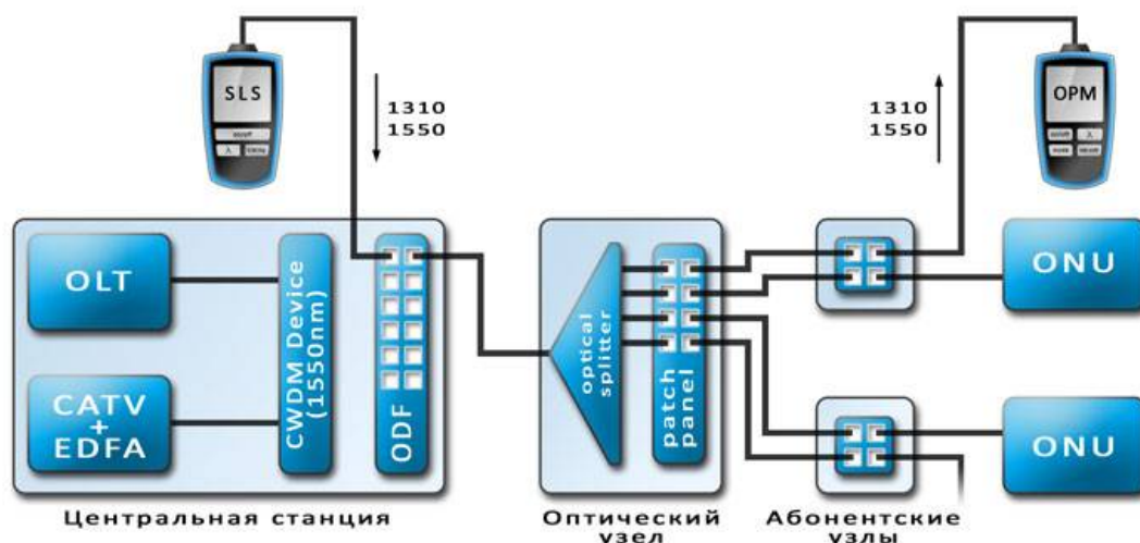
Рис. 7.5. Подключение SLS и OPM.
