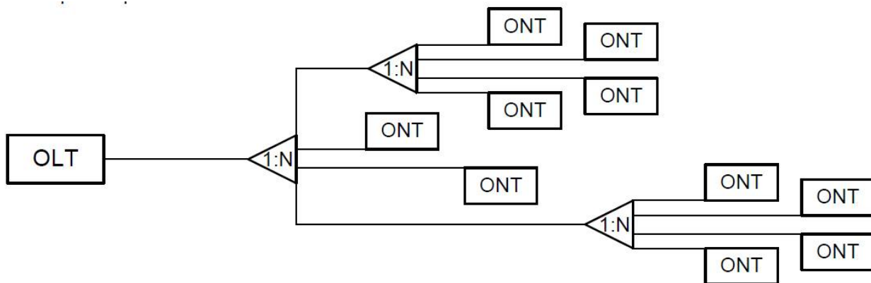
Рис. 2.7. Топология «дерево».
