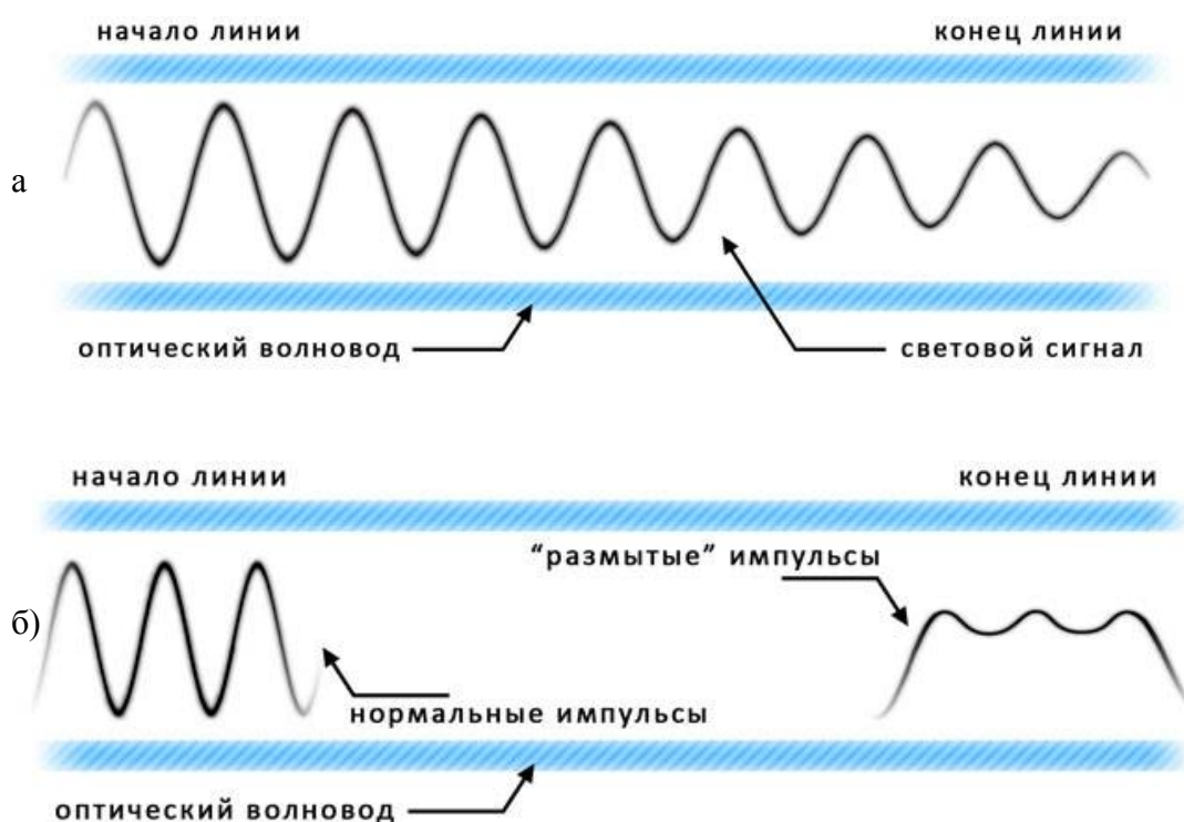
Рис. 7.1. Влияние затухания (а) и дисперсии (б) на форму сигнала.
