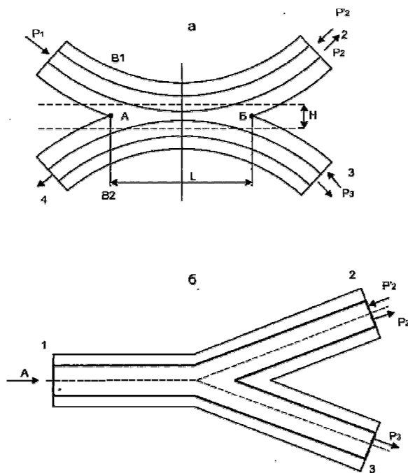
Рис. 5.1. Направленный ответвитель Х-типа (а) и разветвитель Y-типа (б)
