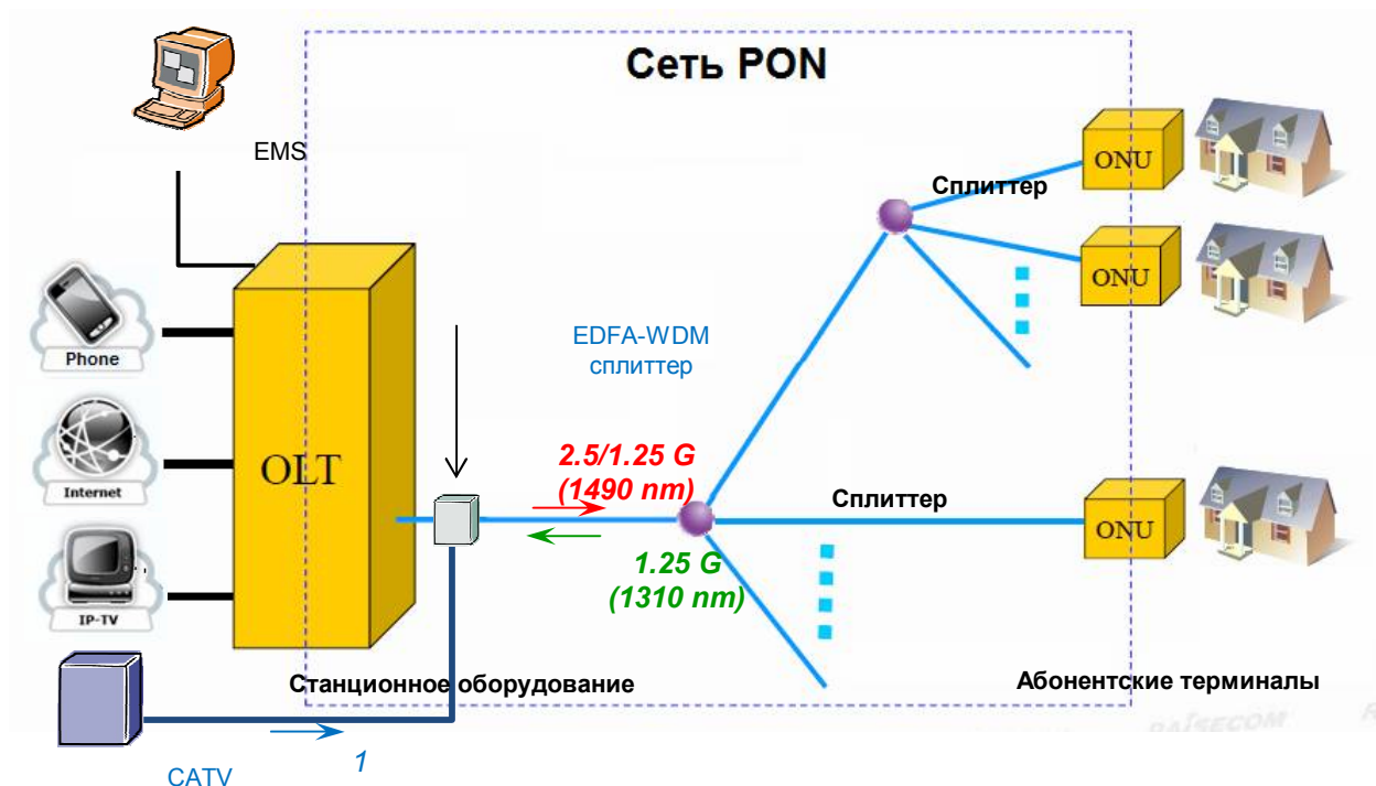
Рис. 2.1. Структура сети PON.
