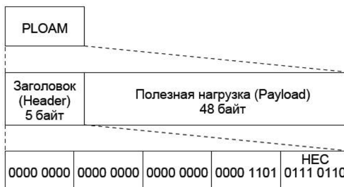
Рис. 2.10. Структура PLOAM ячейки WDM-PON.
