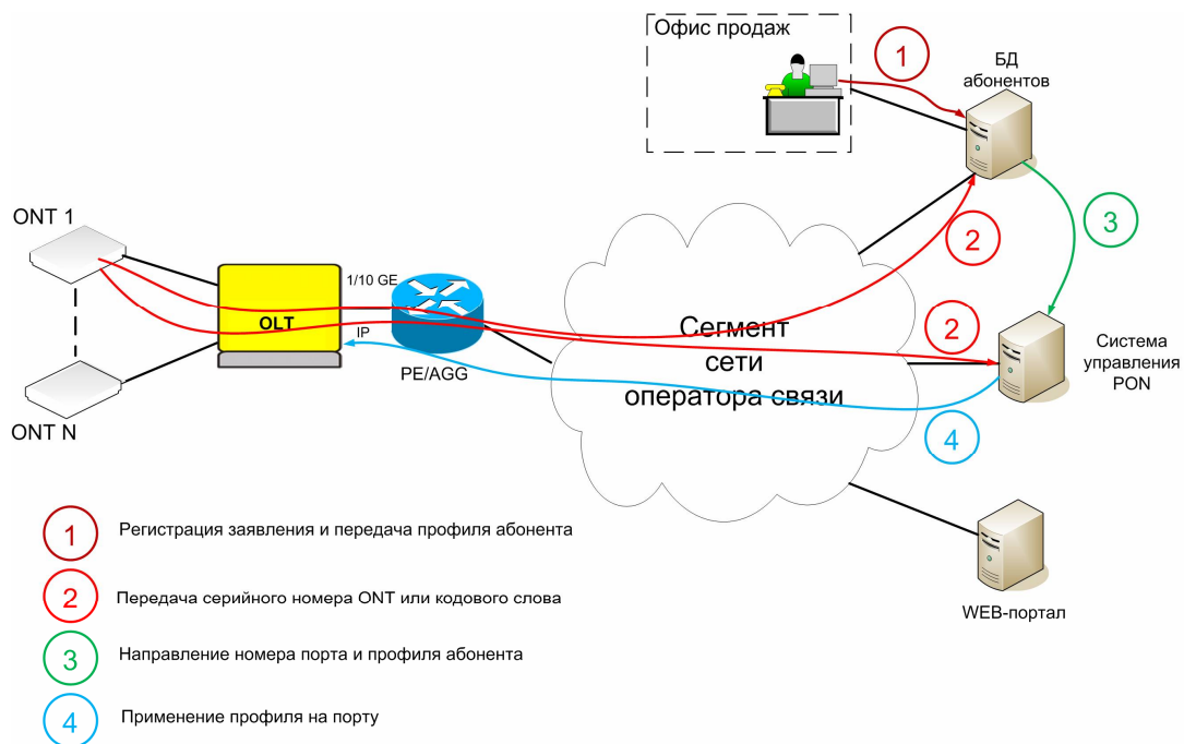
Рис. 6.5. Подключение абонента
