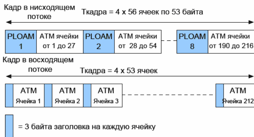
Рис. 2.9. Нисходящий и восходящий кадры WDM-PON для скорости 622 Мбит/с.
