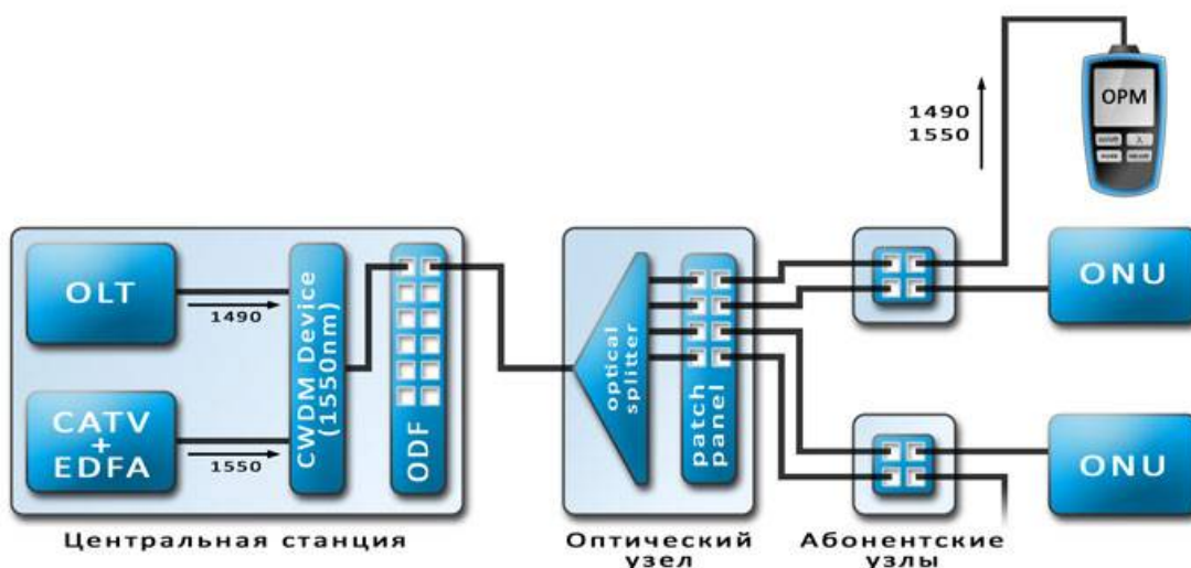
Рис. 7.6. Подключение OPM при использовании передатчика OLT вместо SLS.
