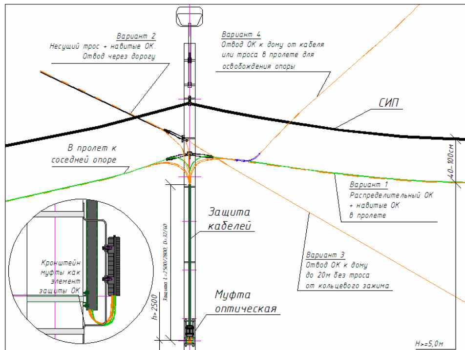
Рис. 5.15. Прокладка ВОК по опорам силовой/осветительной сети.
