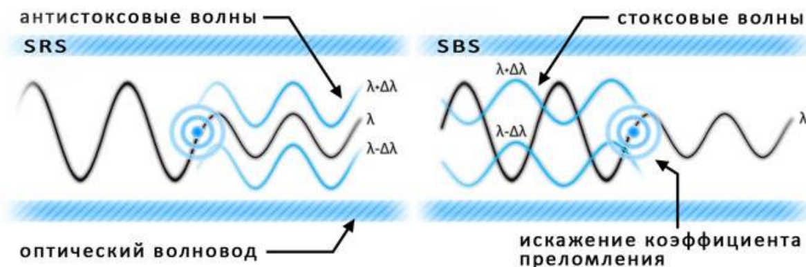
Рис. 7.2. Влияние вынужденного неупругого рассеяния.
