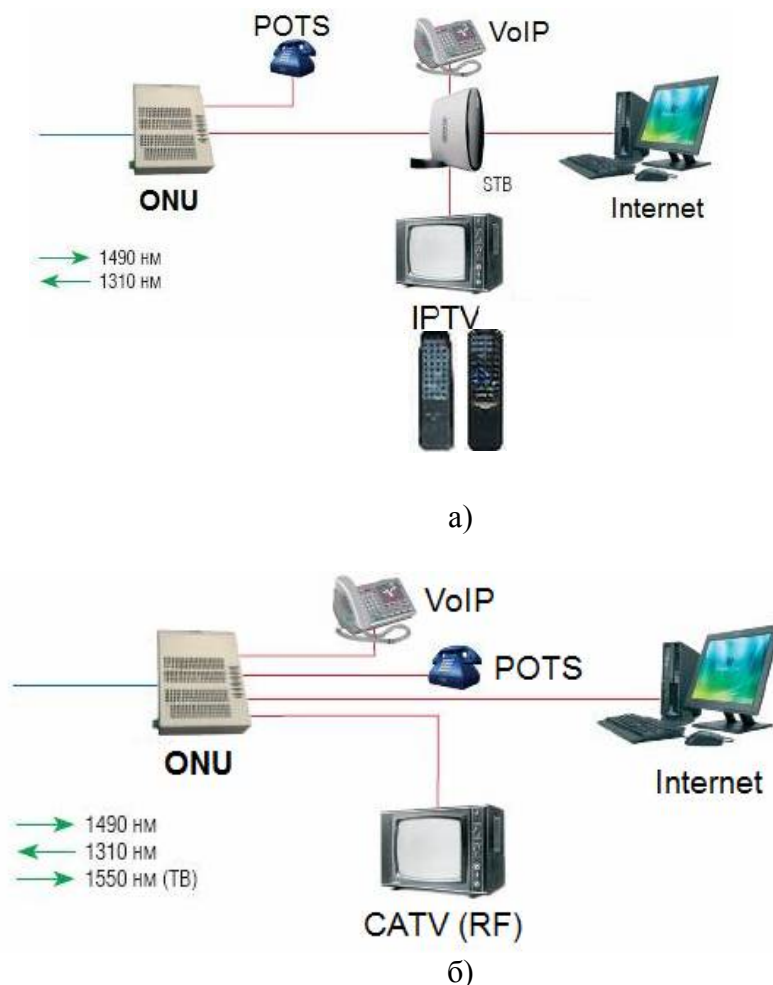
Рис.6.2 Предоставление комплекса мультимедийных услуг: а) по IP (телевизионный сигнал IPTV преобразуется в аналоговый с помощью TV-приставки STB); б) с использованием оптической поднесущей 1550 нм (TV-приёмник подключён непосредственно к ONT через разъём RF)
