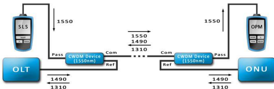
Рис. 7.11. Пример проведения измерений в PON без разрыва связи.
