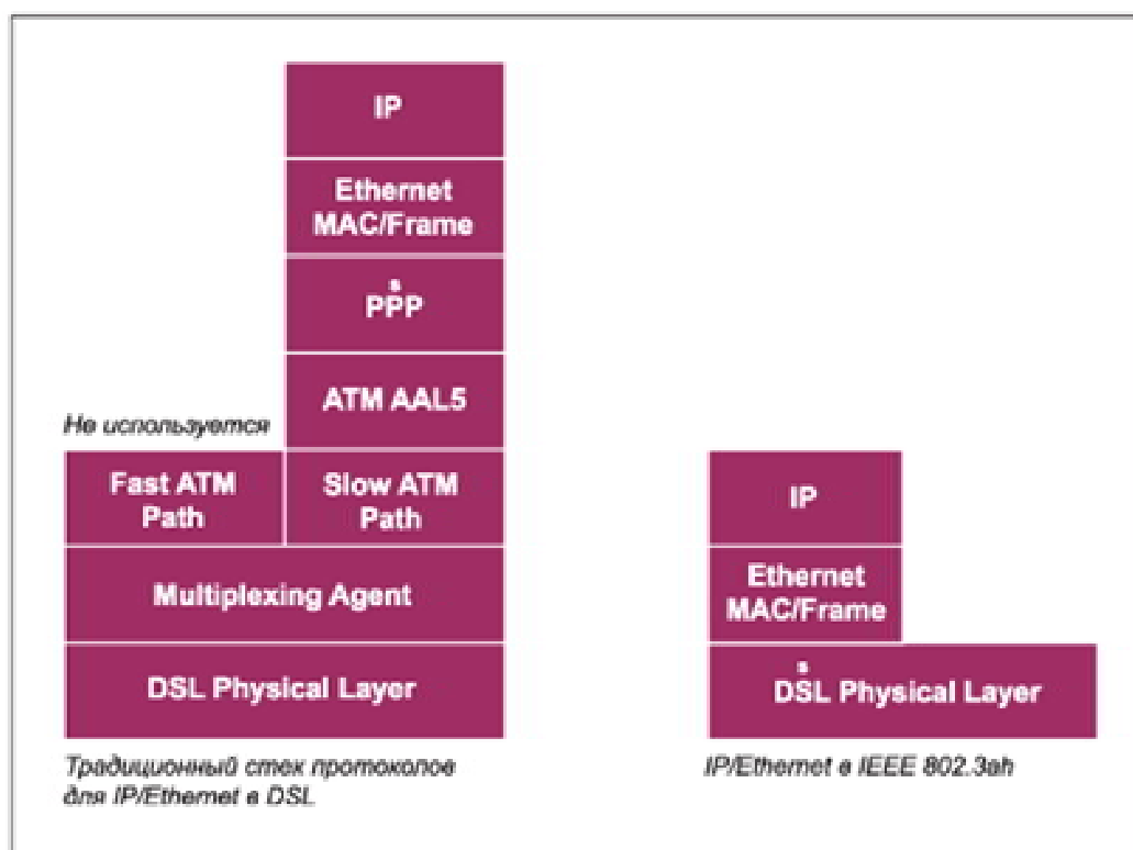
Рис. 1.8 Стек протоколов EFM и традиционного DSL.
