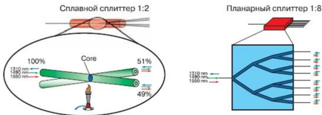
Рис. 5.3. Основные технологии изготовления сплиттеров.
