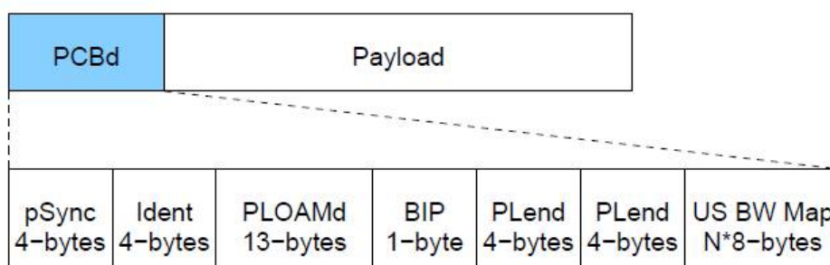
Рис. 2.15. Обзор заголовка PCBd.
