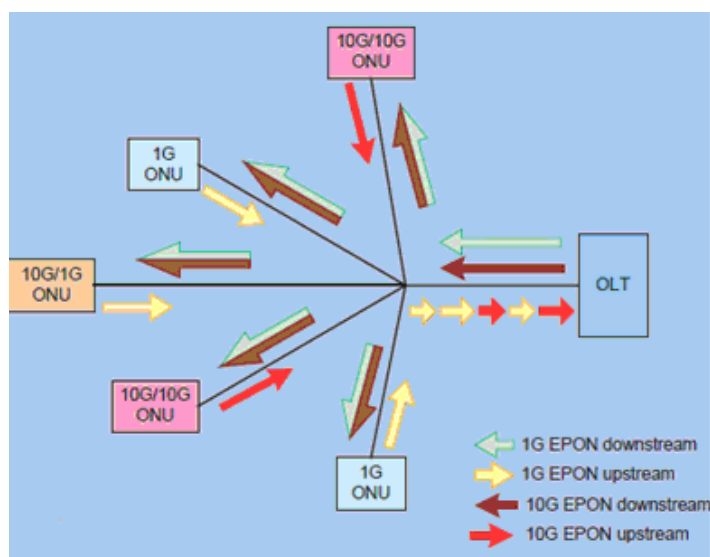
Рис. 3.6. Пример использования 1G-EPON и 10G-EPON в одной сети.
