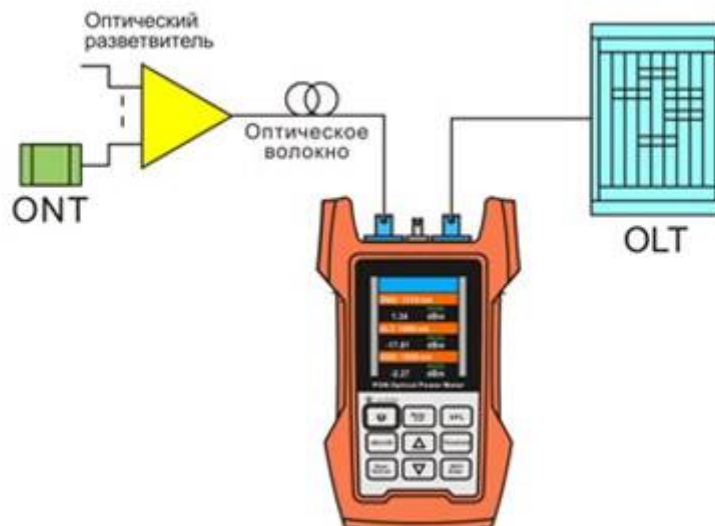
Рис. 7.4. Использование PON-тестера (измерение со стороны OLT на 1490 нм и 1550 нм).
