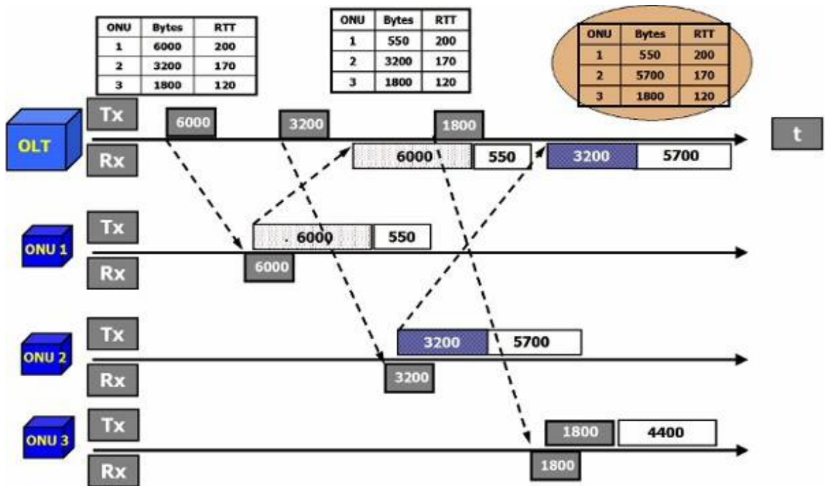
Рис. 6.9. Схема работы алгоритма IPACT в EPON.
