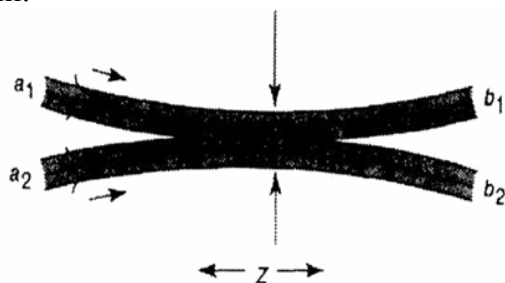
Рис. 5.4. Схематичное изображение сплавного биконического разветвителя
