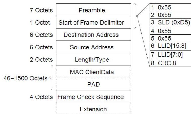
Рис. 3.4. Структура кадра MAC.
