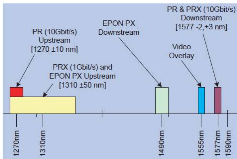
Рис. 3.5. Распределение спектра для сетей стандарта 10 Гбит/с EPON (10G-EPON).
