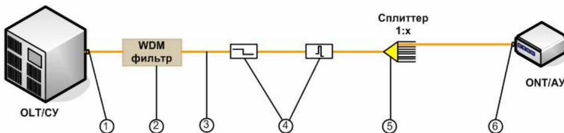
Рис. 7.3. Основные источники потерь в сетях PON.
