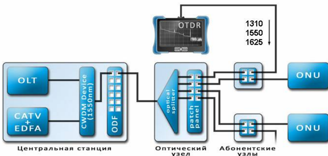
Рис. 7.8. Подключение рефлектометра (OTDR).
