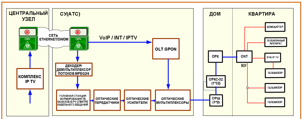
Рис. 6.11. Пример типовой схемы предоставления услуги КТВ
