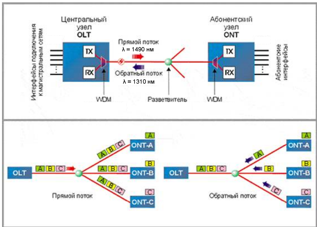
Рис. 2.2. Принцип действия общий вид организации PON.
