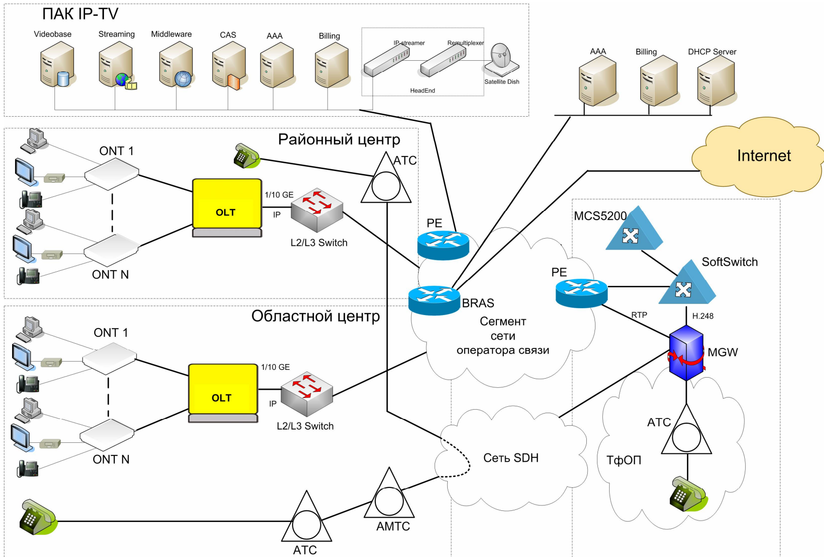
Рис. 6.6. Пример схемы предоставления услуг в сетях PON.
