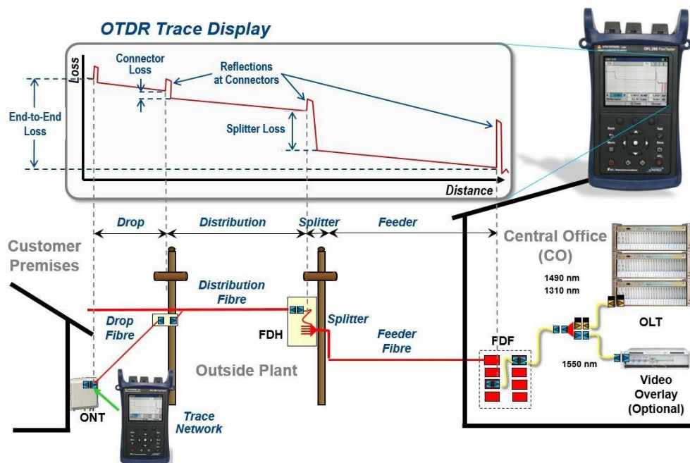
Рис. 7.9. Пример рефлектограммы, снятой со стороны абонента (ONT/ONU).
