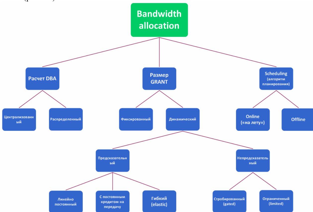
Рис. 6.8. Блок-диаграмма критериев распределения полосы пропускания в сетях EPON.
