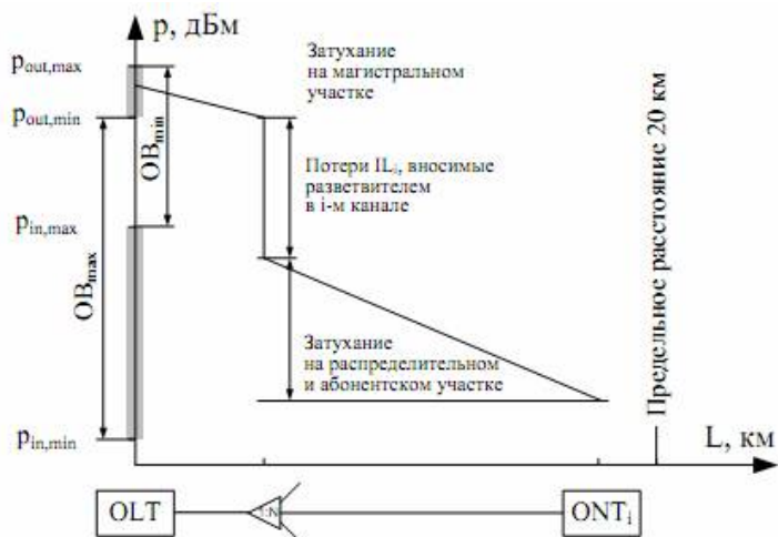
Рисунок 5.16 – Ослабление мощности сигнала.
