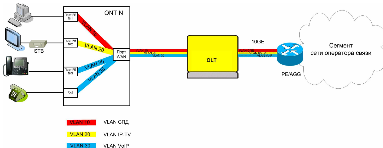
Рис. 6.4. Назначение VLAN.
