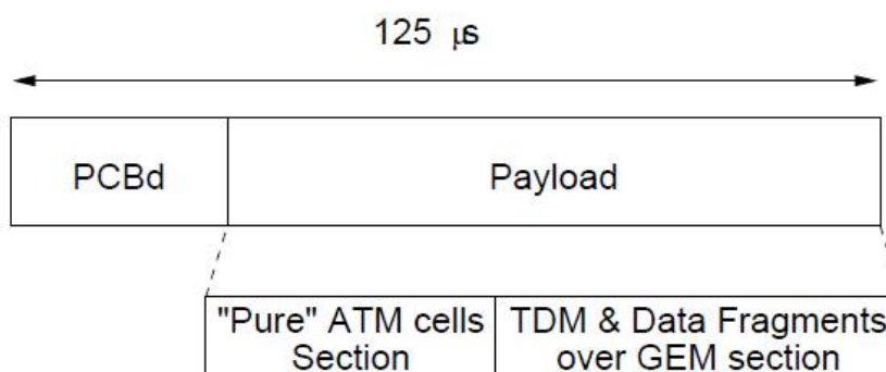
Рис. 2.14. Кадр GPON в нисходящем направлении.
