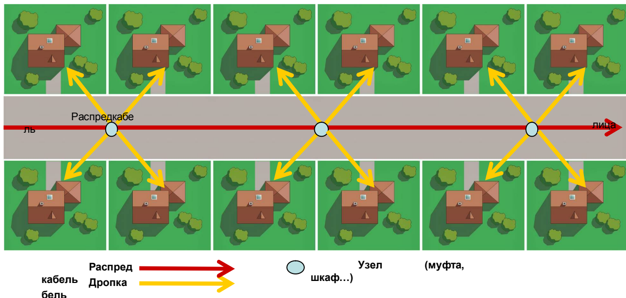
Рис. 5.11. Пример организации ОСД по технологии PON в малоэтажном секторе.
