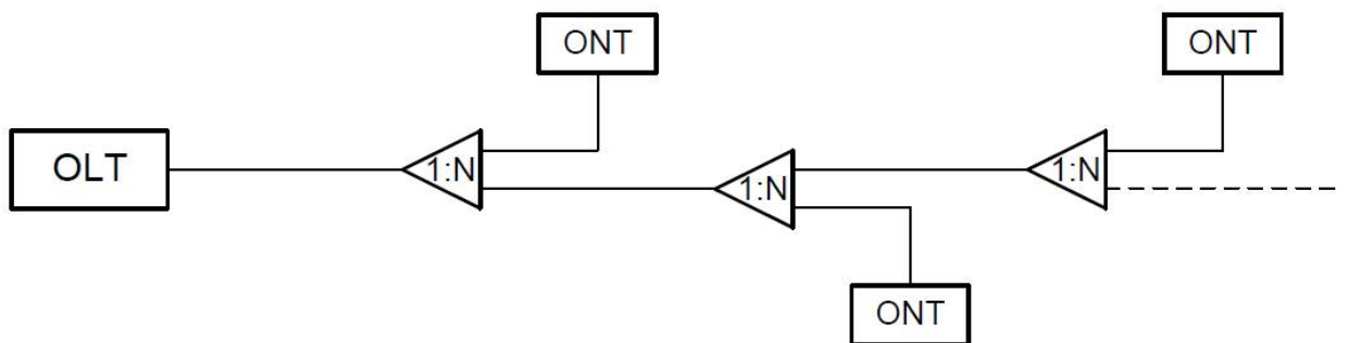
Рис. 2.6. Топология «шина» с использованием неравномерных разветвителей.
