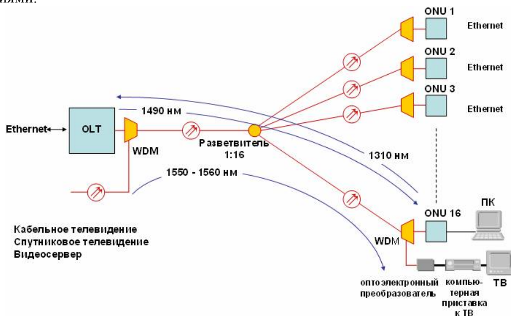
Рис. 3.2. Сеть EPON, предоставляющая услуги аналогового (AM-VSB) или цифрового (DVB-C) телевидения.
