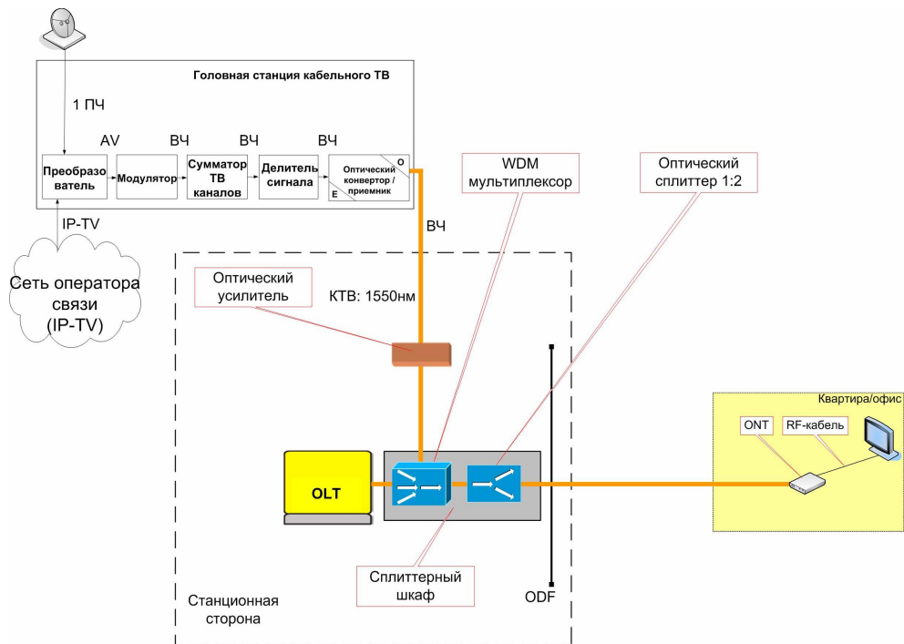
Рис. 6.10 Схема предоставления услуг КТВ в сетях PON.
