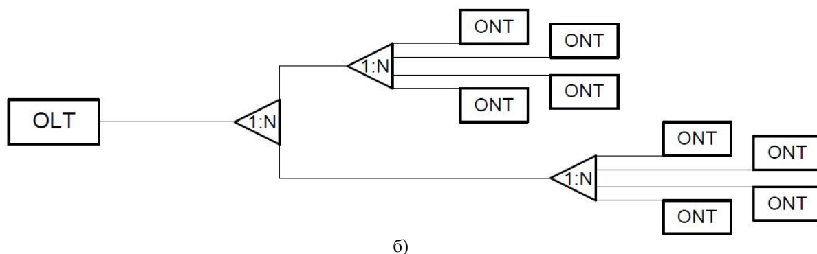
а) одноуровневая схема включения сплиттеров б) многоуровневая схема включения сплиттеров
