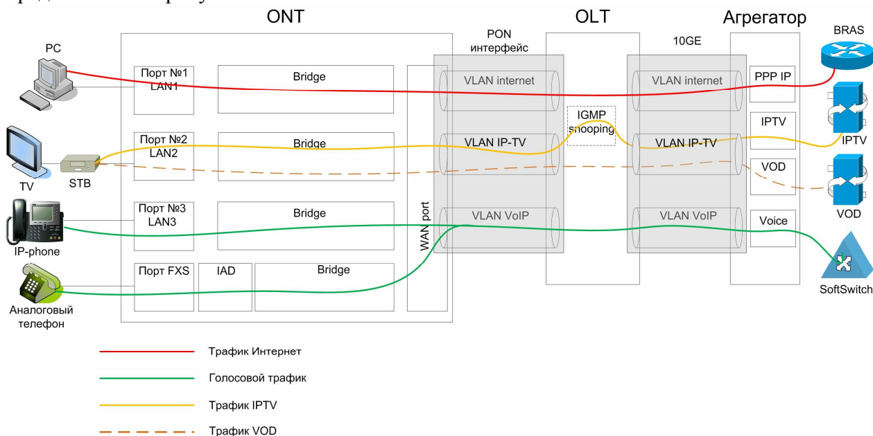
Рис. 6.1. Реализация логической модели предоставления услуг.
