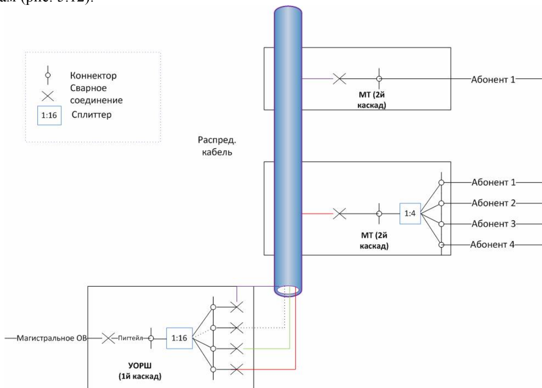
Рис. 5.12. Двухкаскадная схема (1x16 + 1x4) организации связи по технологии PON.
