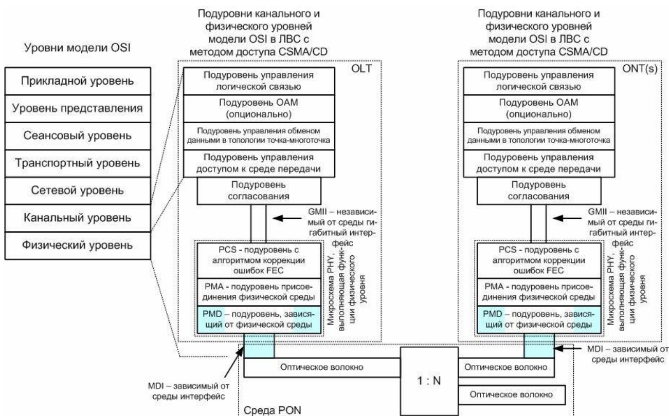
Рис. 3.1. Архитектура сети 1G-EPON.
