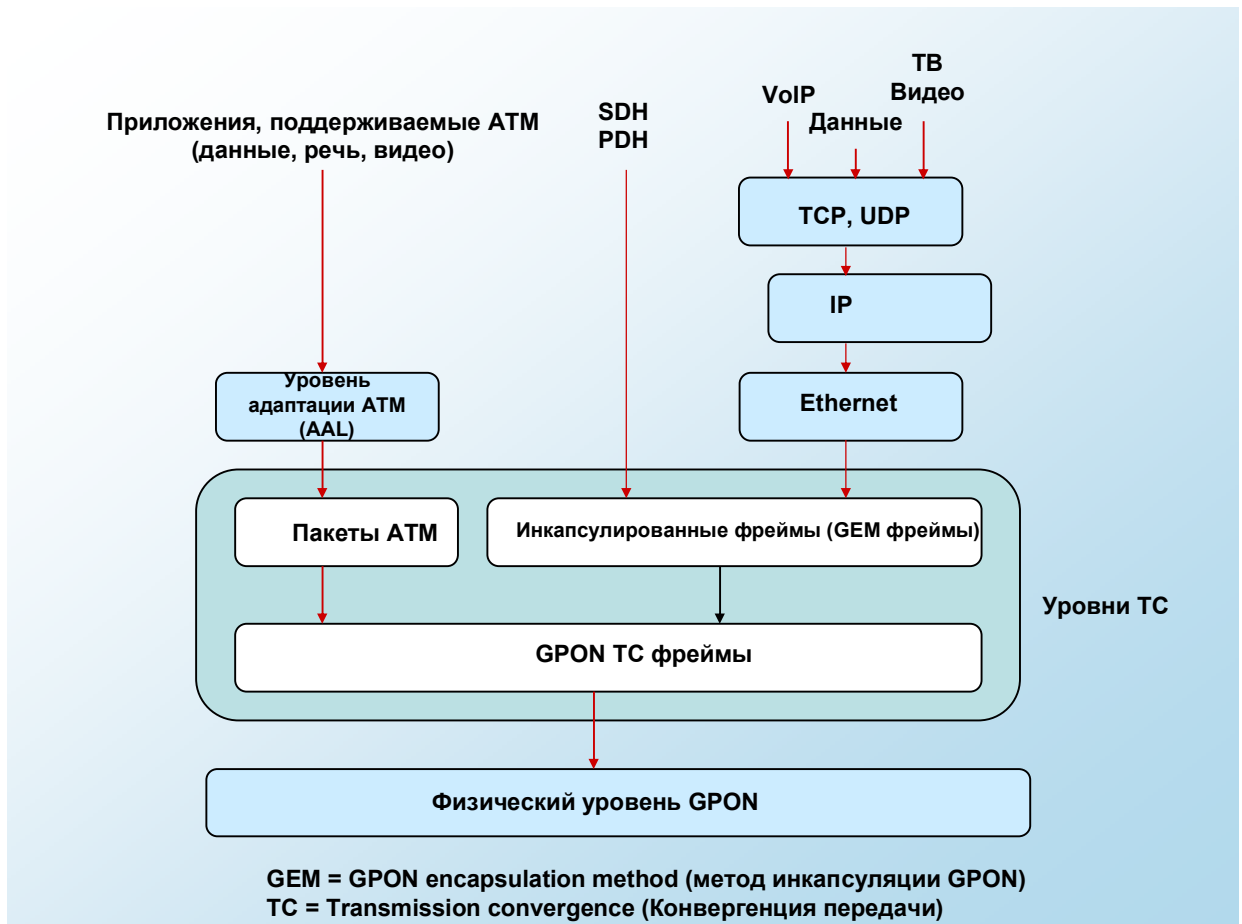
Рис. 2.12. Принципы генерации пакетов GPON.
