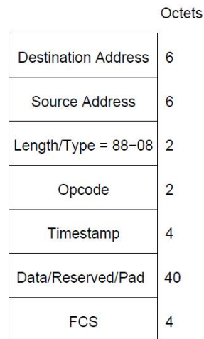
Рис. 3.3. Структура MPCPDU.
