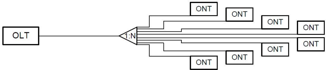
Рис. 2.5. Топология «звезда».
