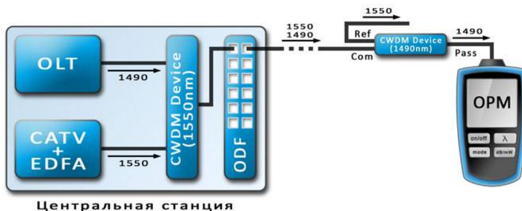
Рис. 7.7. Подключение OPM через CWDM-фильтр.
